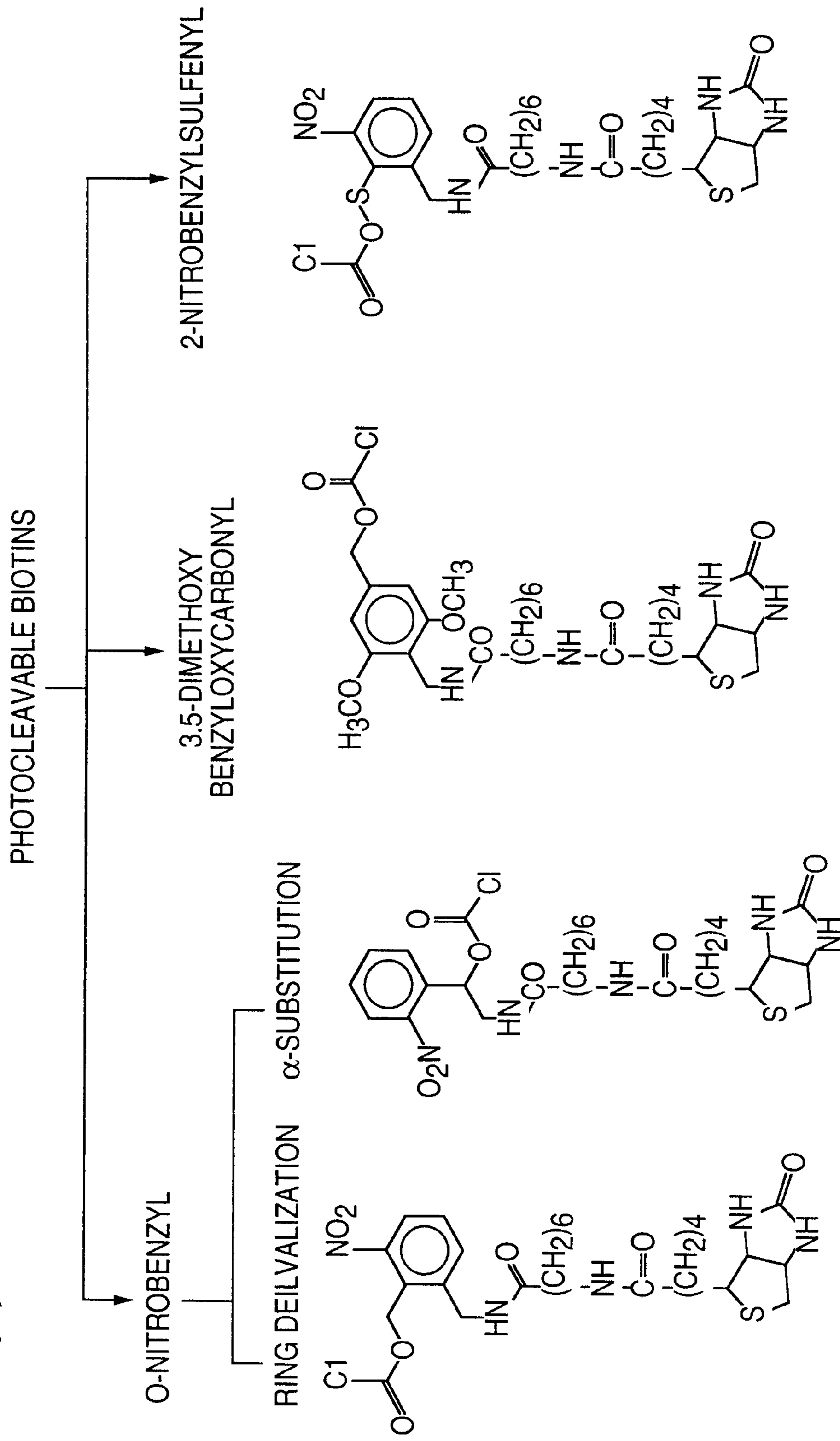
FIG. 8(A)
