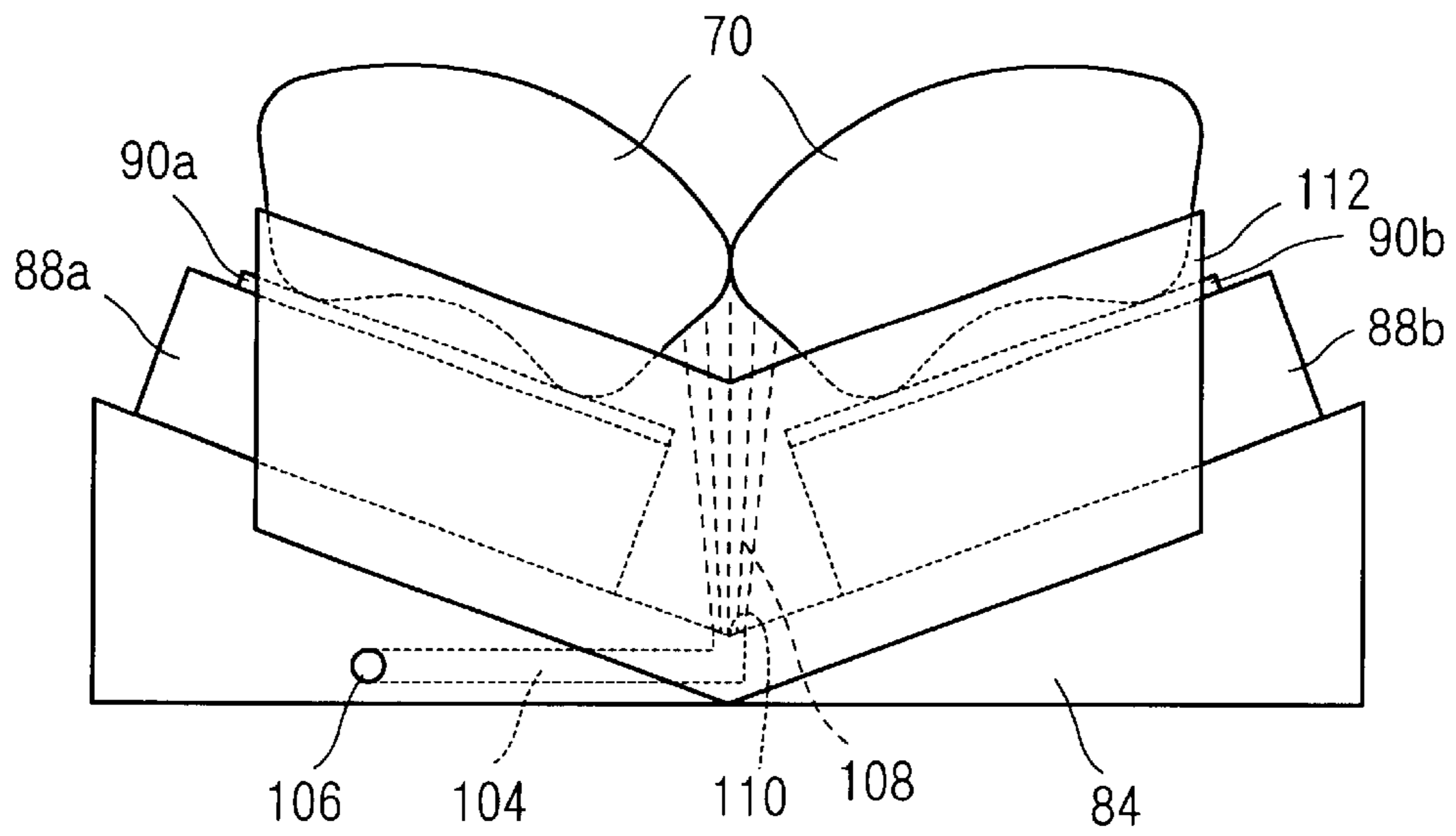
FIG. 11B
