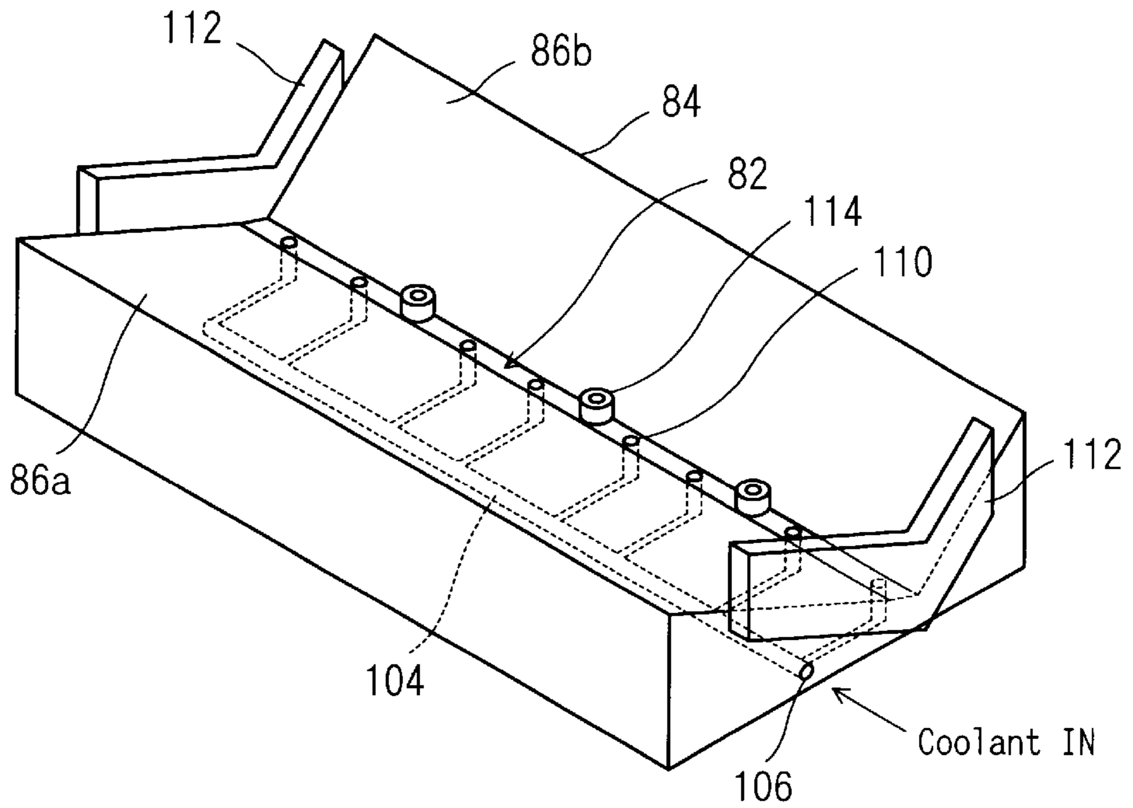
FIG. 11B
