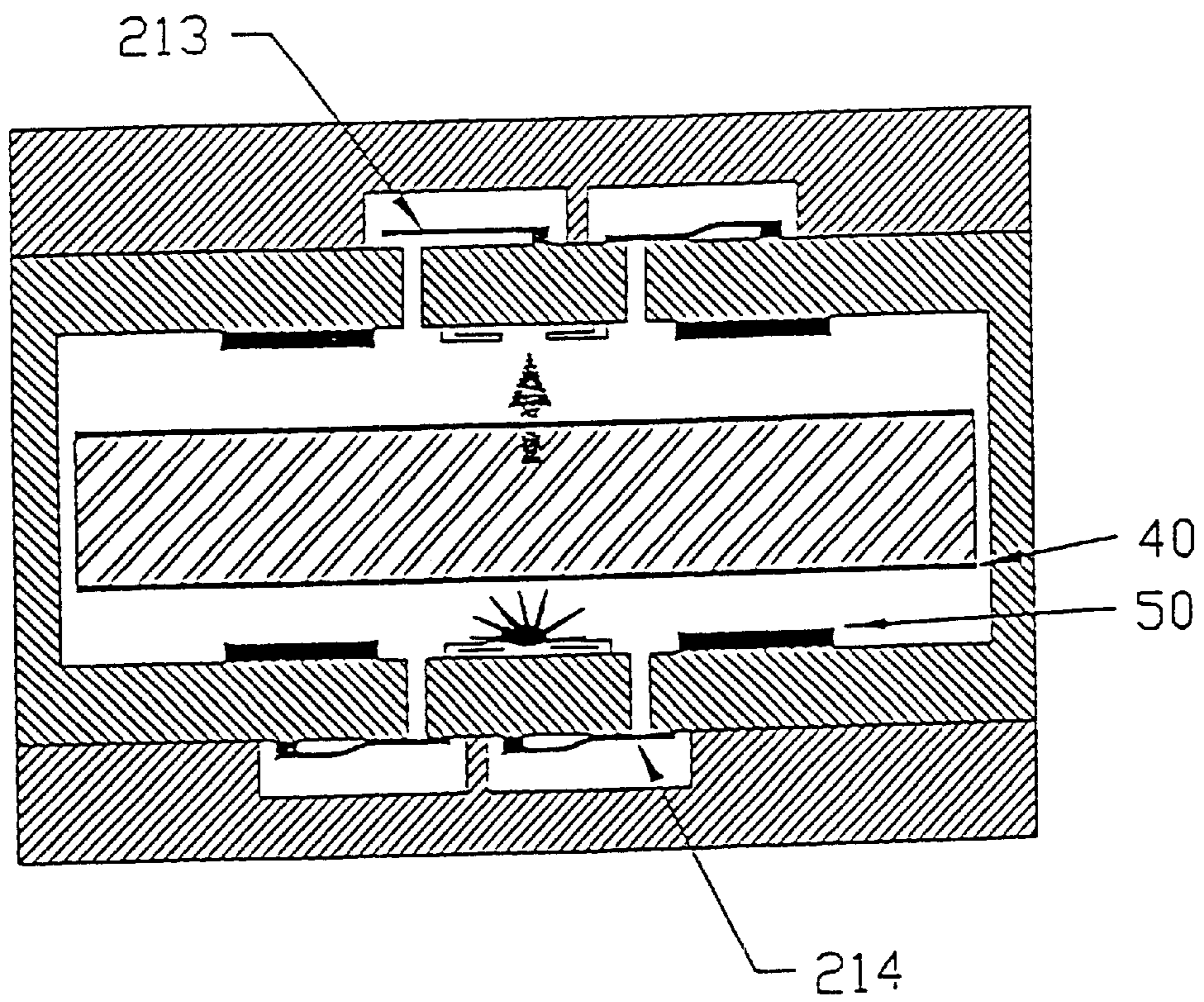
(engine, step 4) FIG. 6d
