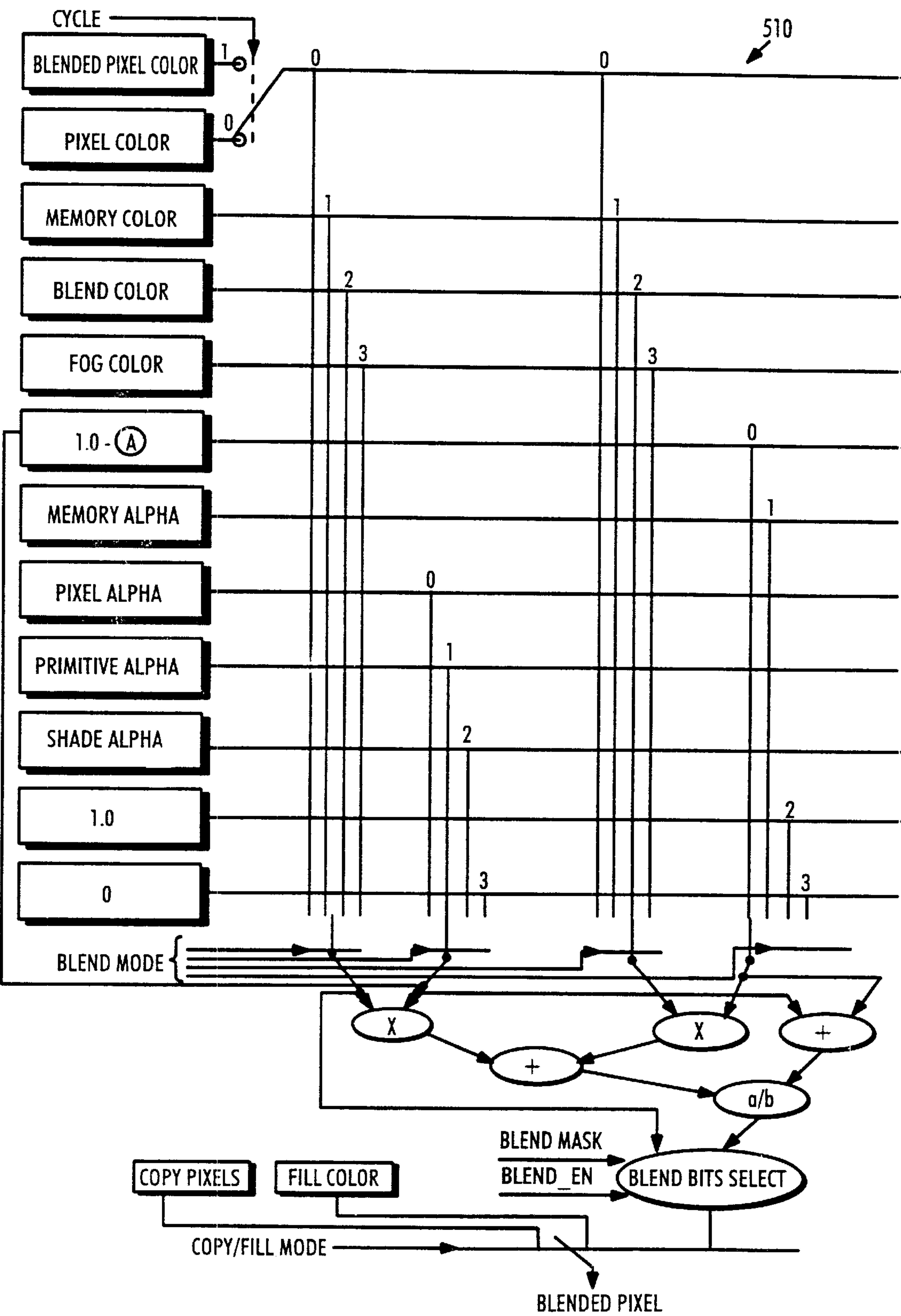
Fig. 31 BLENDER
