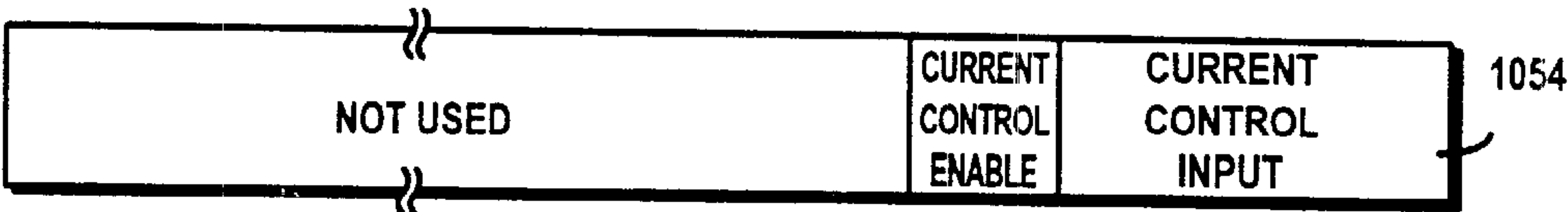
Fig. 37B MI CONFIG REGISTER (R/W)
