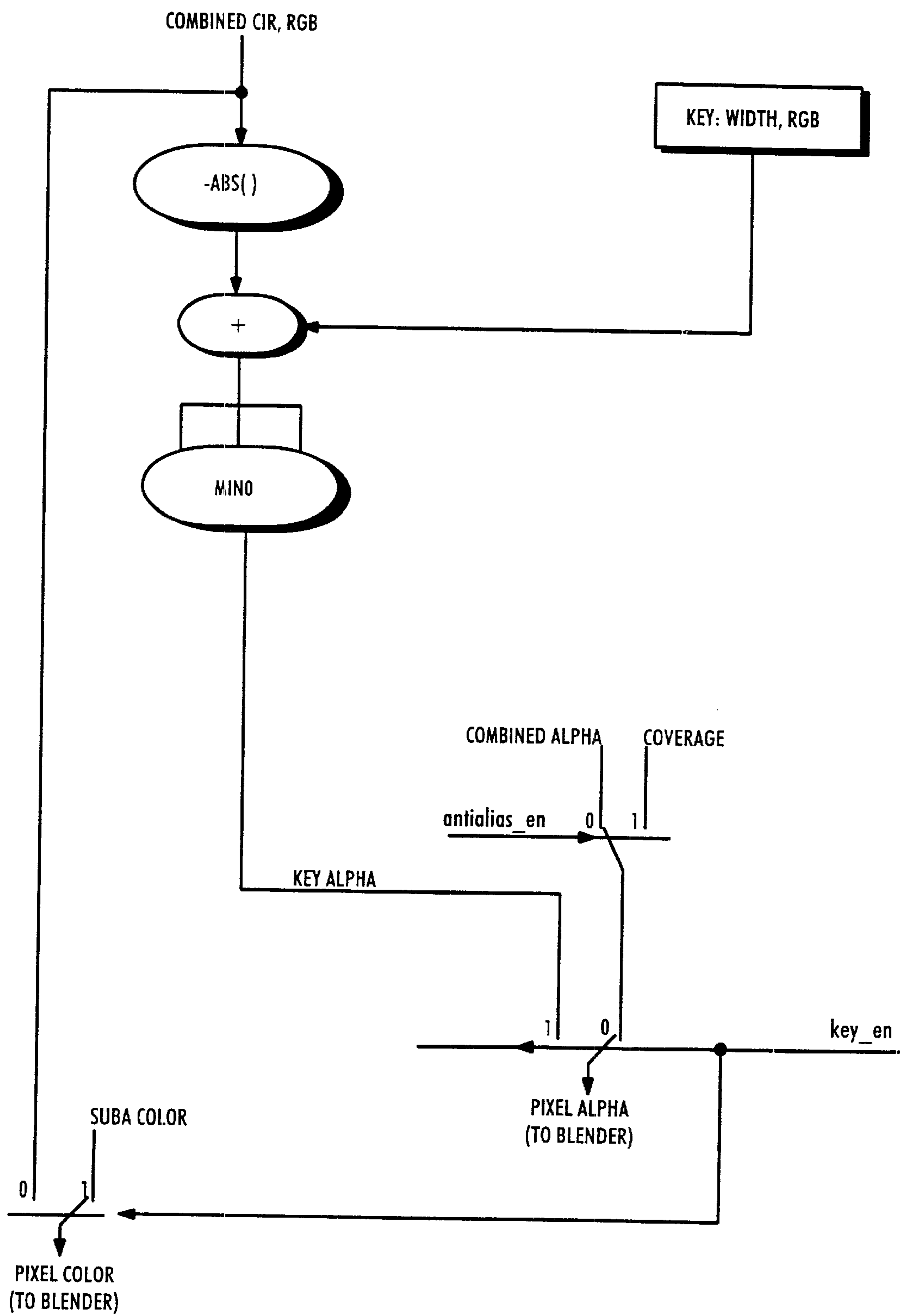
Fig. 29 ALPHA FIXUP
