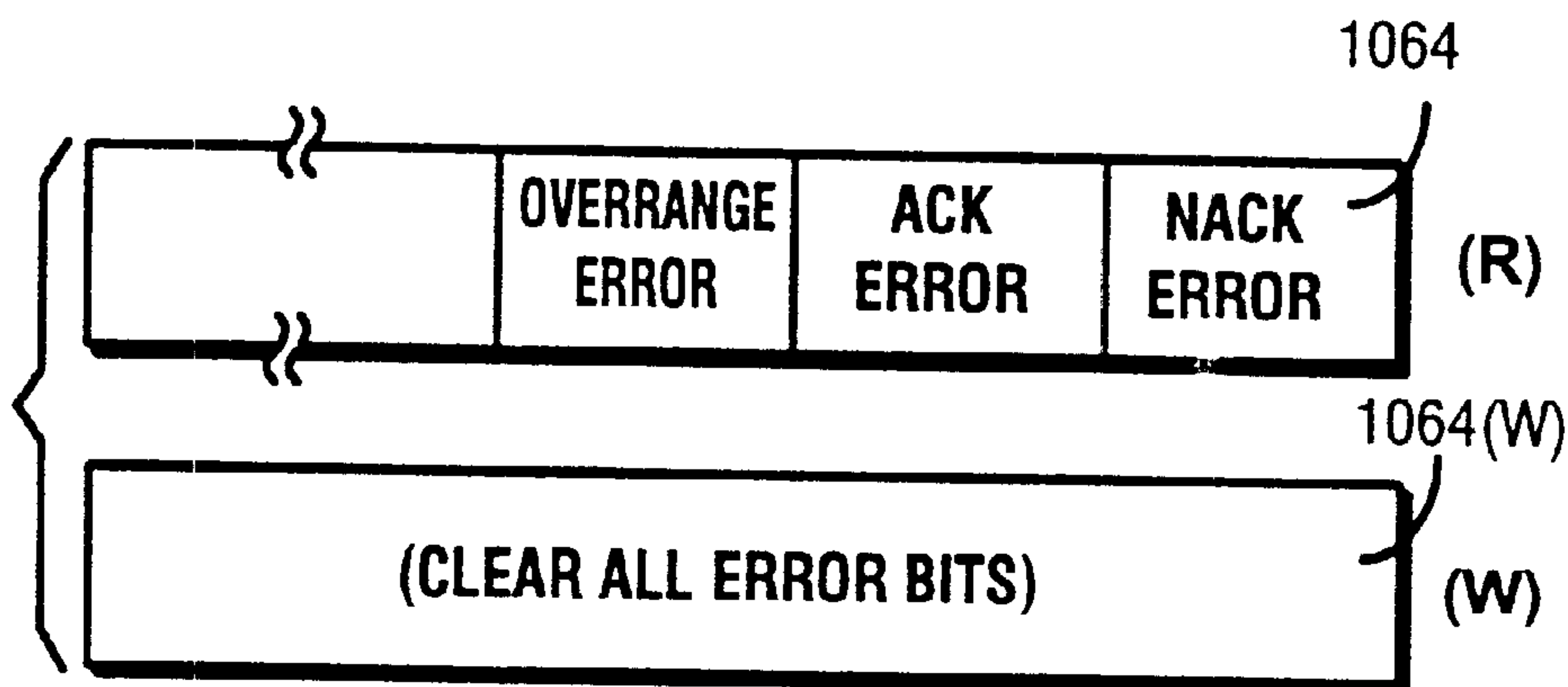
Fig. 37G ERROR REGISTER
