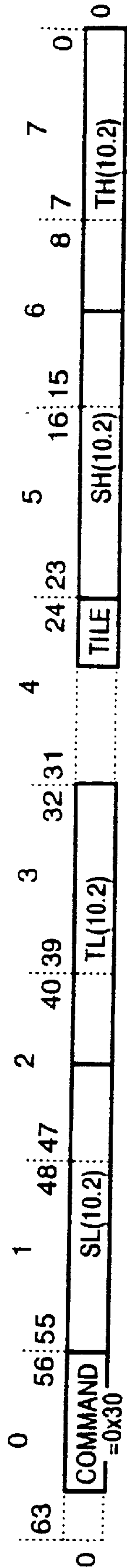
Fig. 62 Load_Tlut
