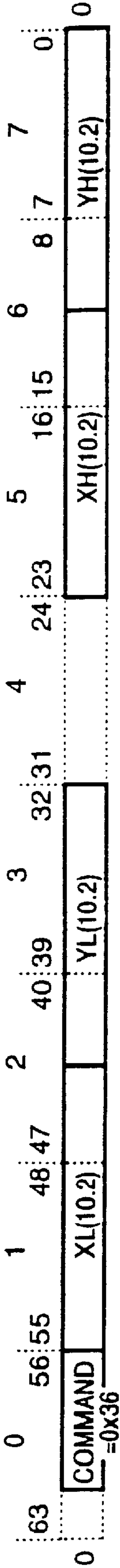
Fig. 77 Fill Rectangle
