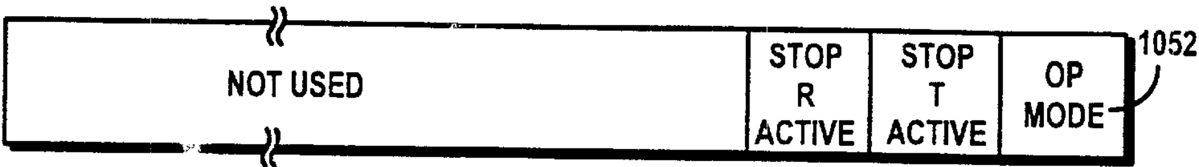
Fig. 37A MI MODE REGISTER(R/W)
