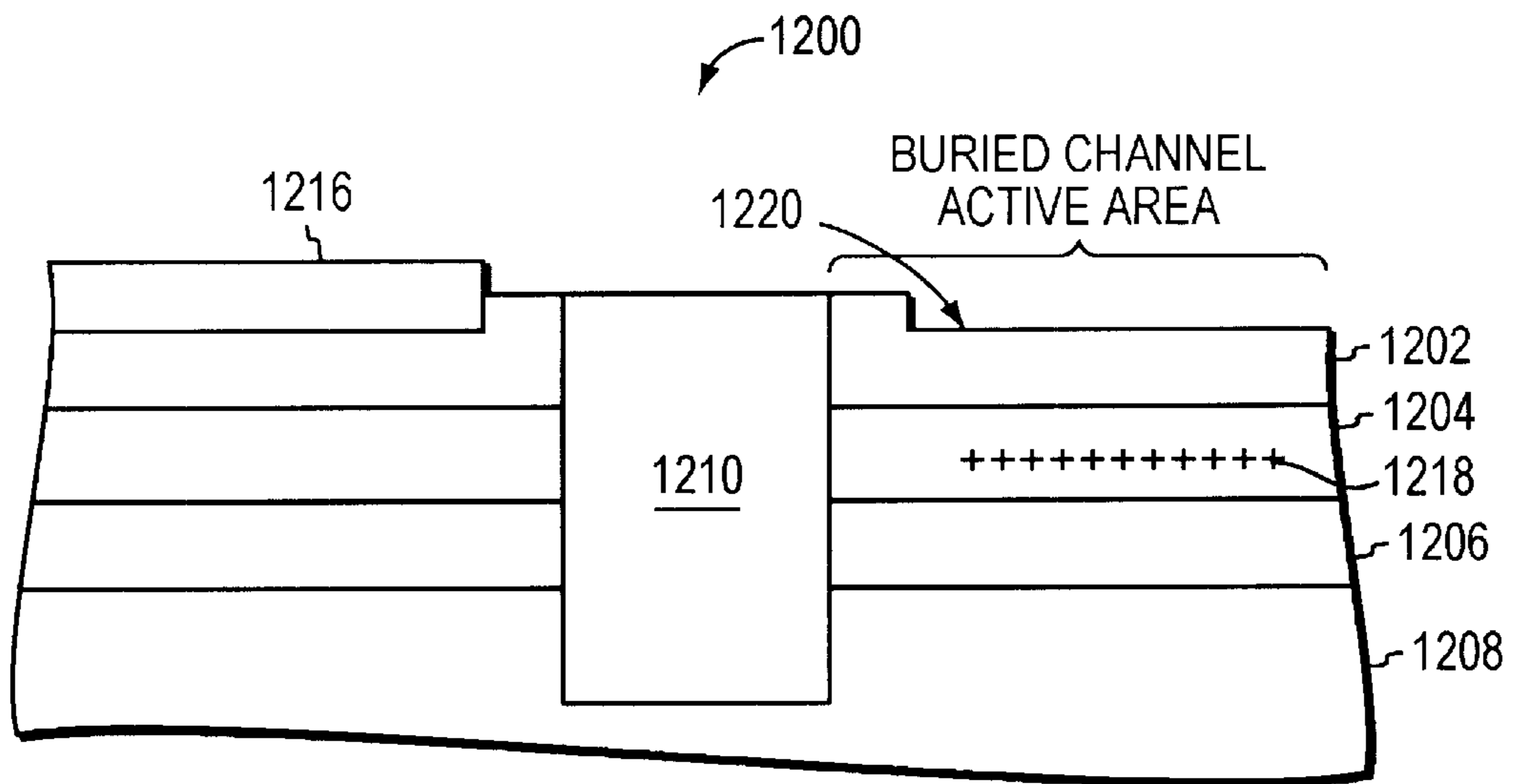
FIG. 12C
