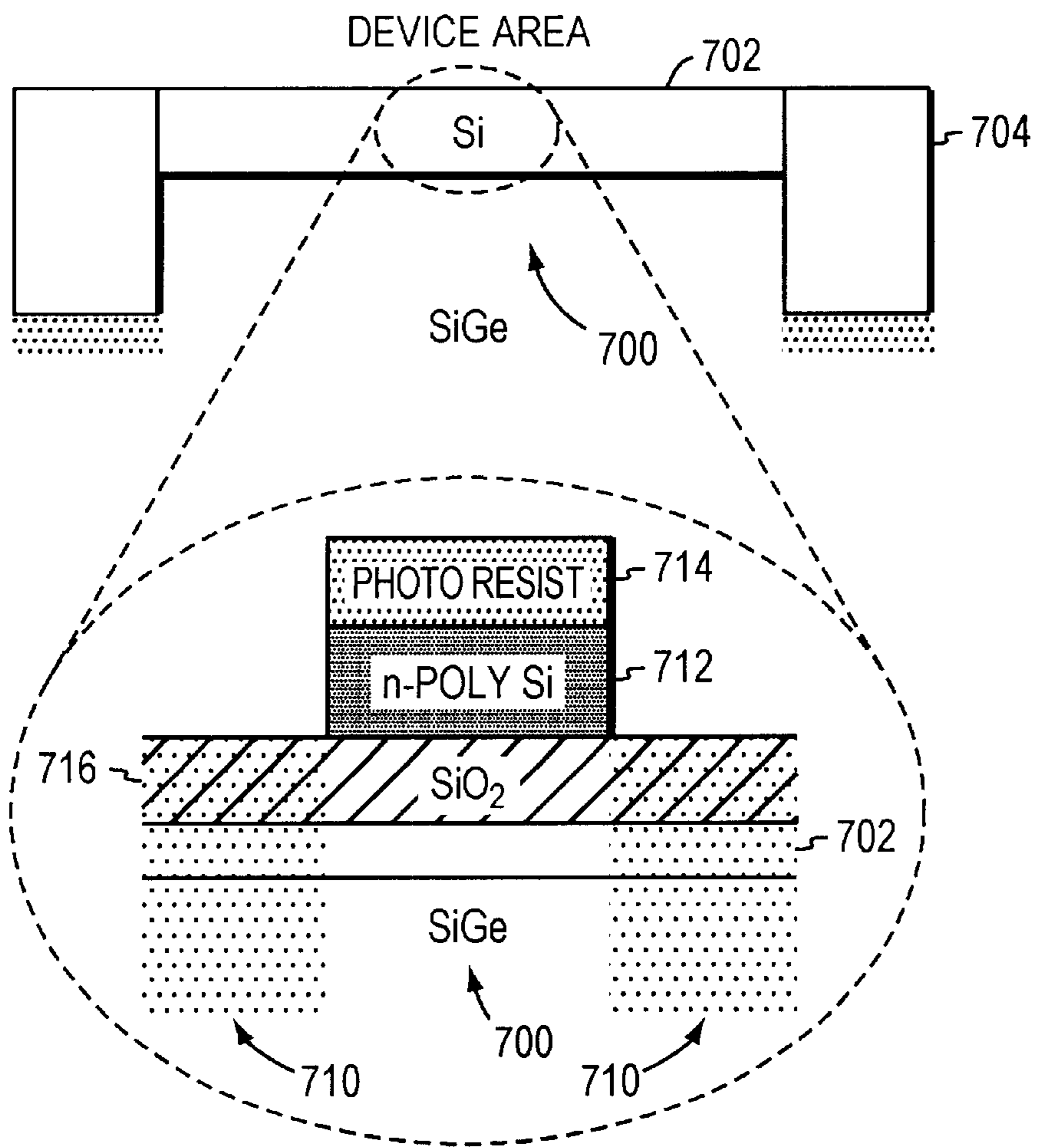
FIG. 7B
