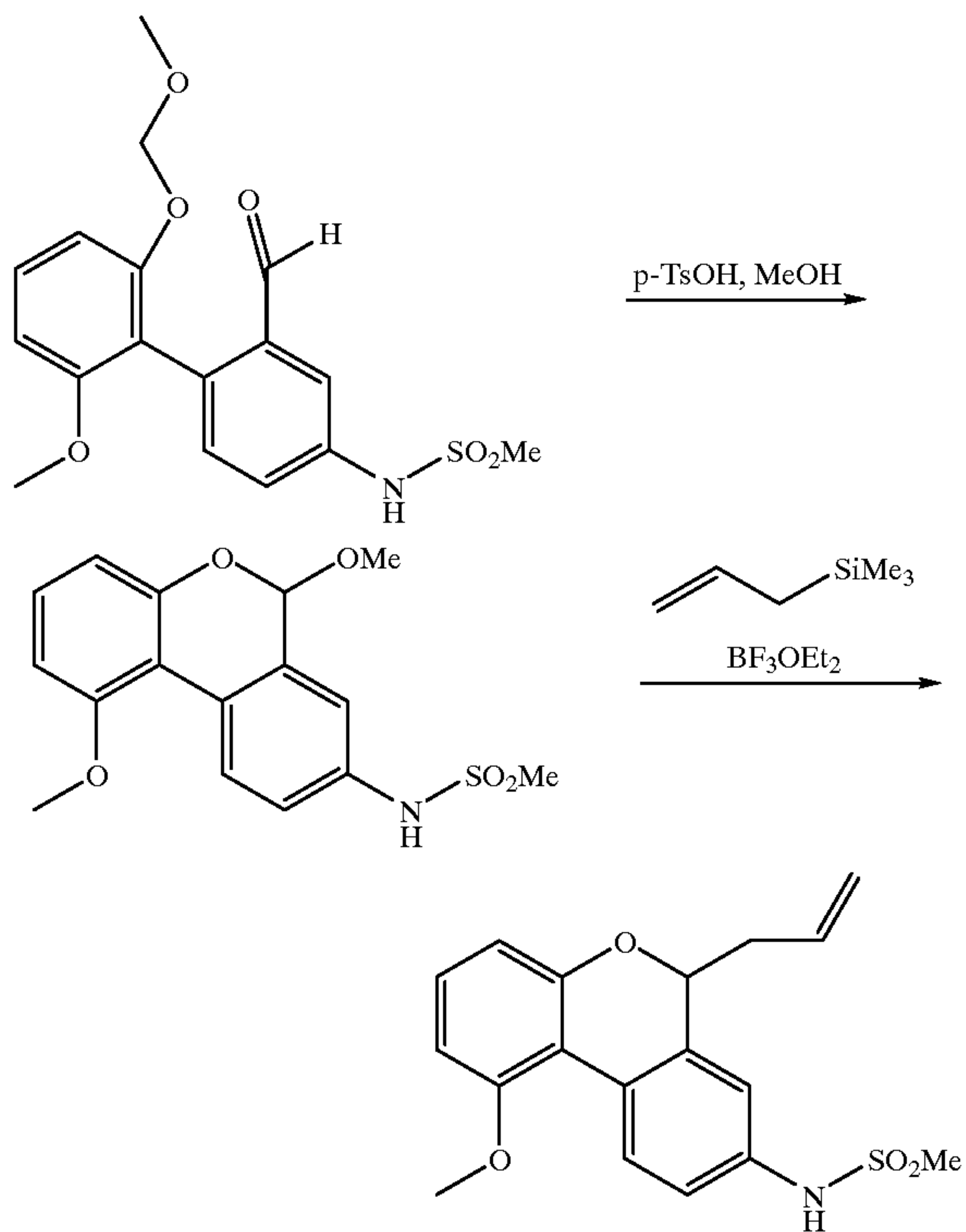
Scheme VI
