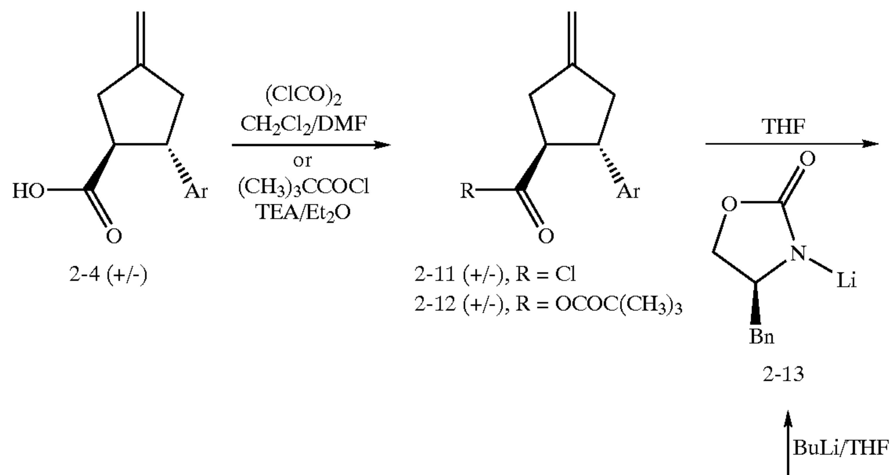
SCHEME 2A
