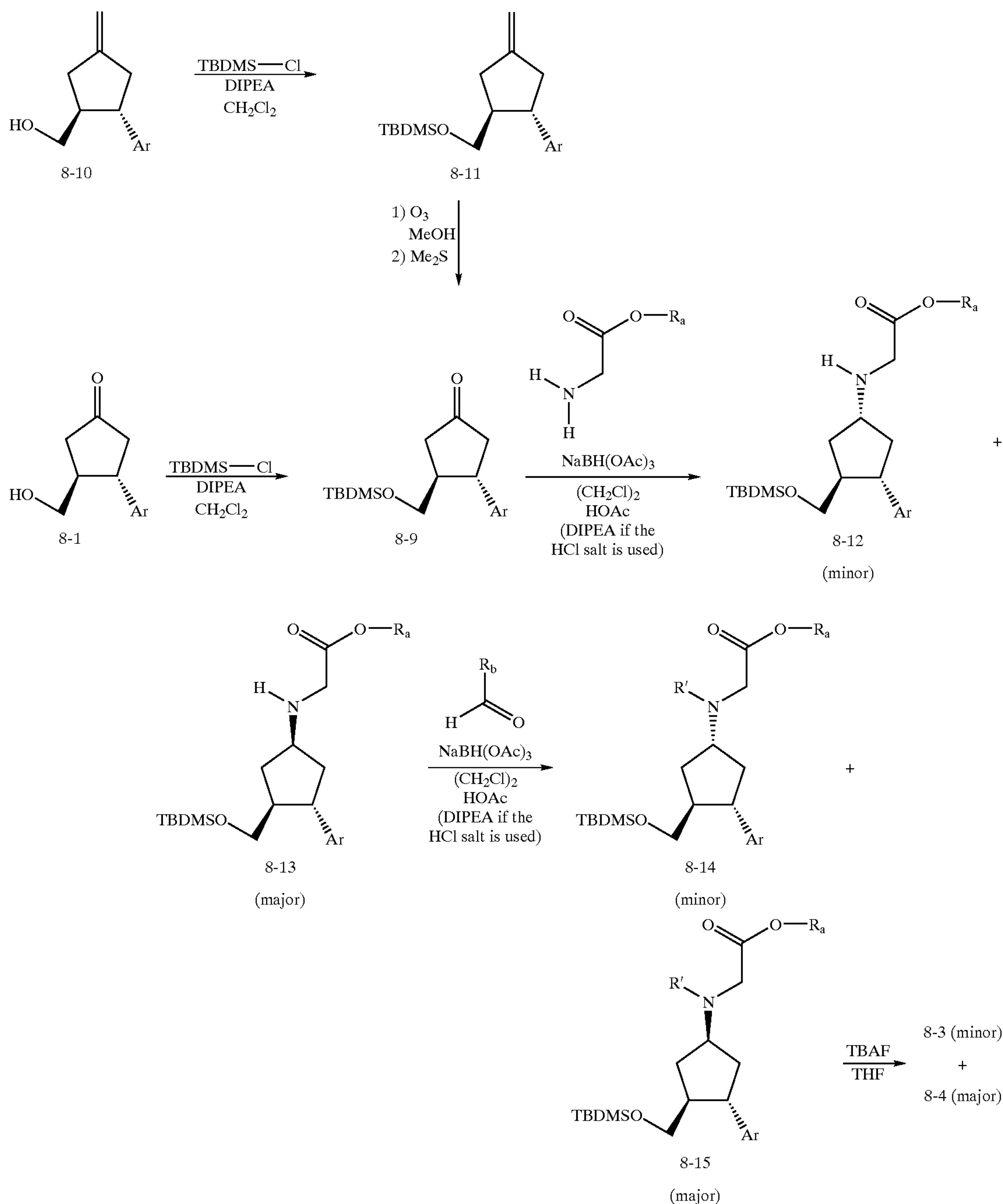
SCHEME 8A
