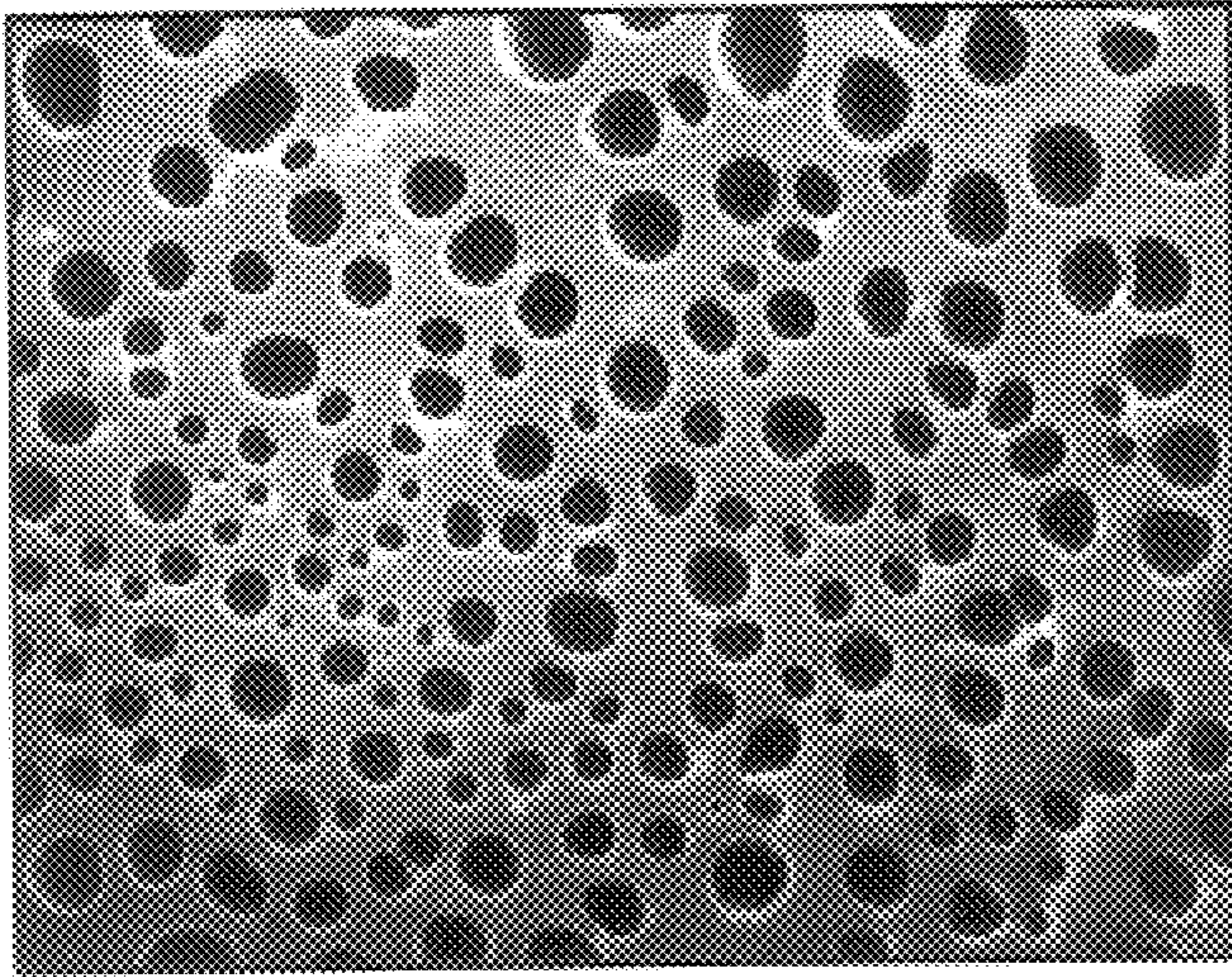
FIG. 41d —— 10 \mu m 3.0 kV x 1.300 10mm
