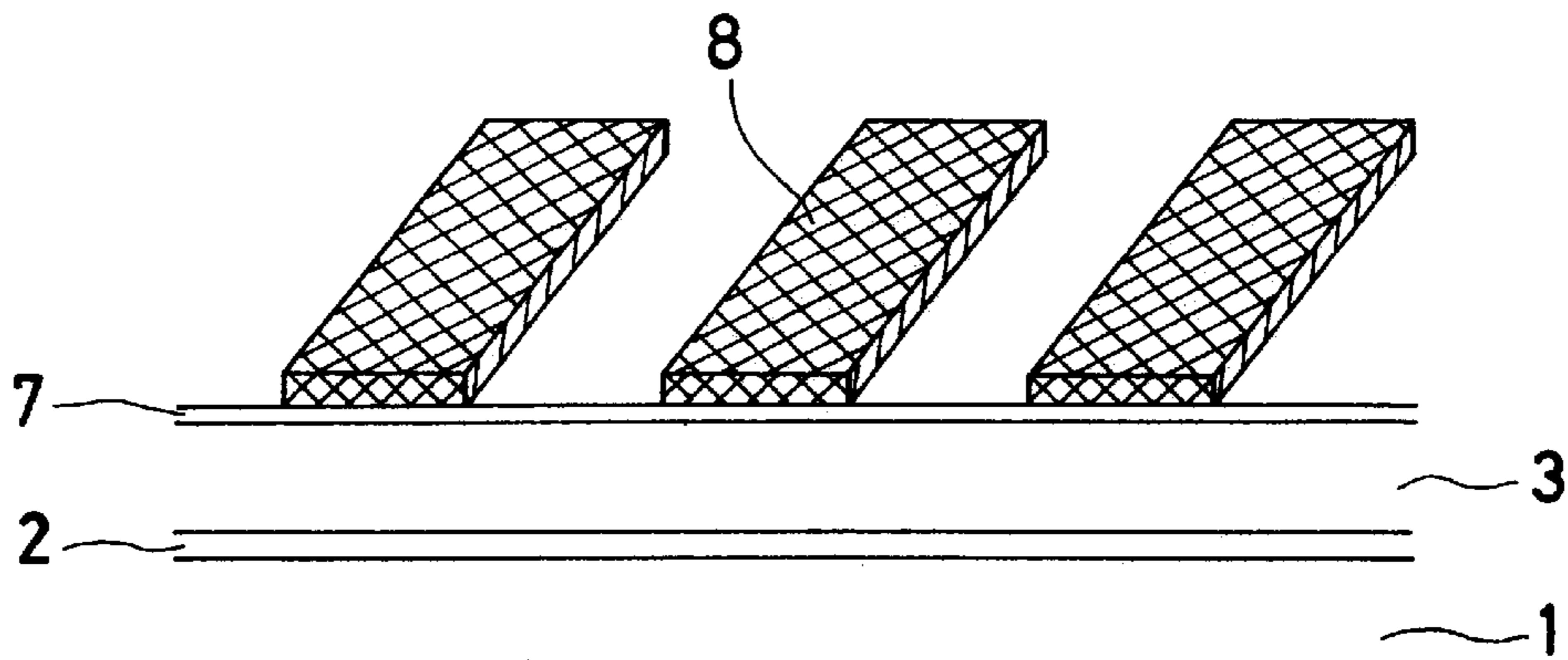
FIG. 2 (b)
