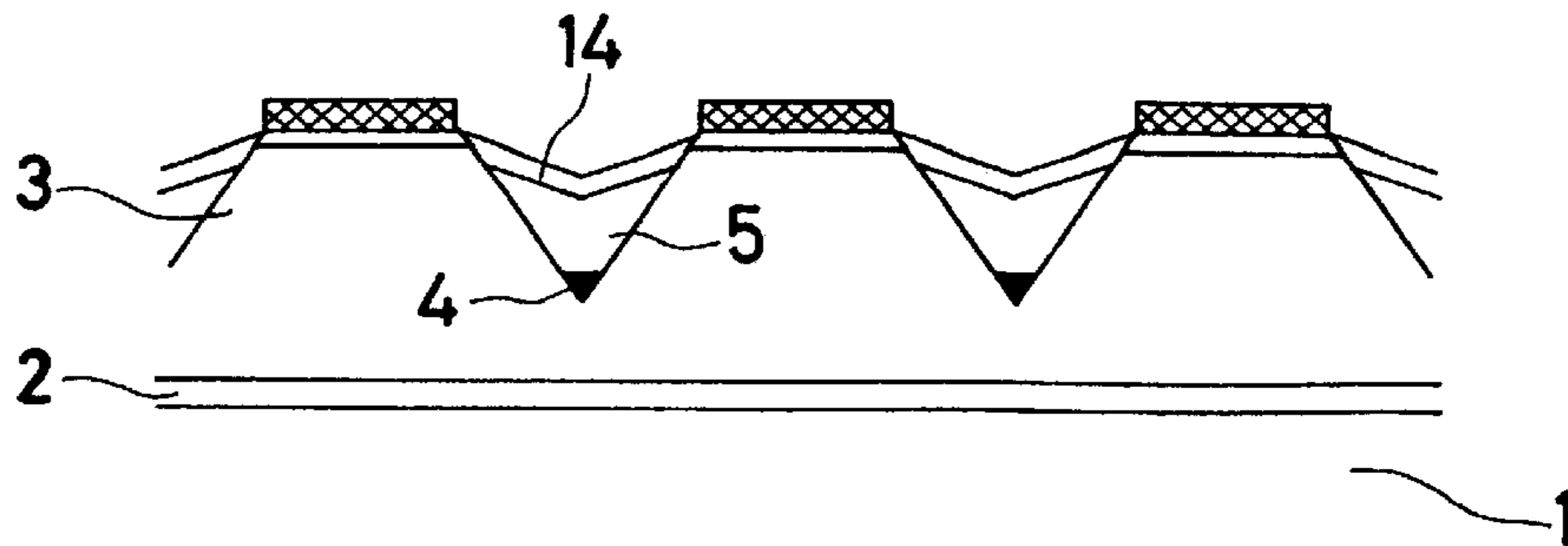
FIG. 2 (d)
