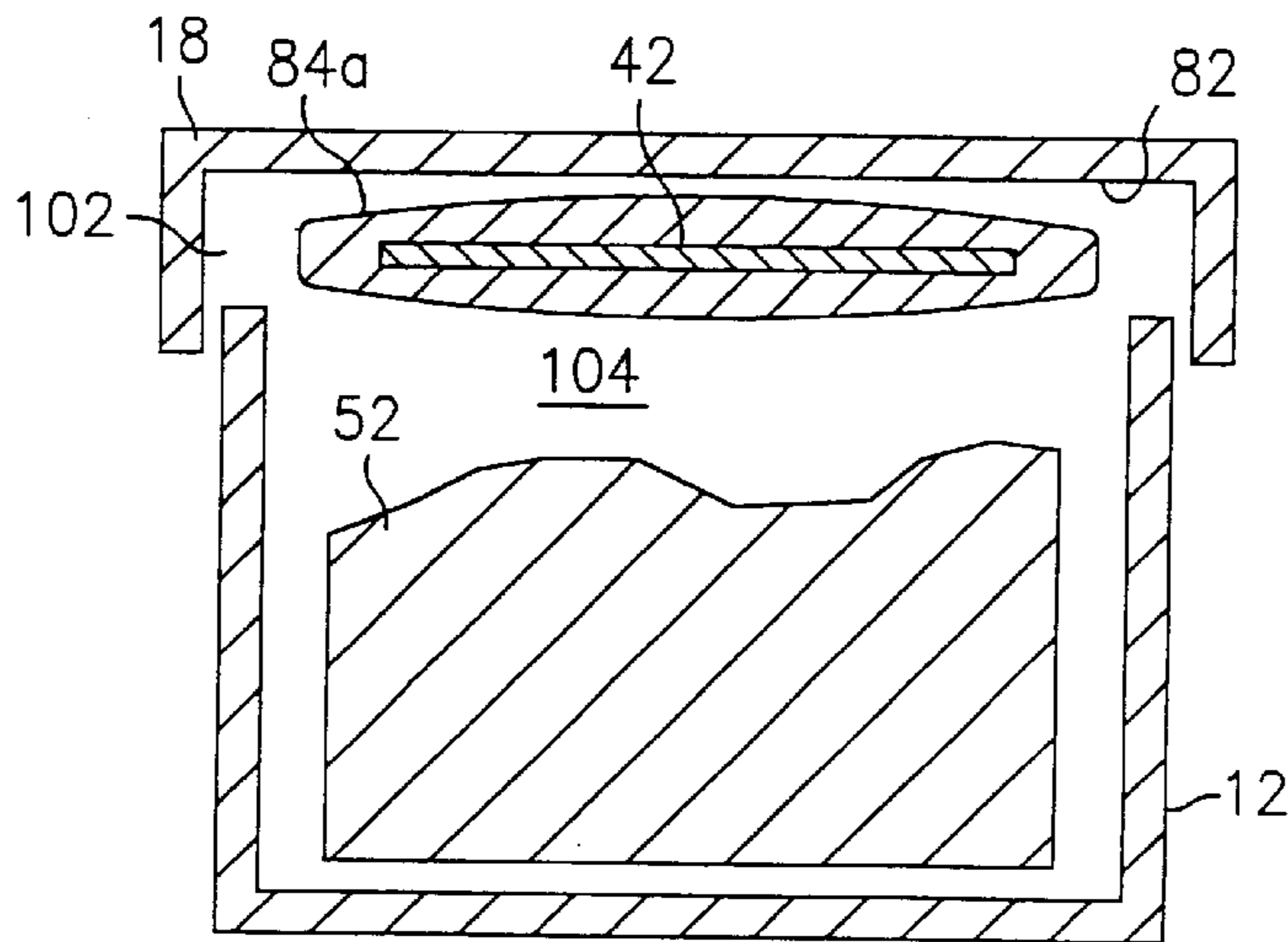
FIG. 7A
