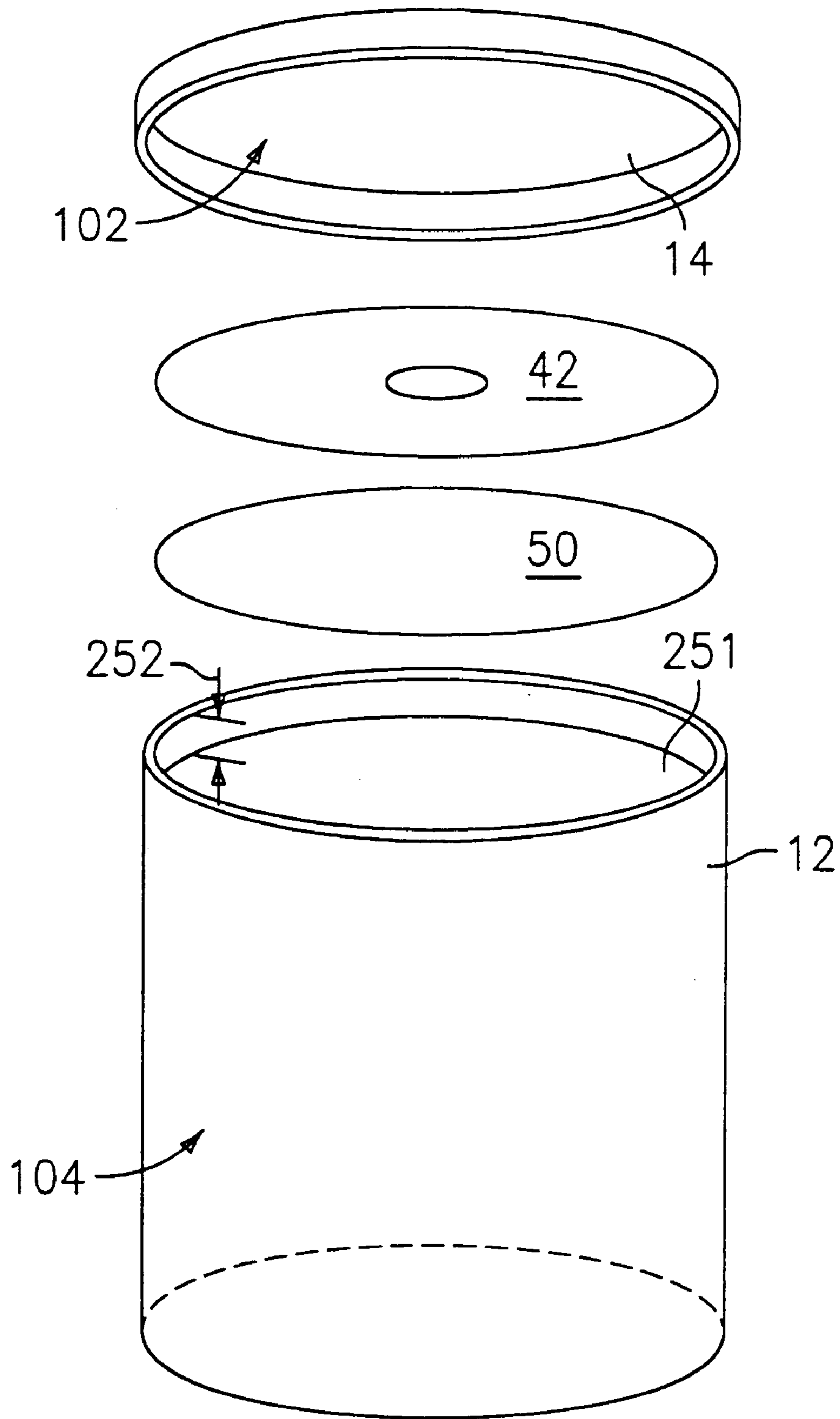
FIG. 14
