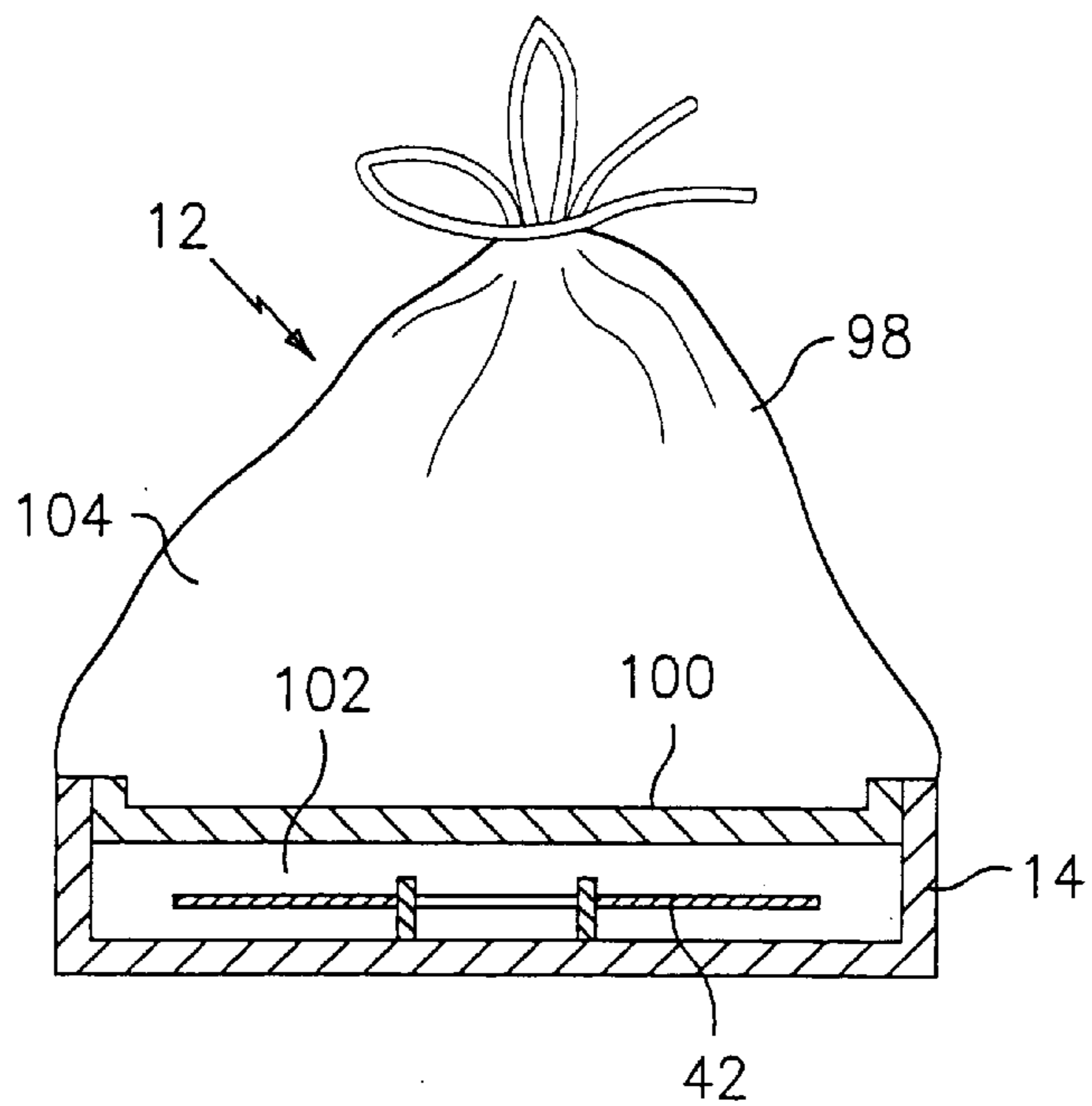
FIG. 8A
