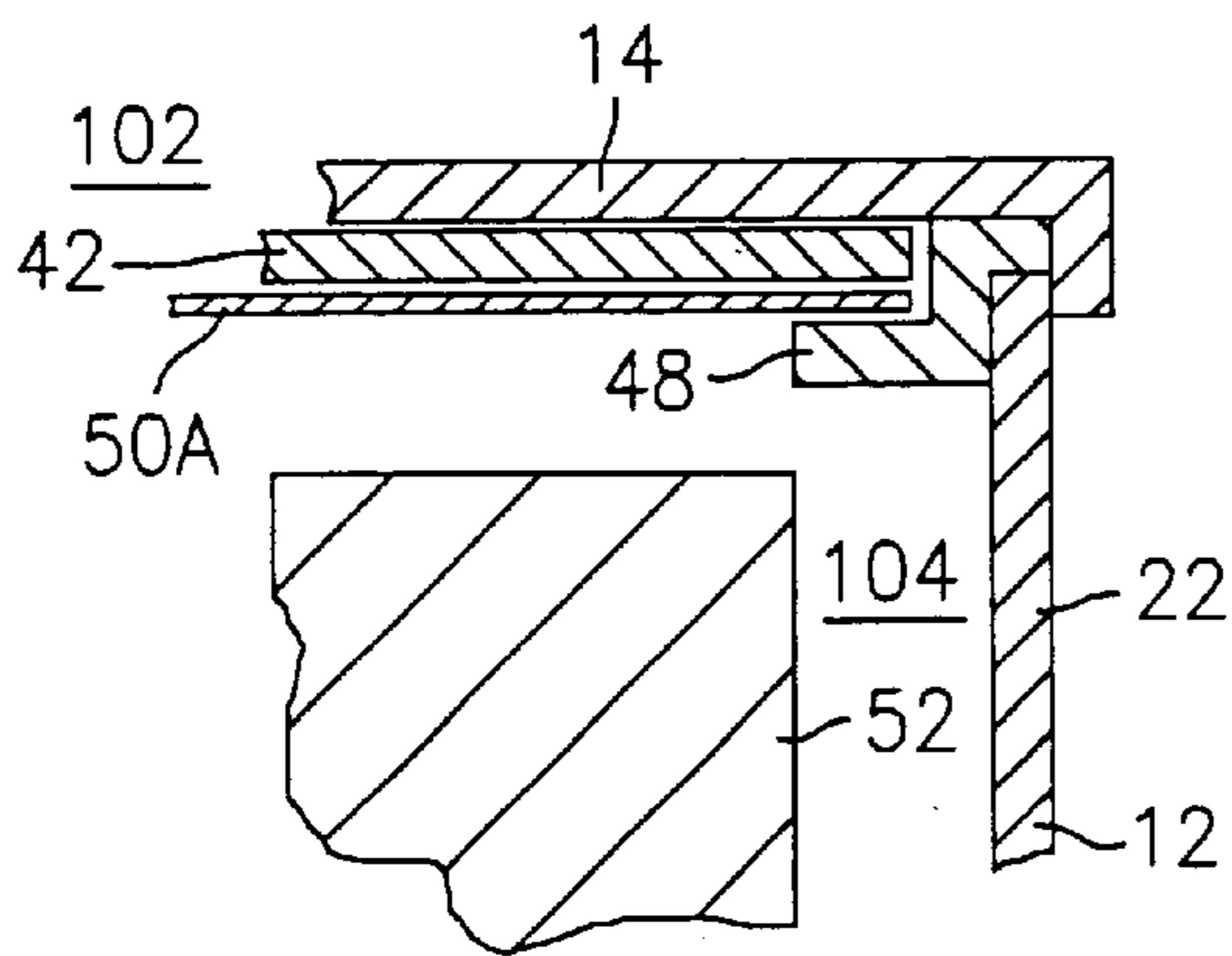
FIG. 2B
