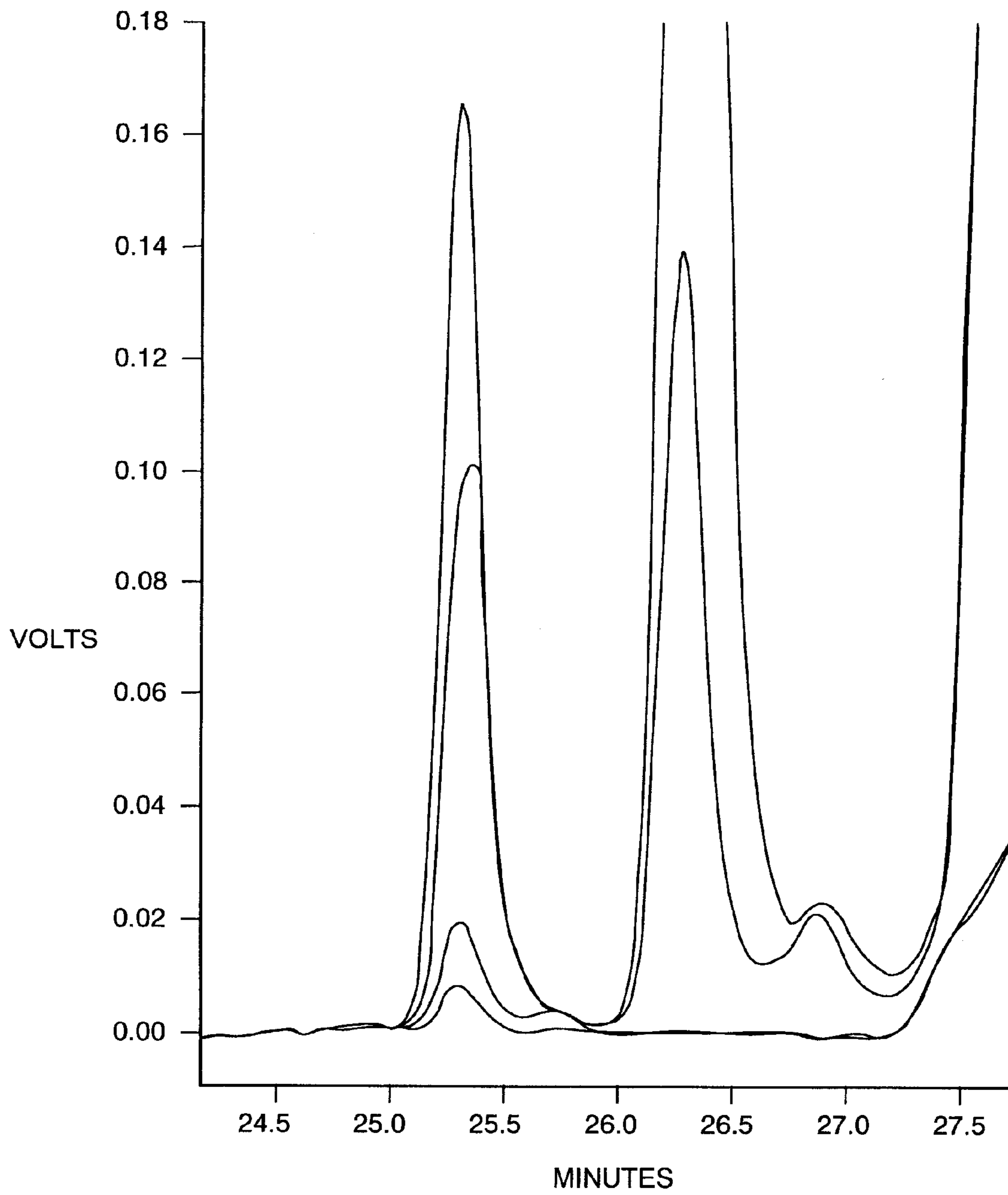
FIG. 4
