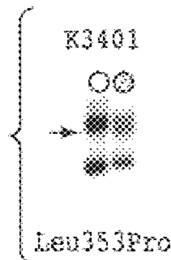
Leu353Pro FIG. 12N
