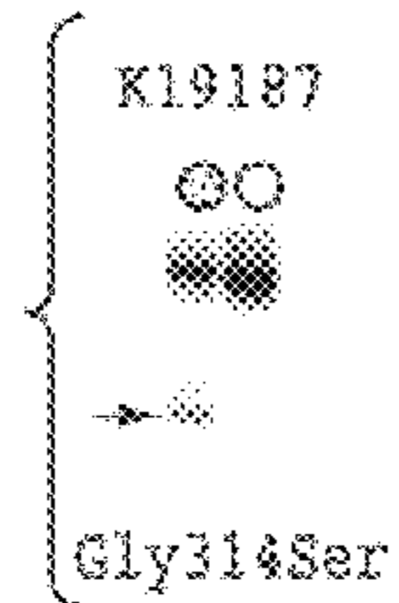
Gly314Ser FIG. 12K
