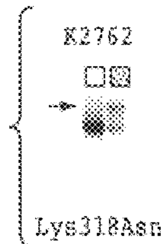
Lys318Asn FIG. 12M
