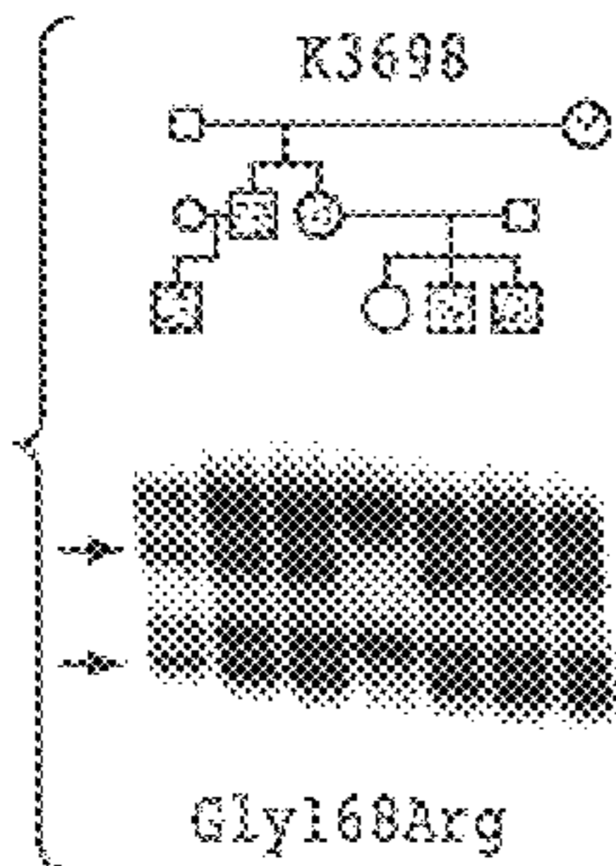
Gly168Arg FIG. 12J
