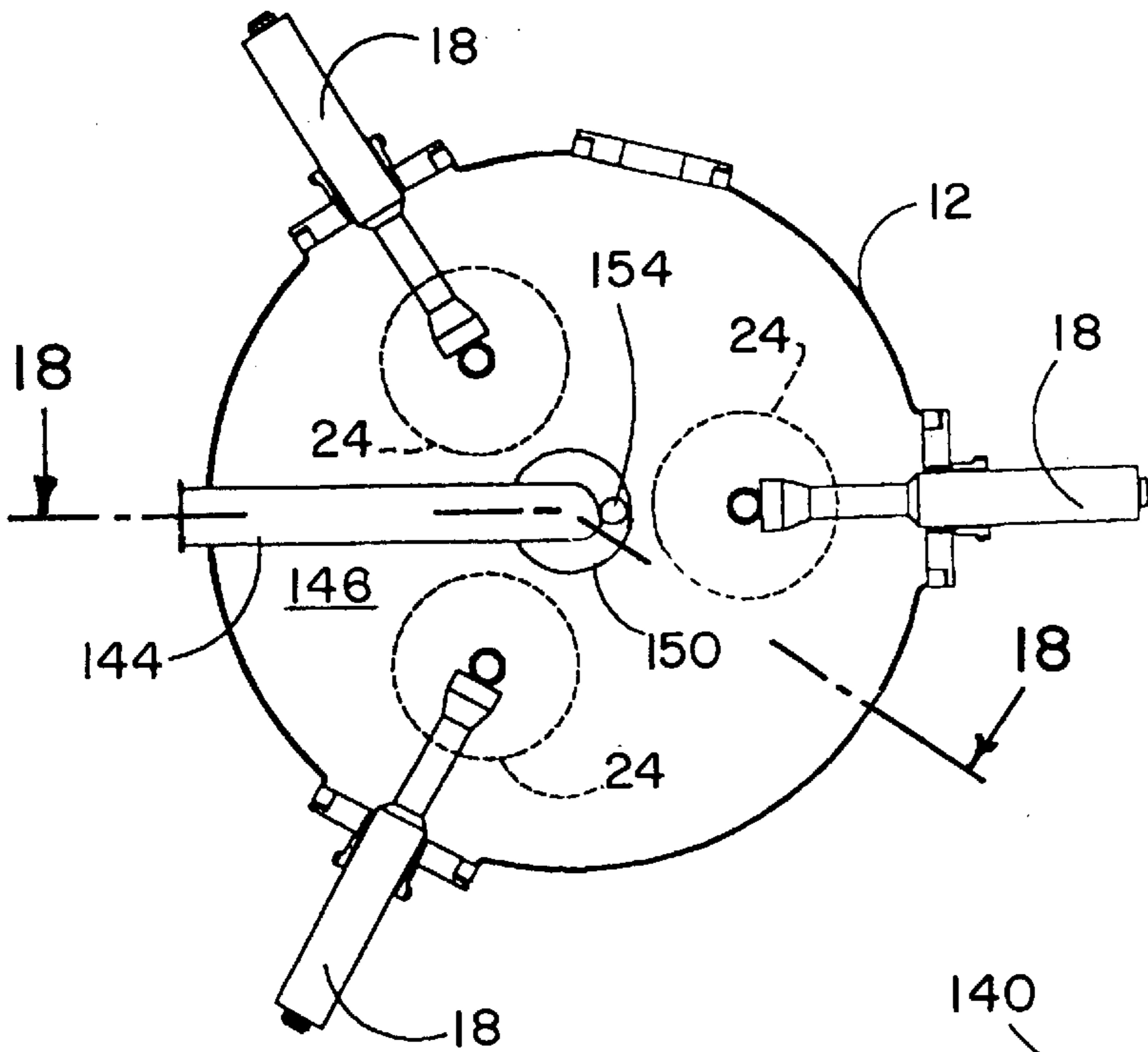
FIG. 19
