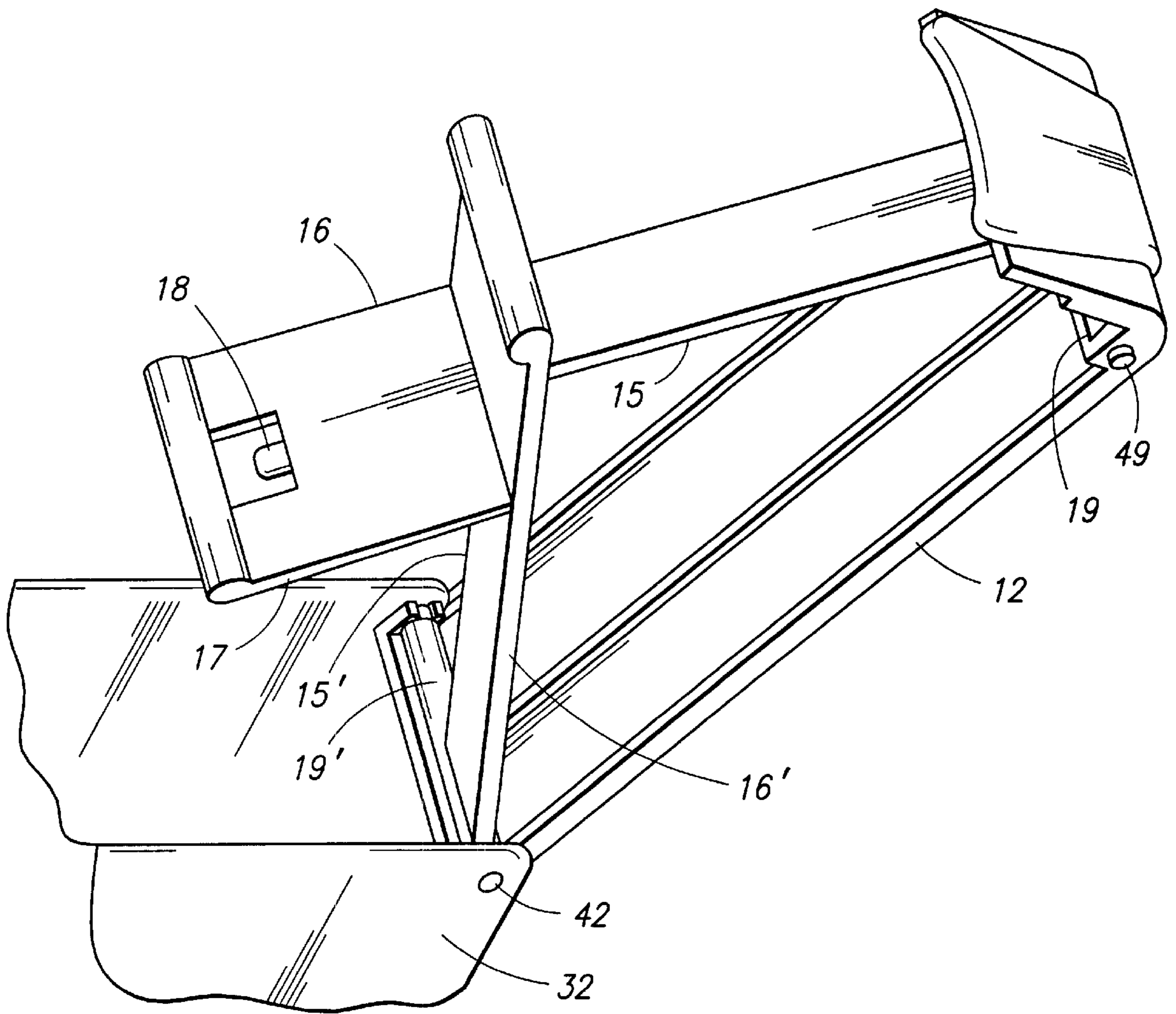
FIG. 2A
