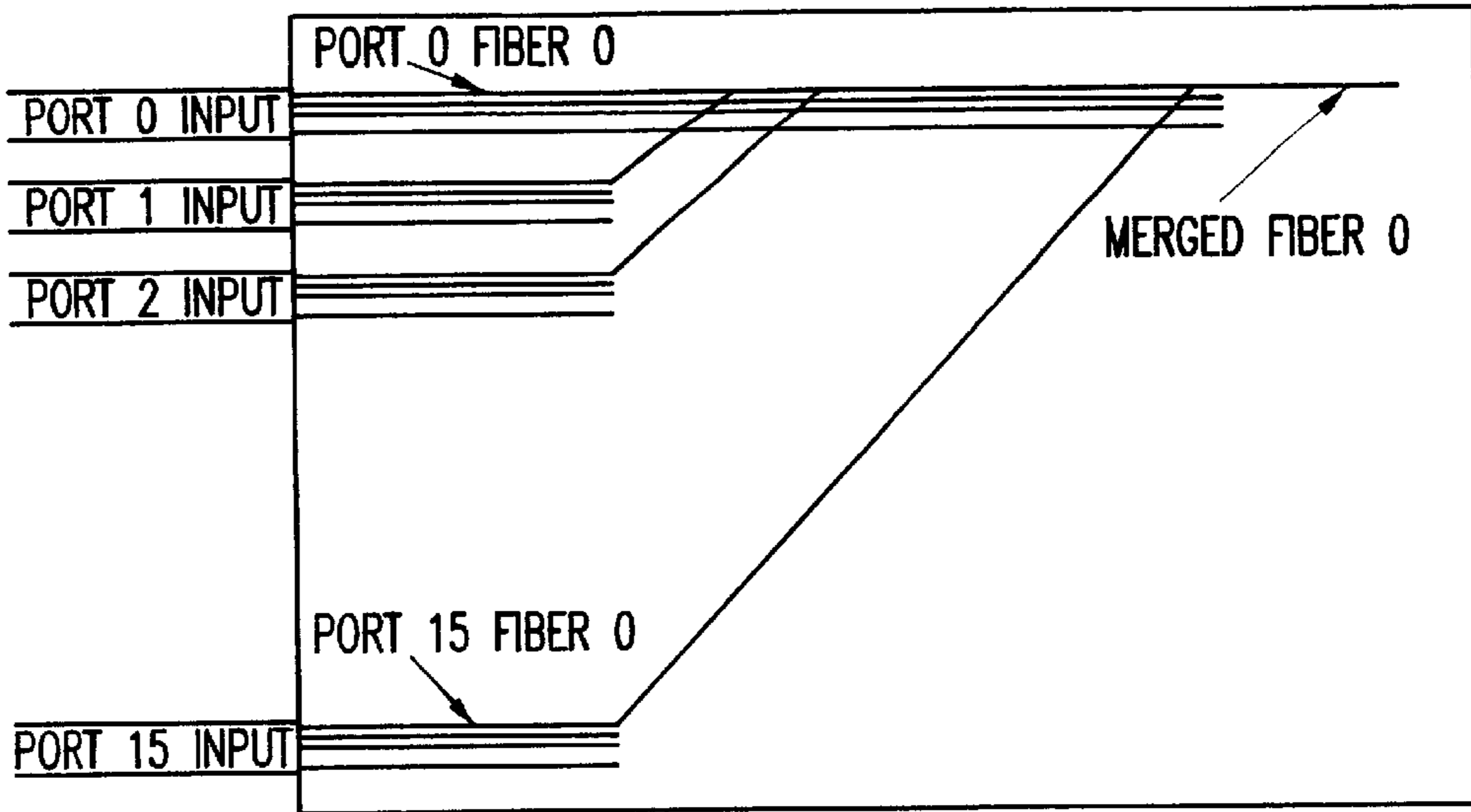
FIG.6
