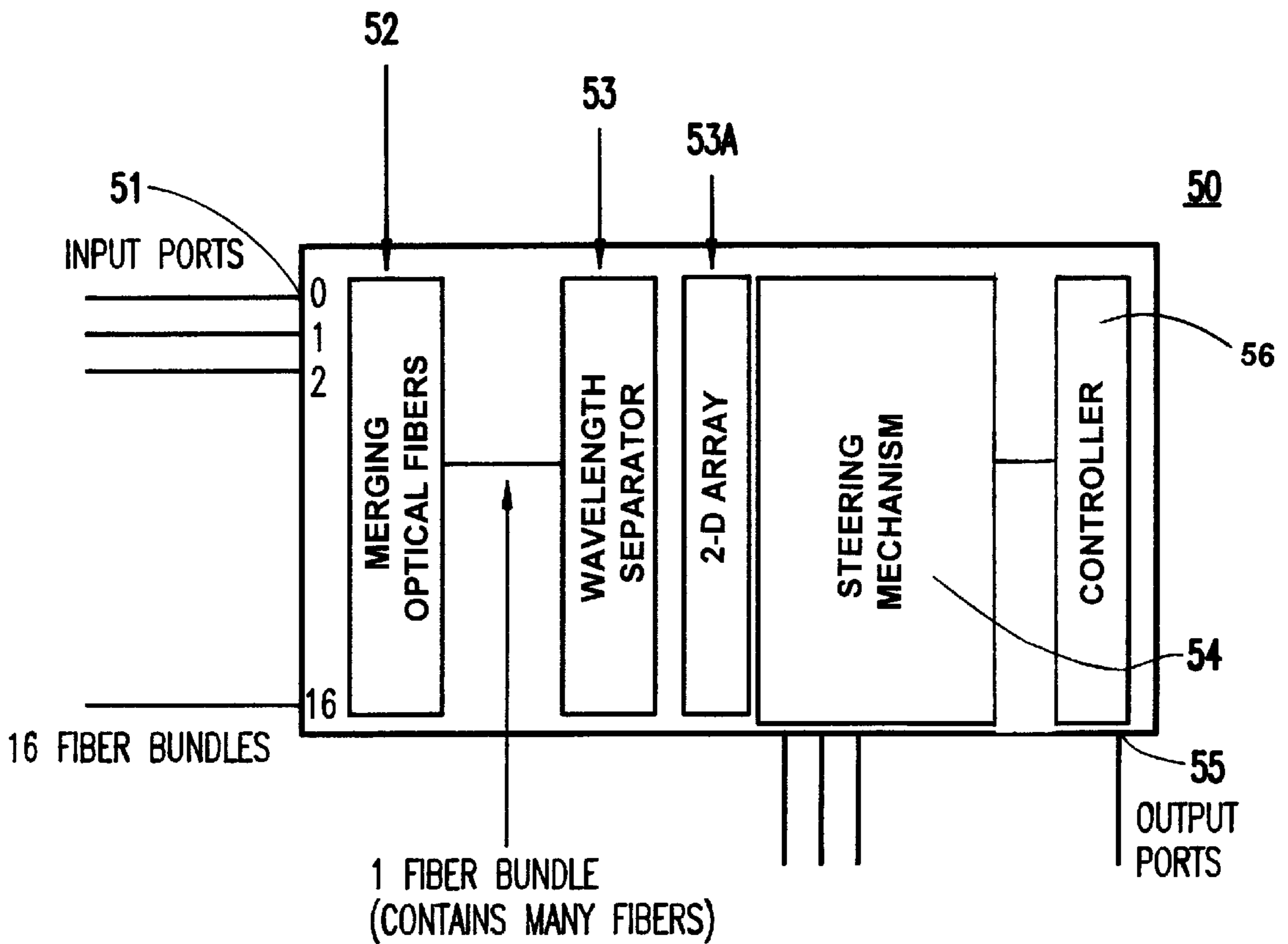
FIG.5B
