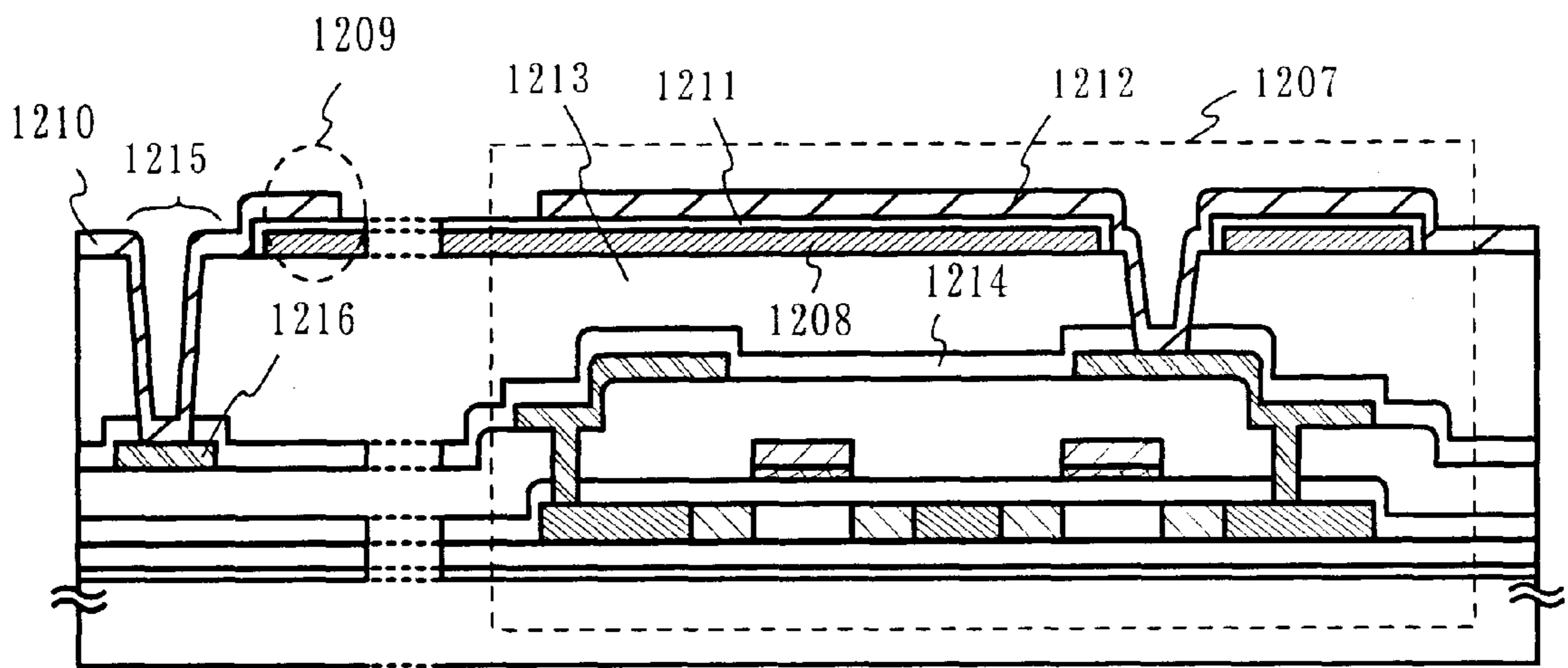
FIG. 12B
