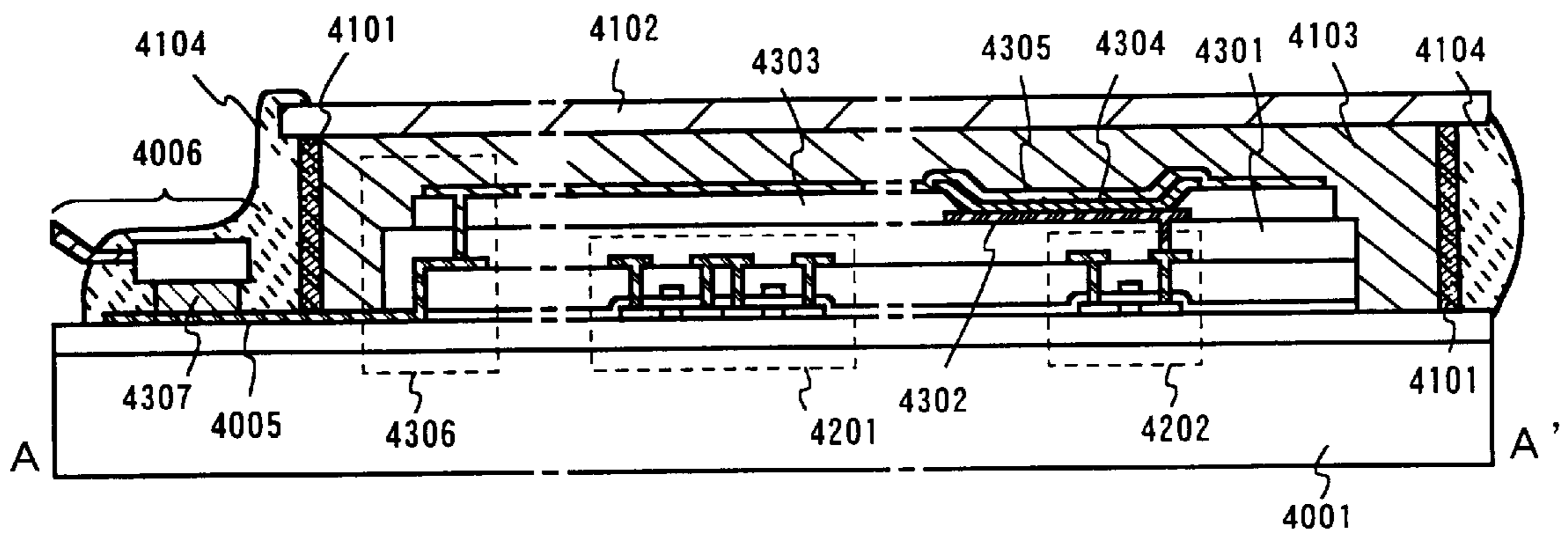
FIG. 25B
