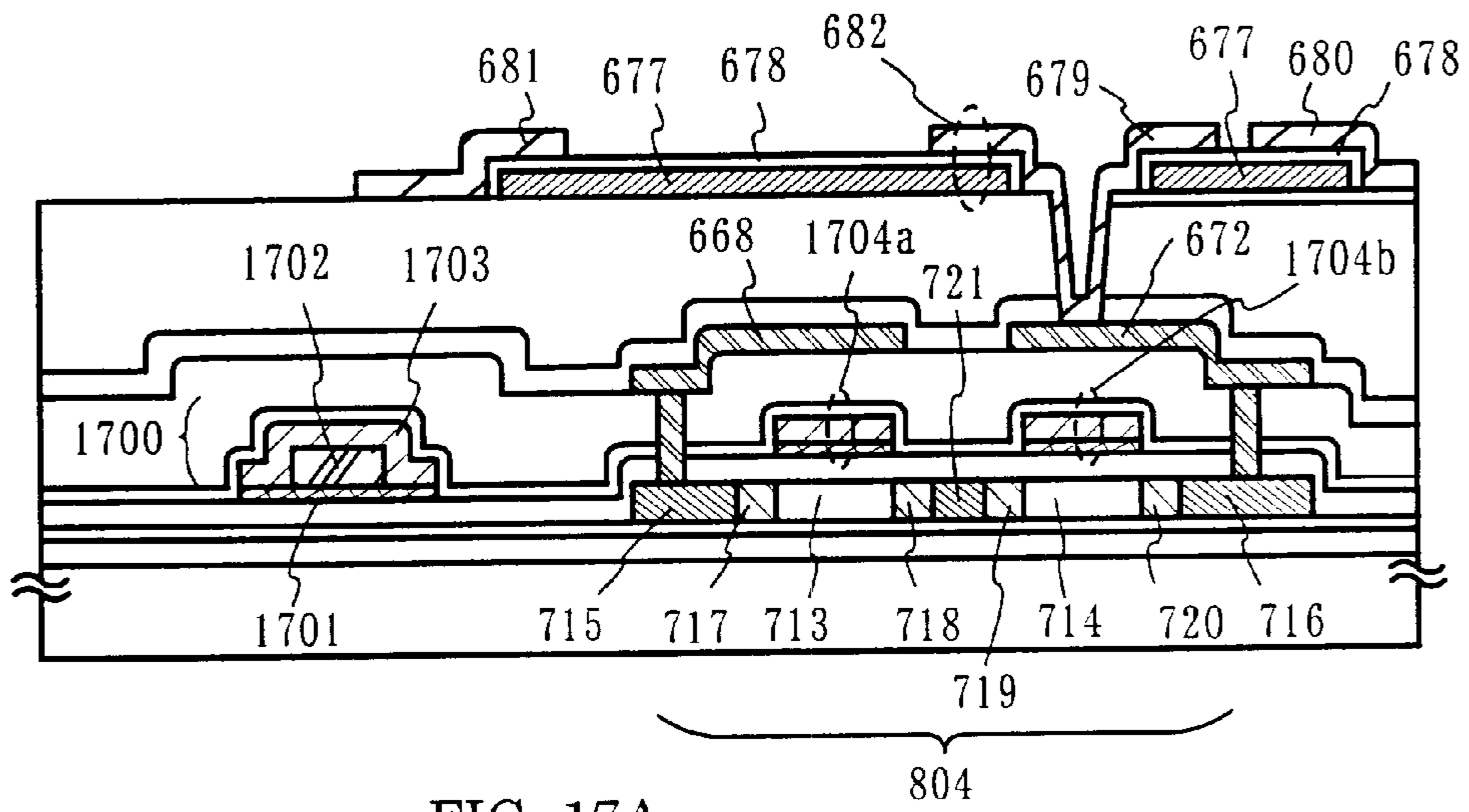
FIG. 17A
