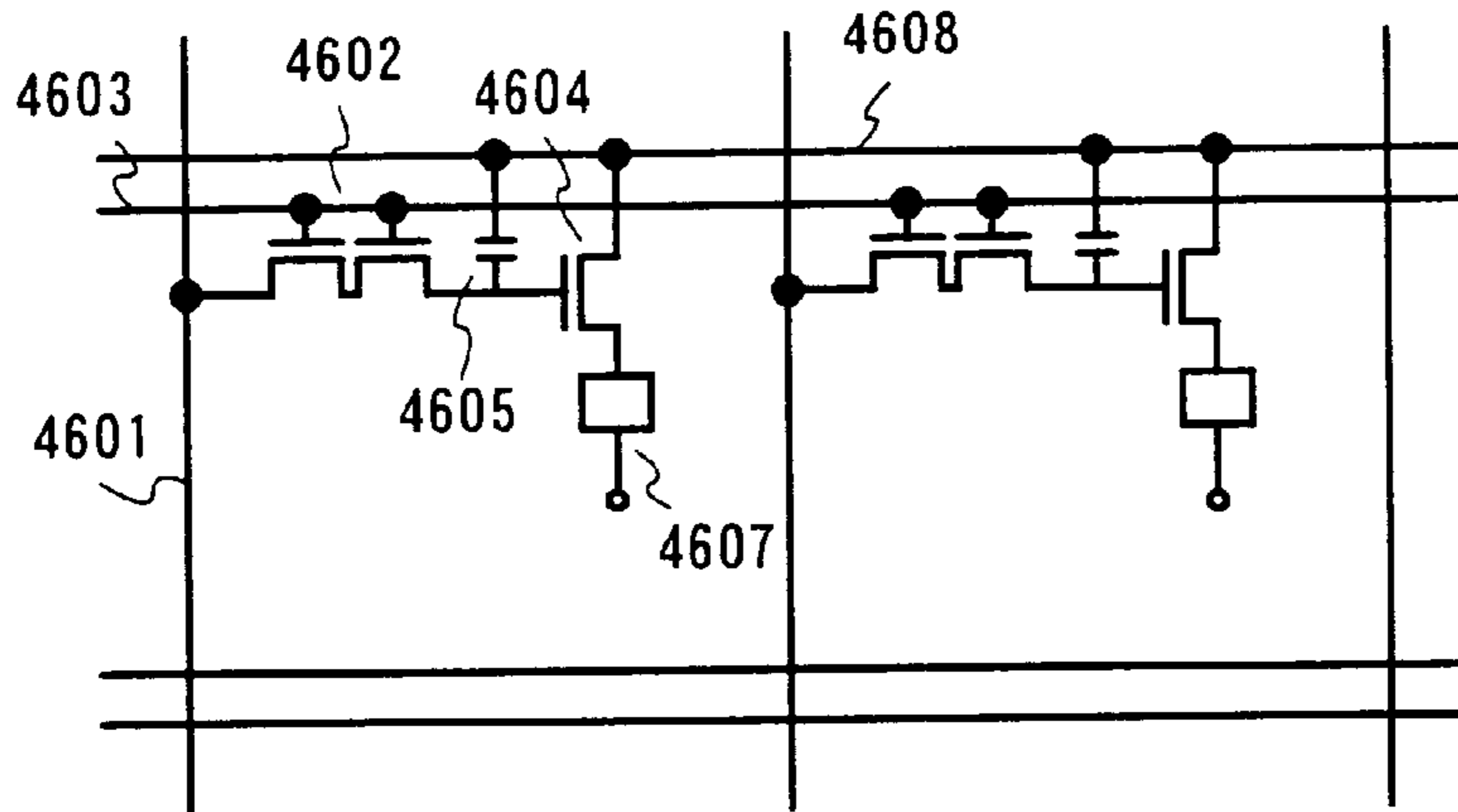
FIG. 29B
