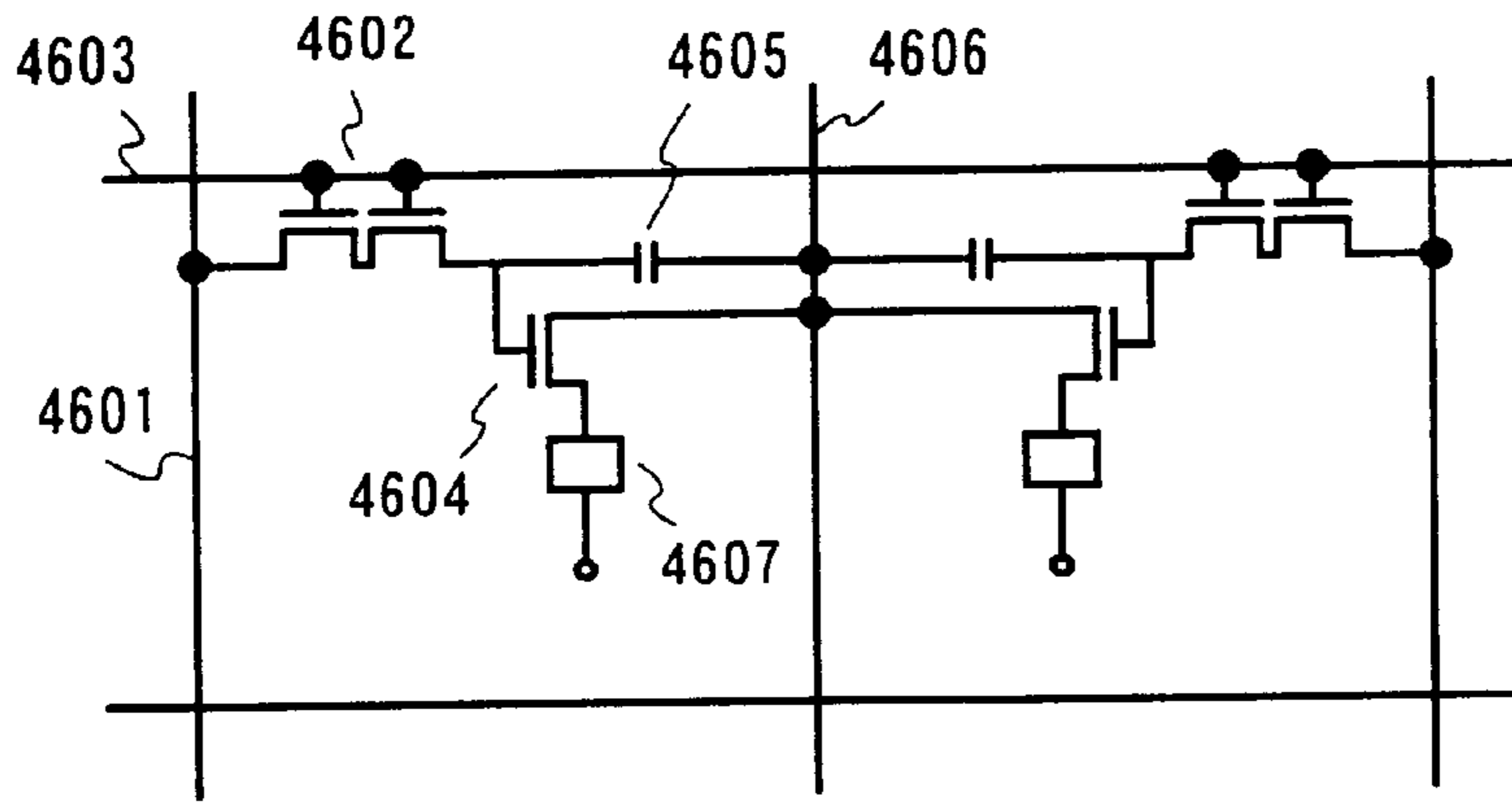
FIG. 29A
