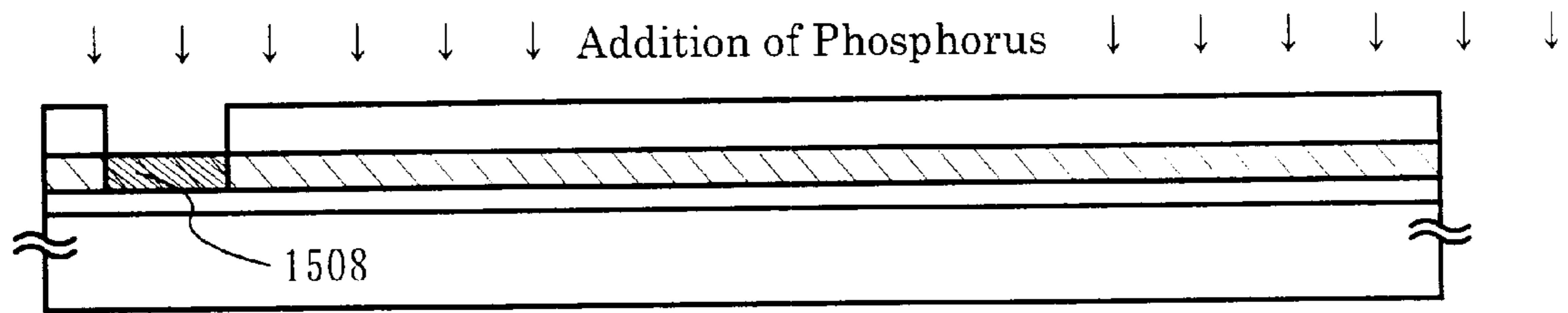
FIG. 15C
