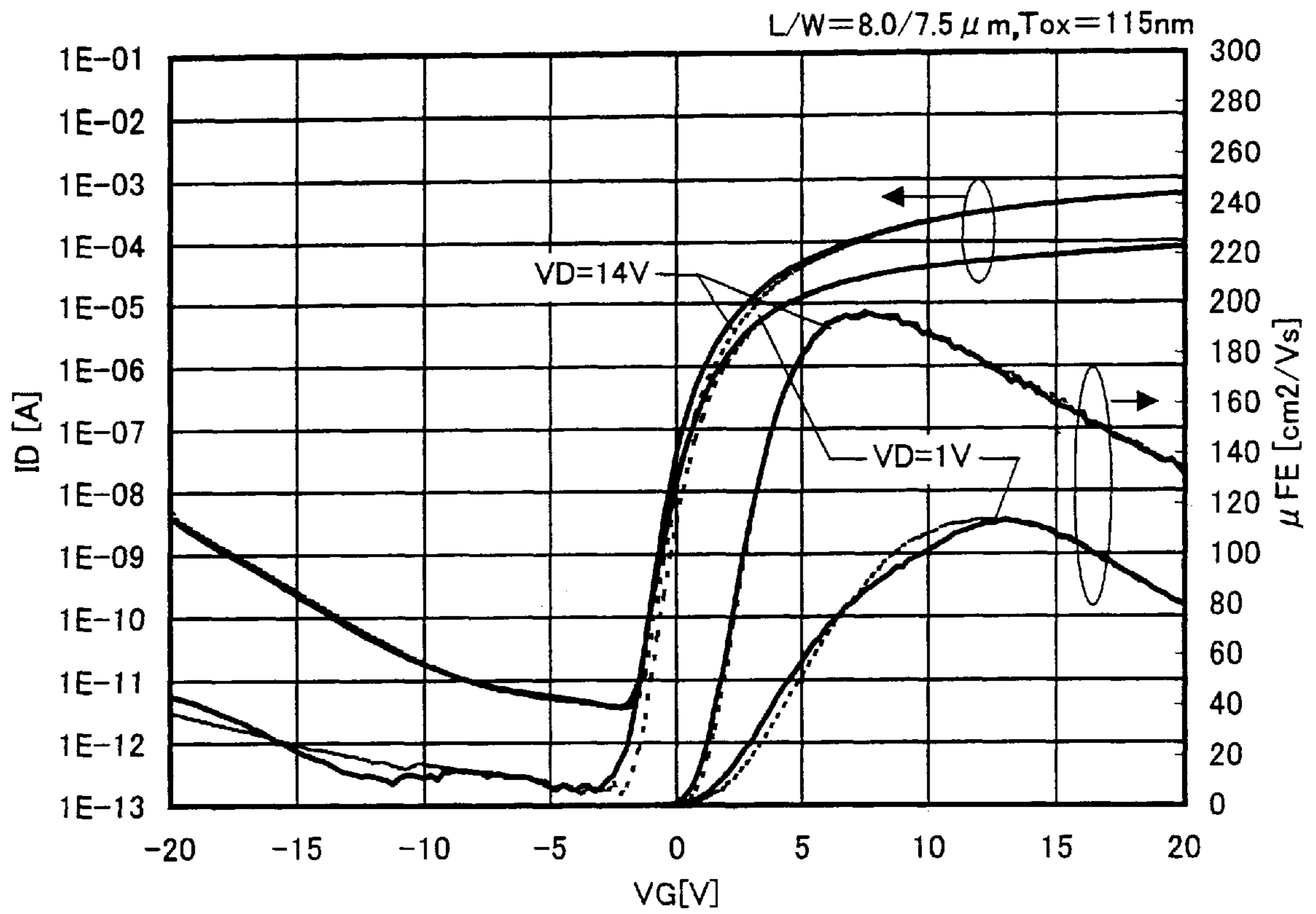
FIG. 33
