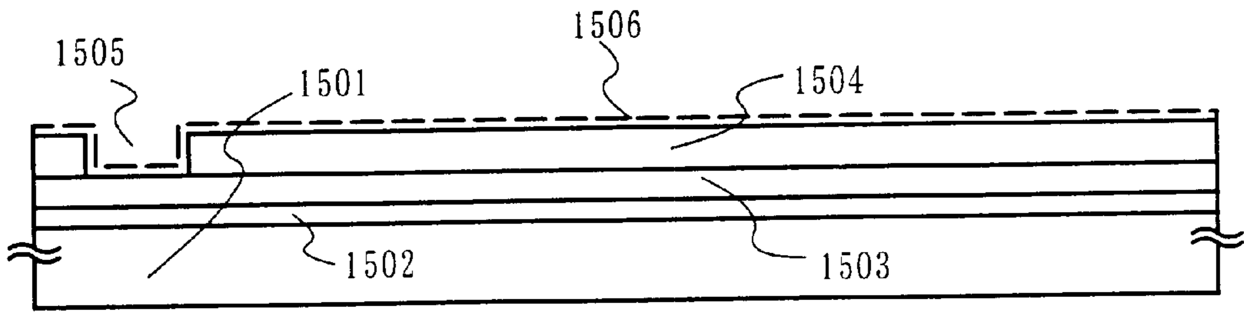
FIG. 15A
