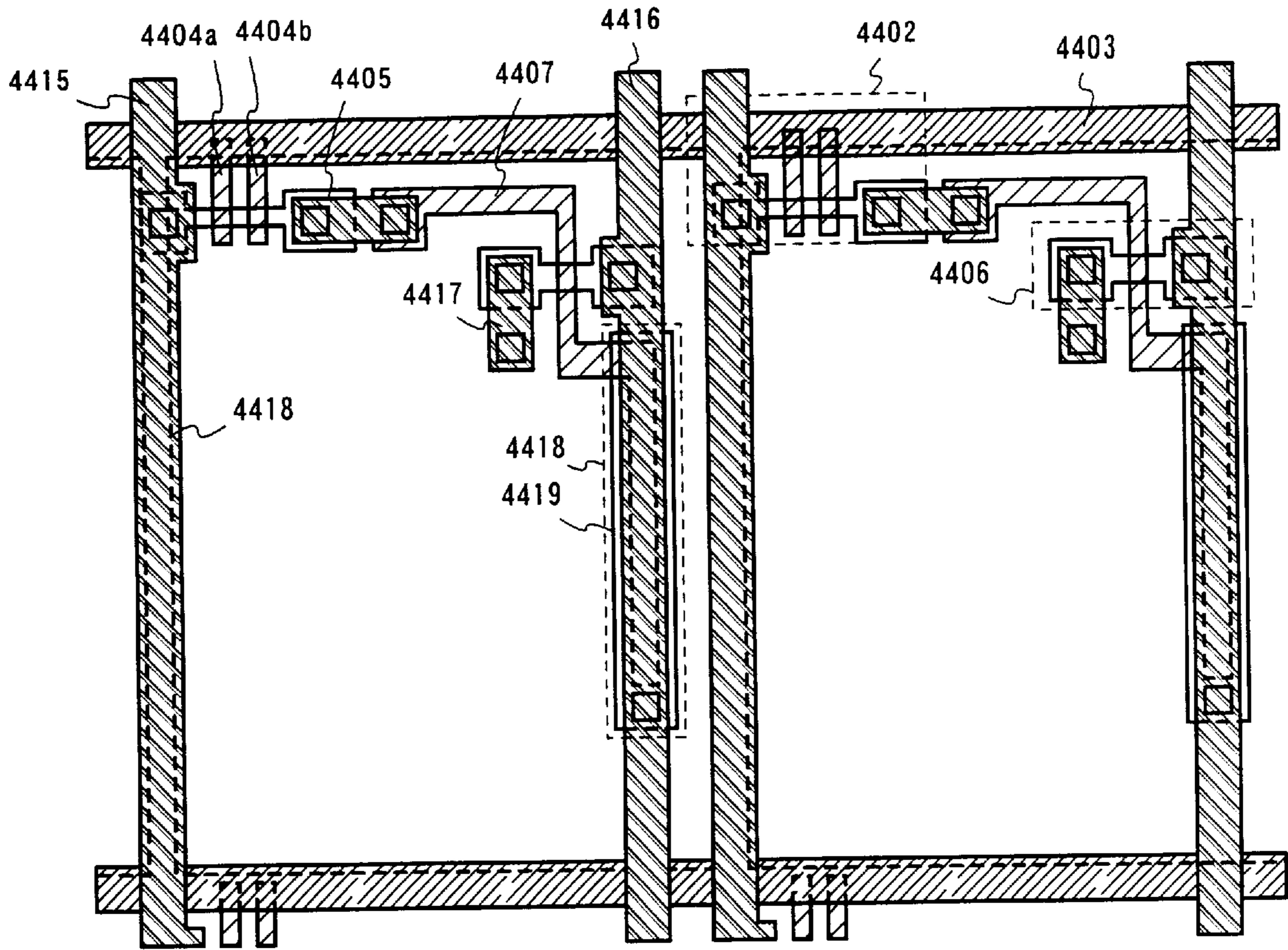
FIG. 27A
