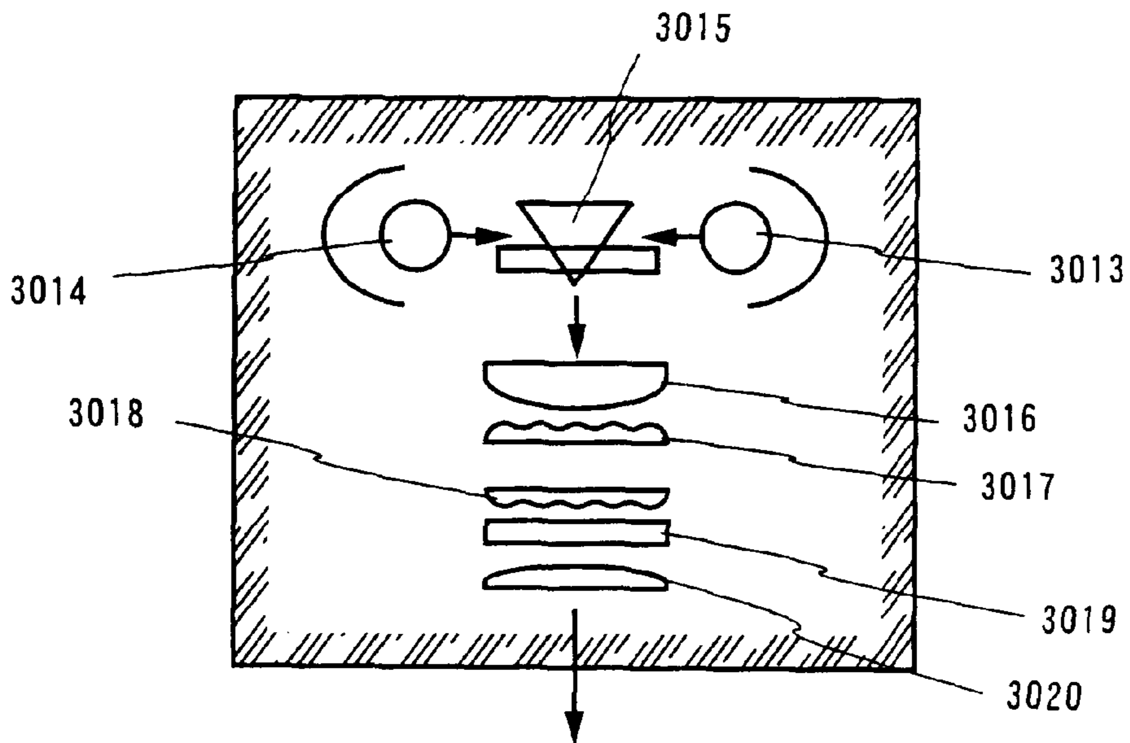
FIG. 32B
