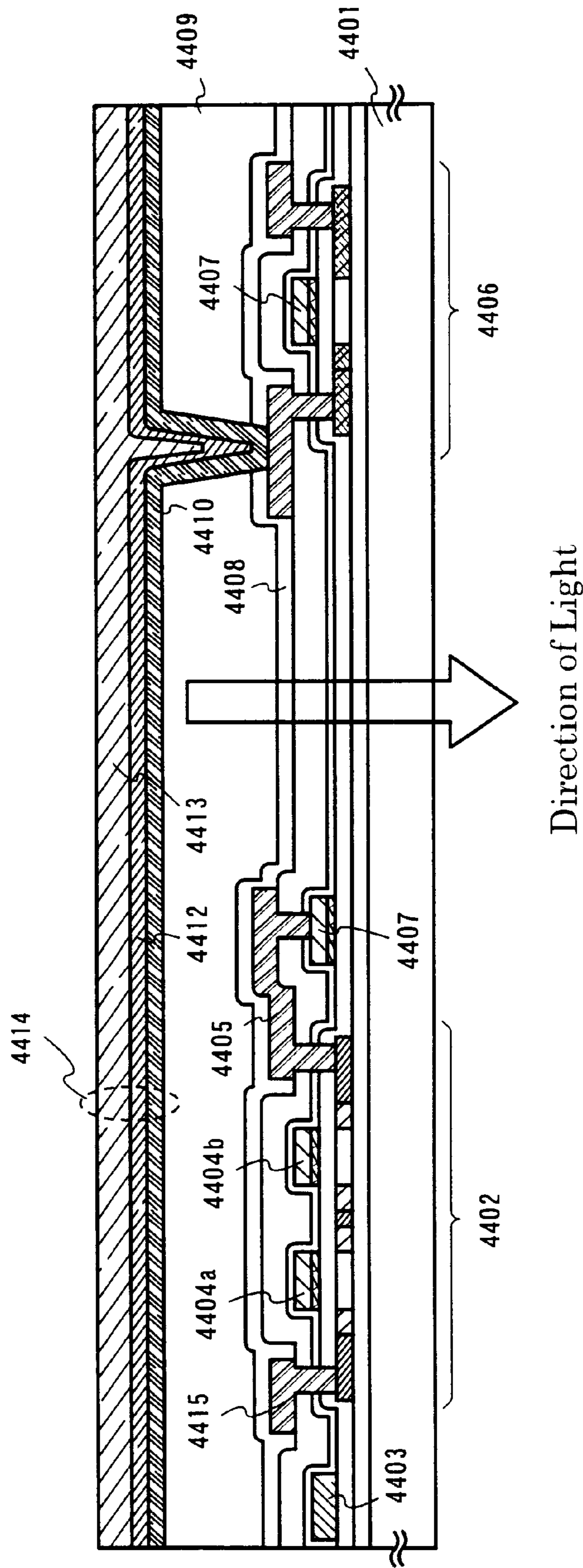
FIG. 26
