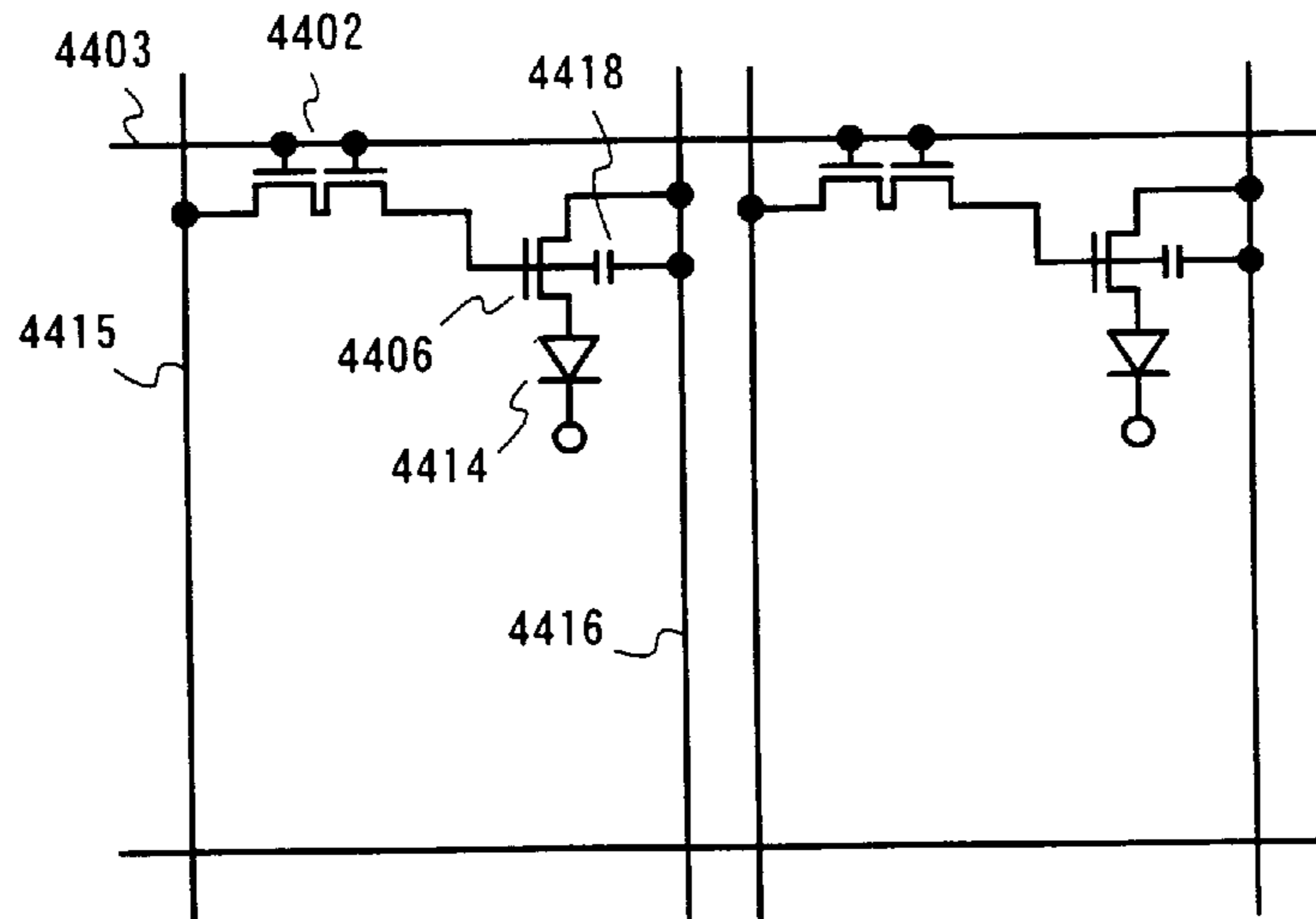
FIG. 27B
