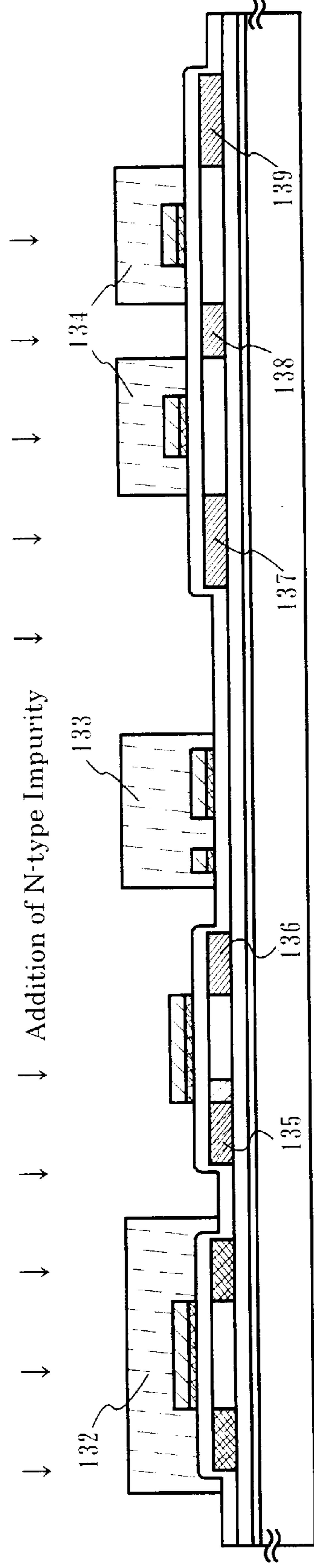
FIG. 2C
