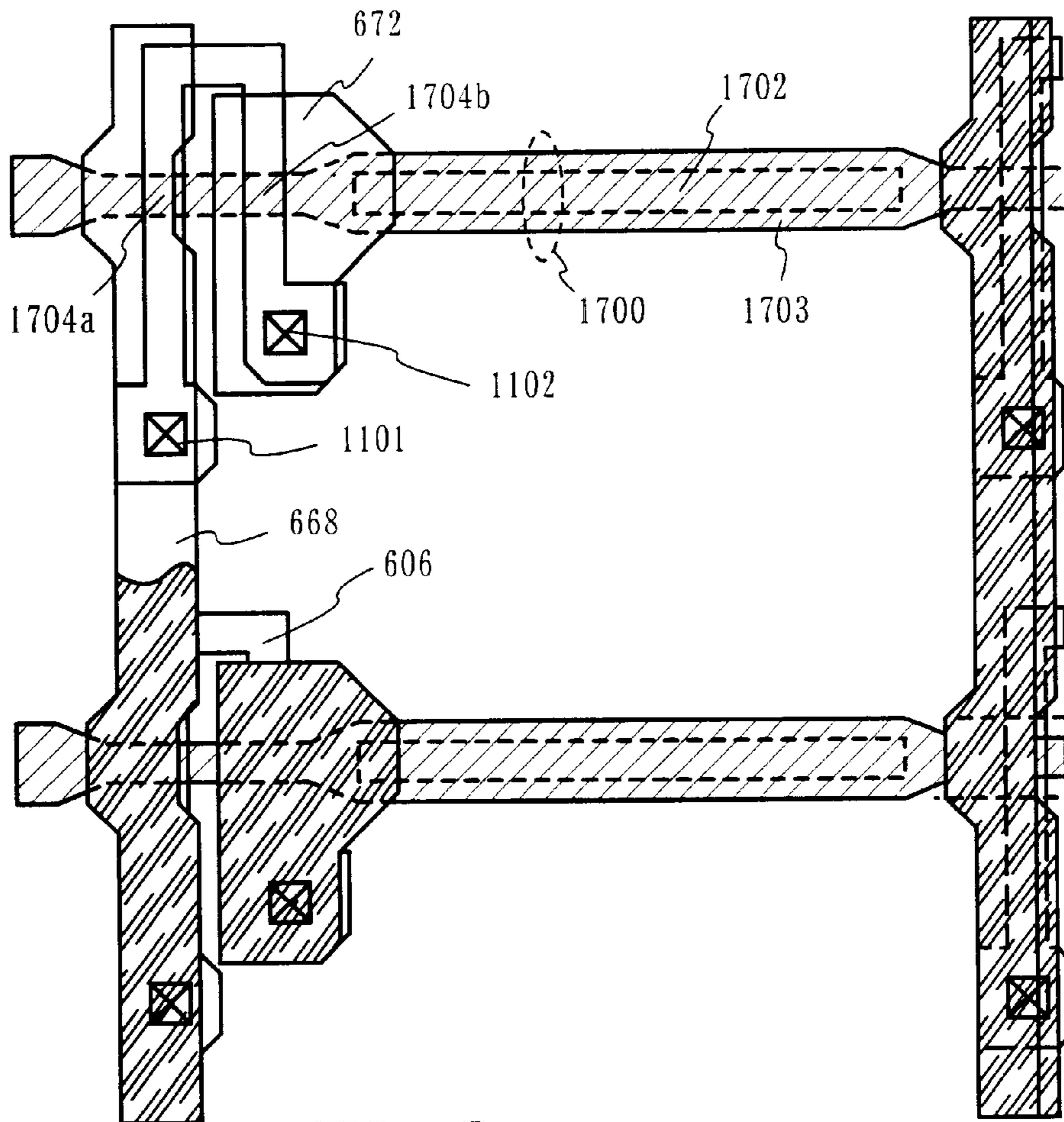
FIG. 17B
