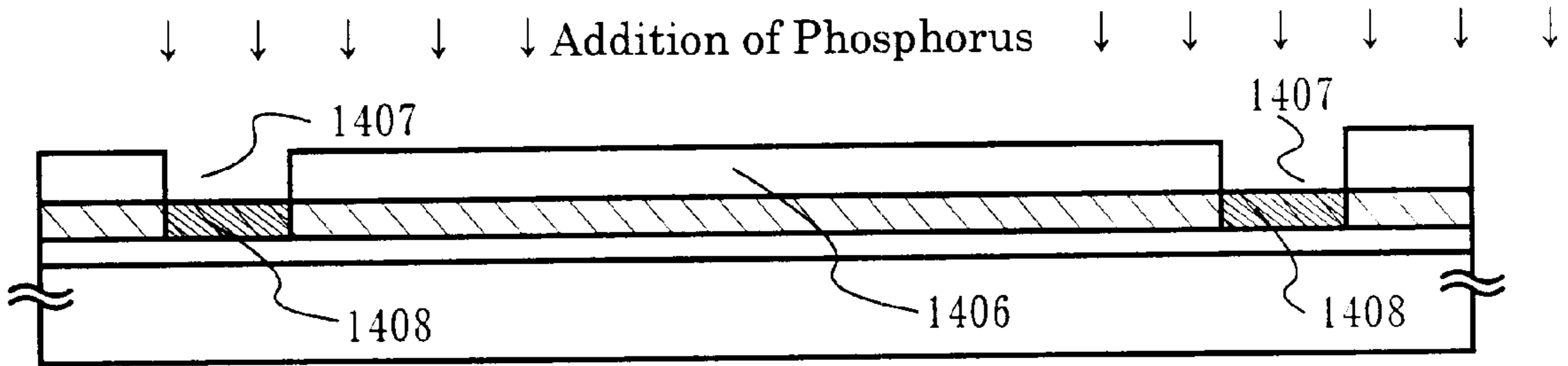
FIG. 14C
