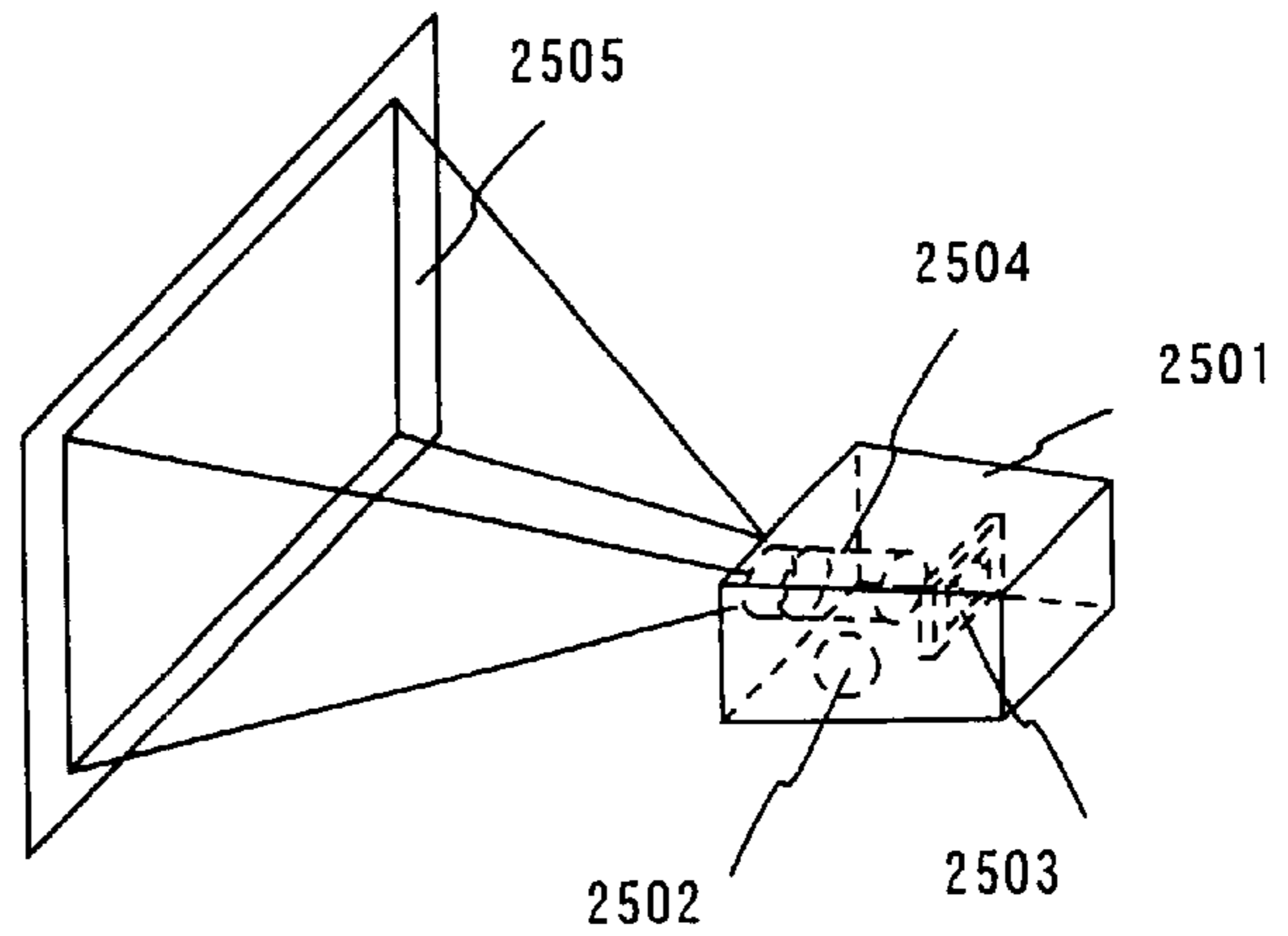
FIG. 30F
