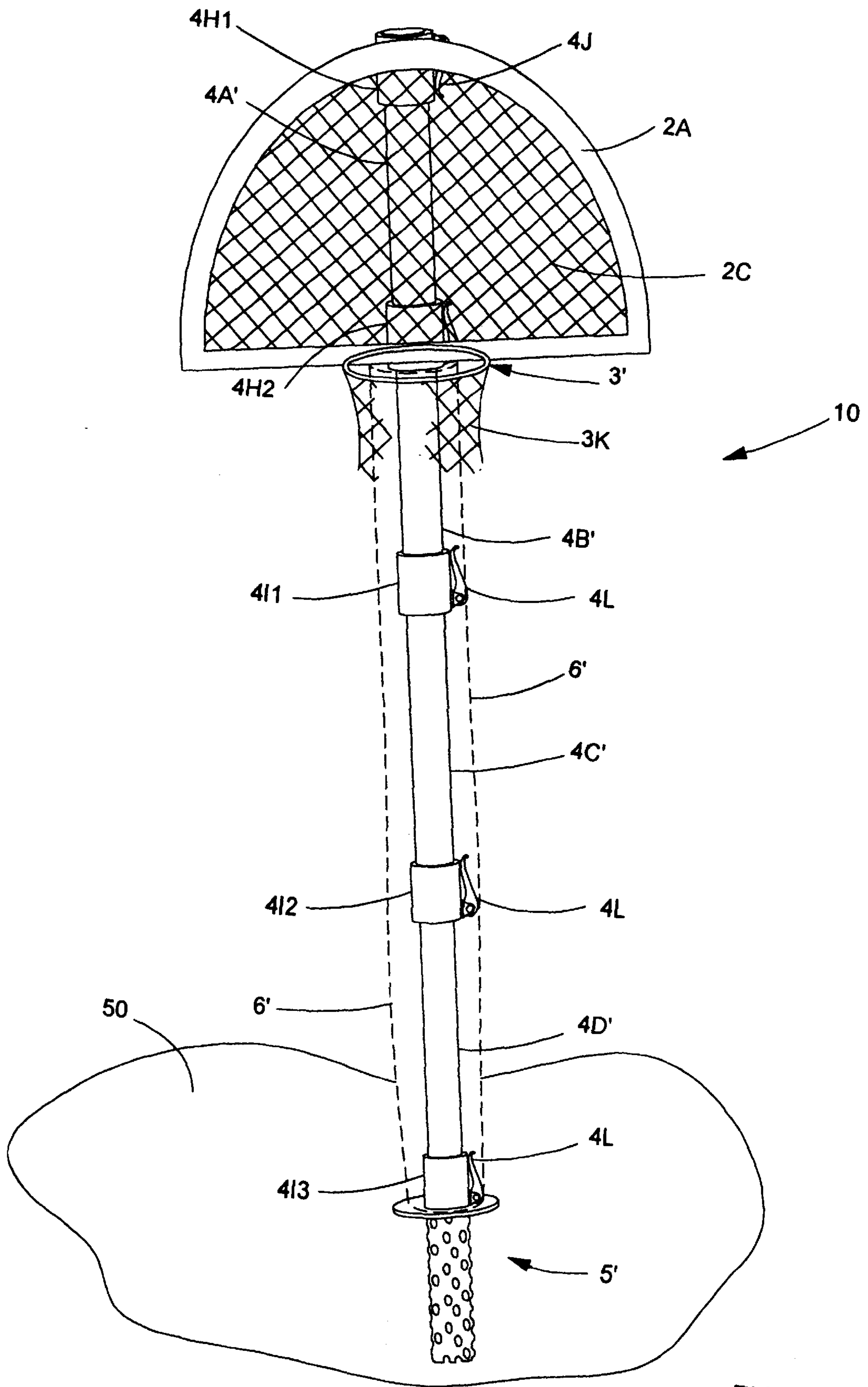
FIG. 3A
