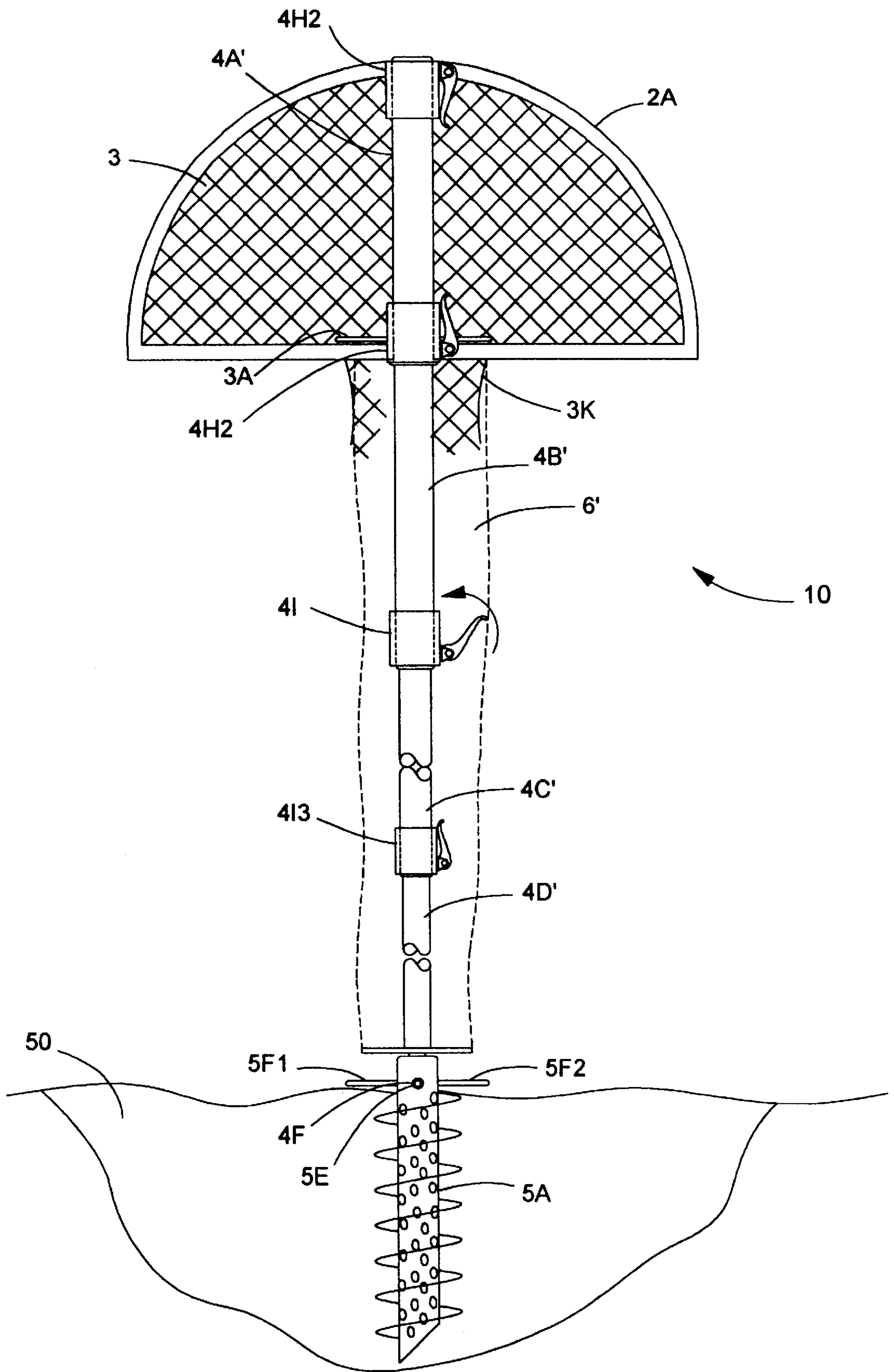
FIG. 3B
