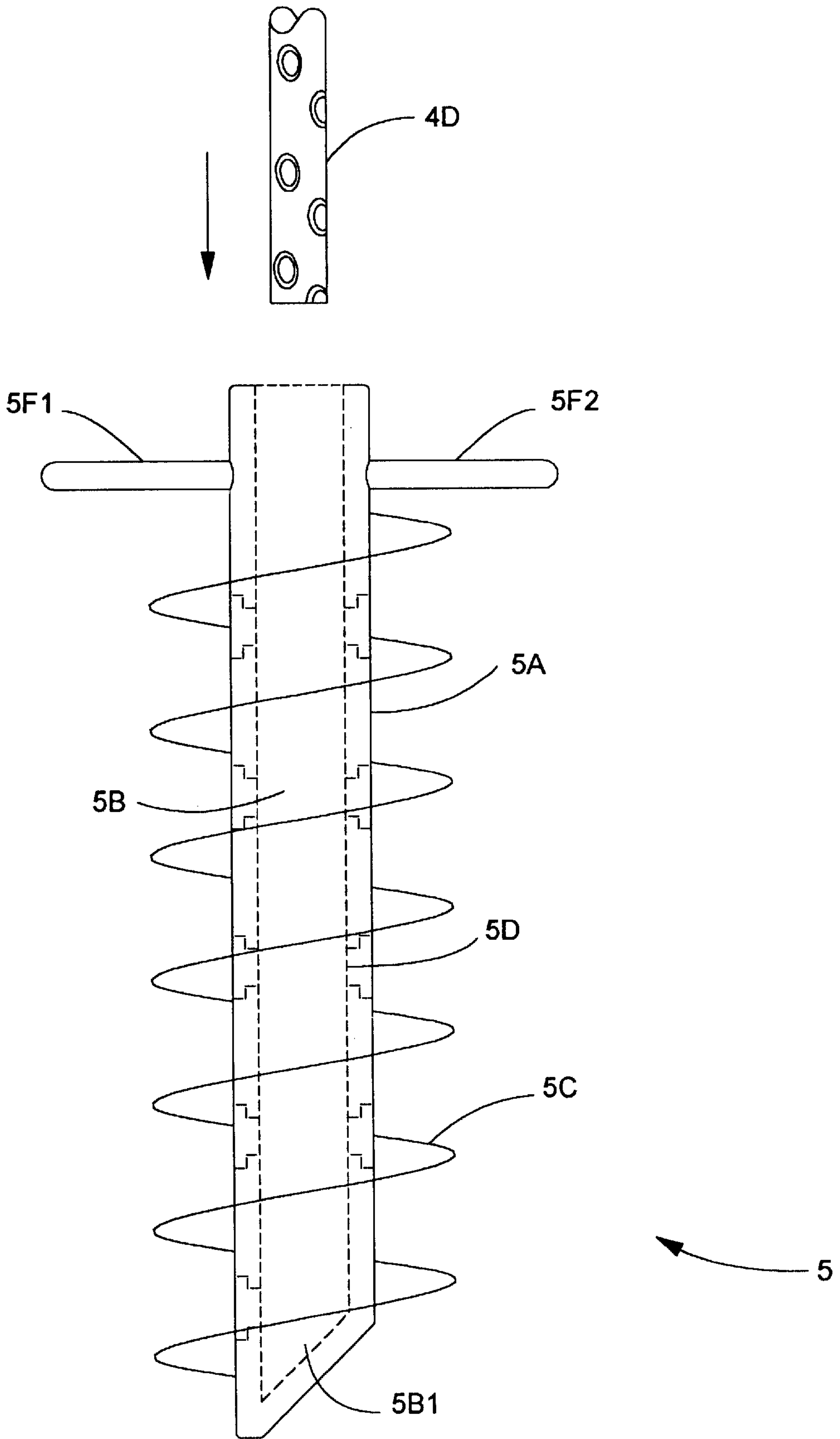
FIG. 2B2
