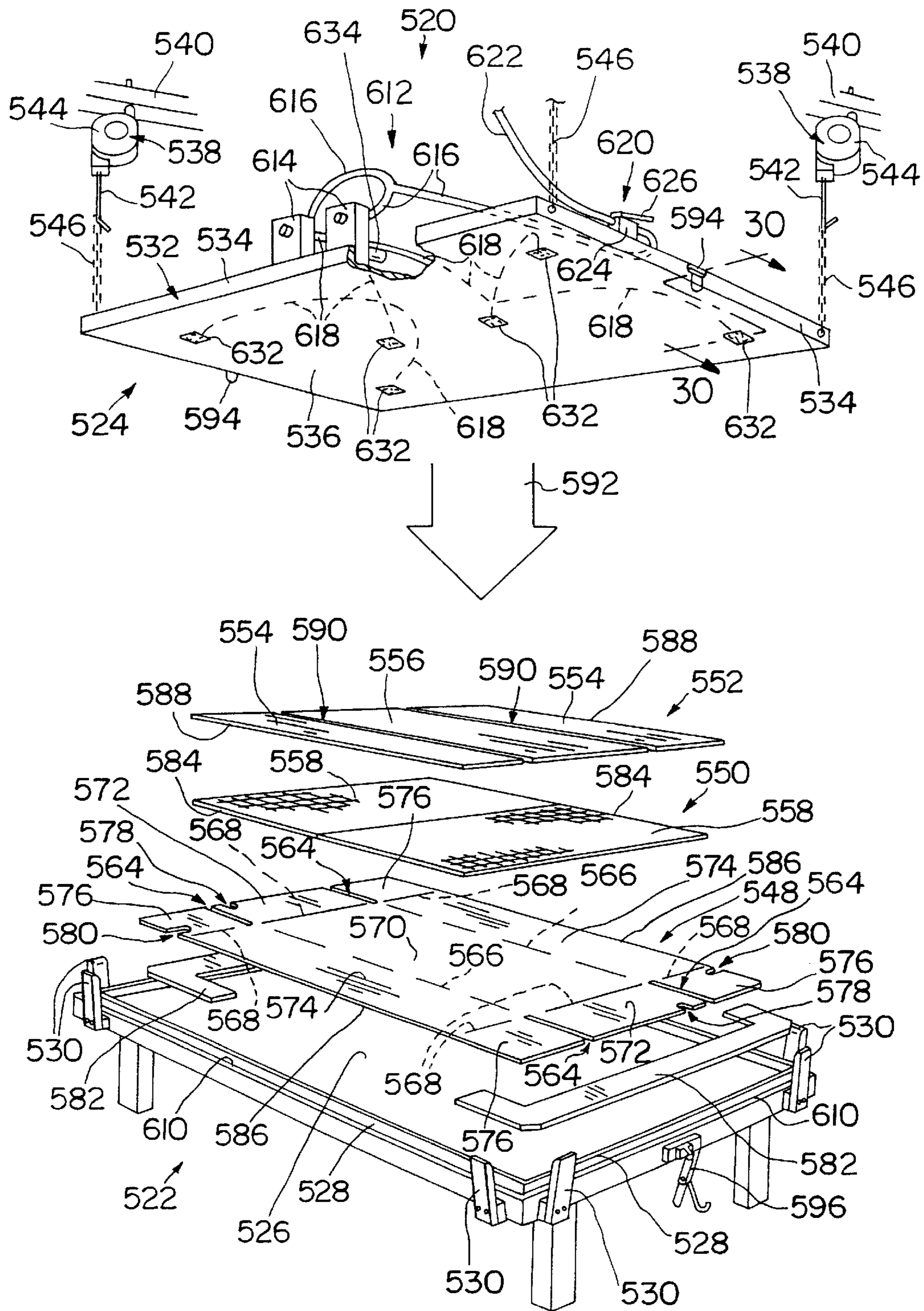
FIG. 29
