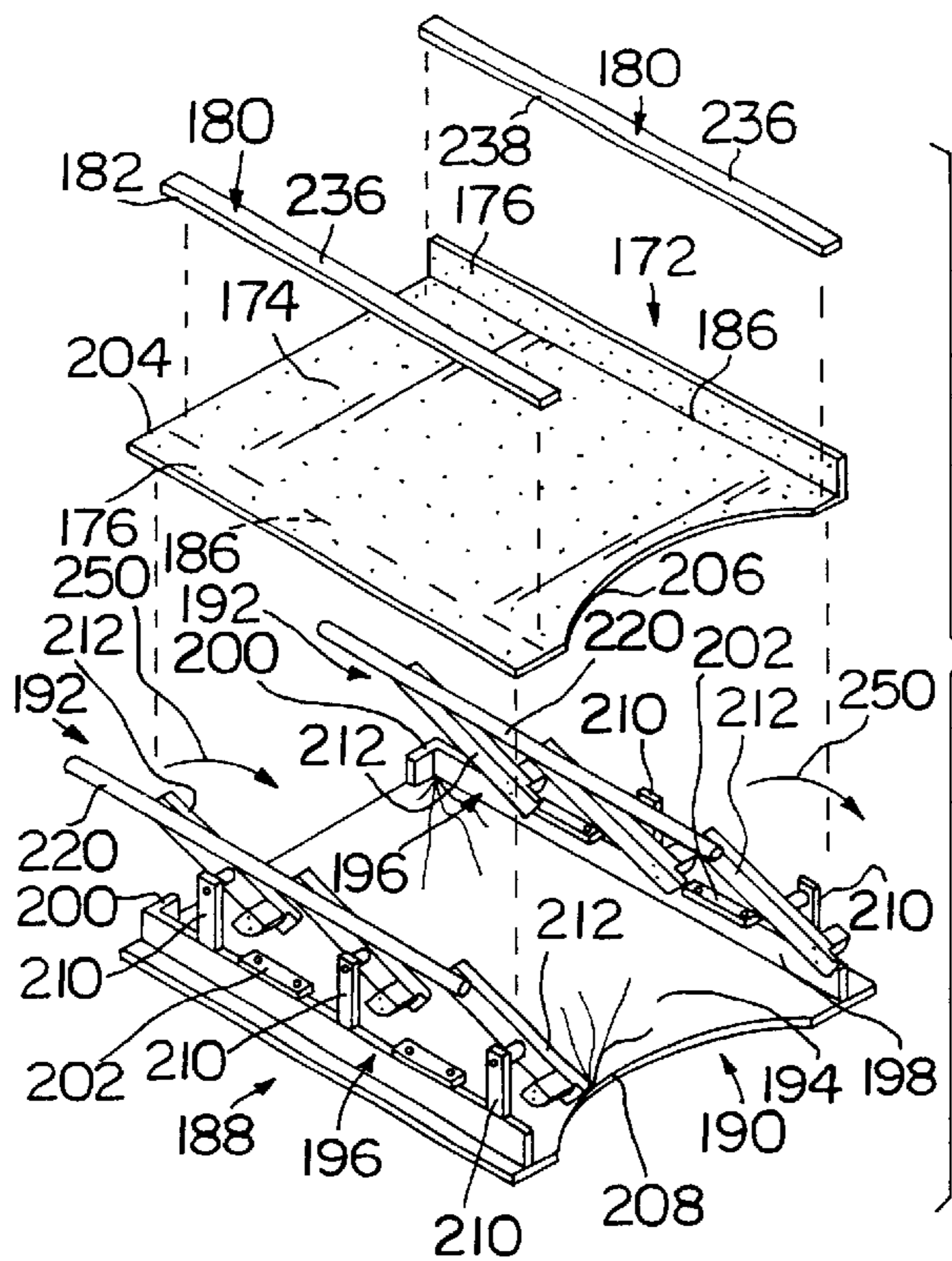
FIG. 12
