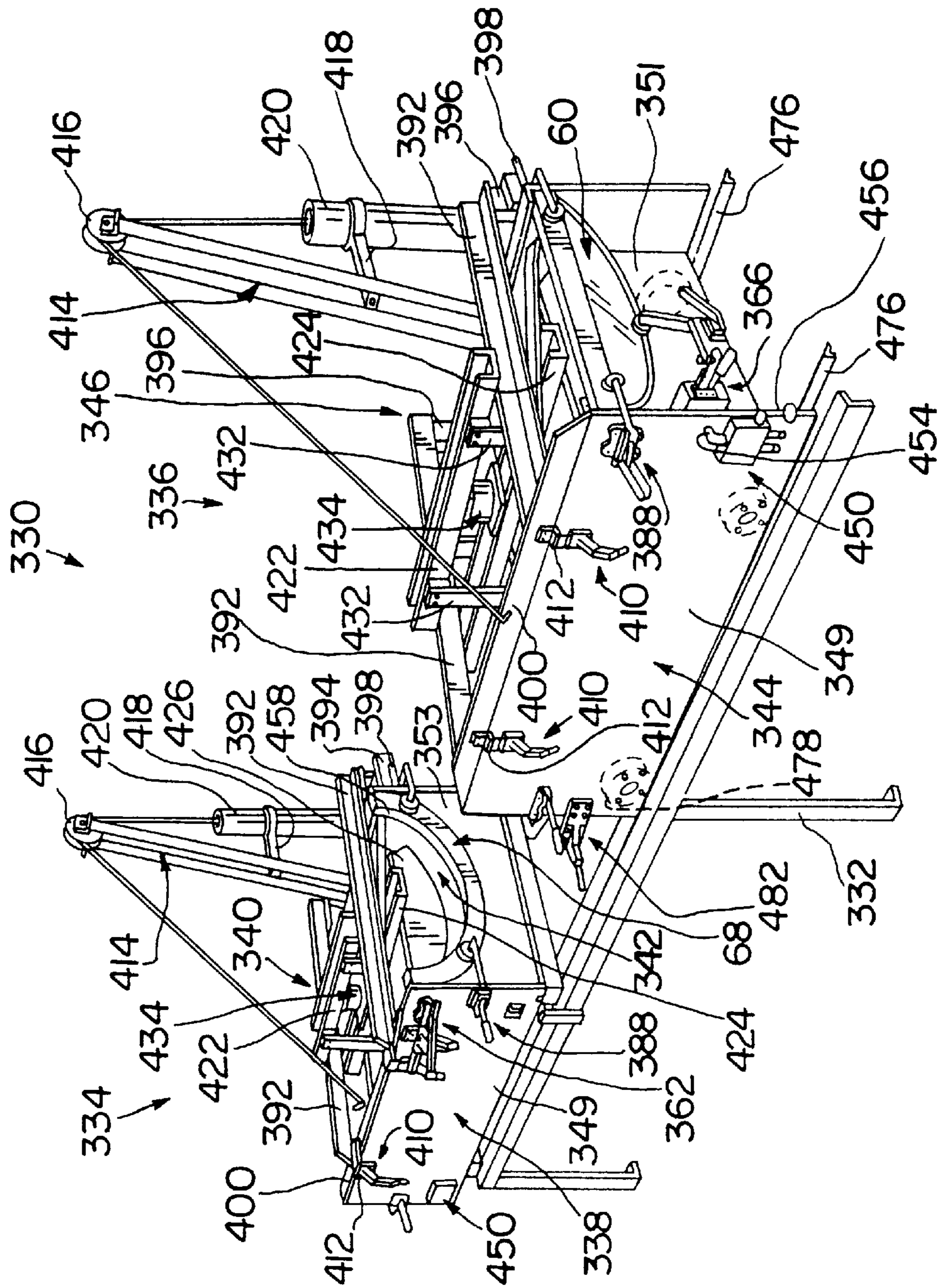
FIG. 21
