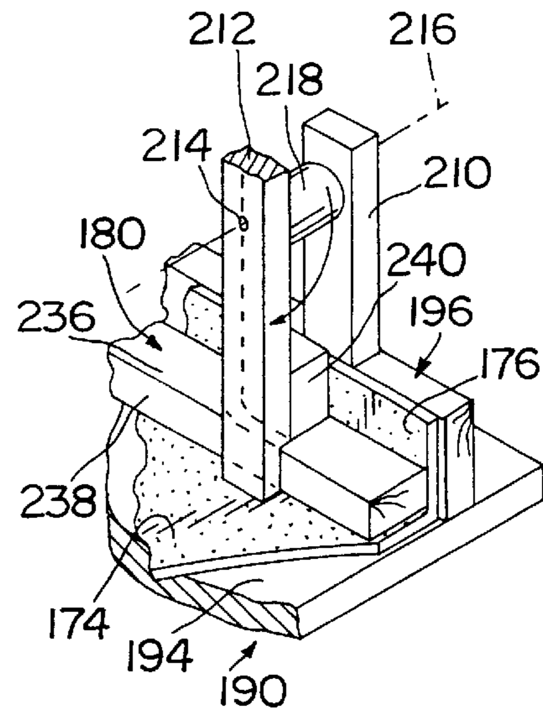
FIG. 14
