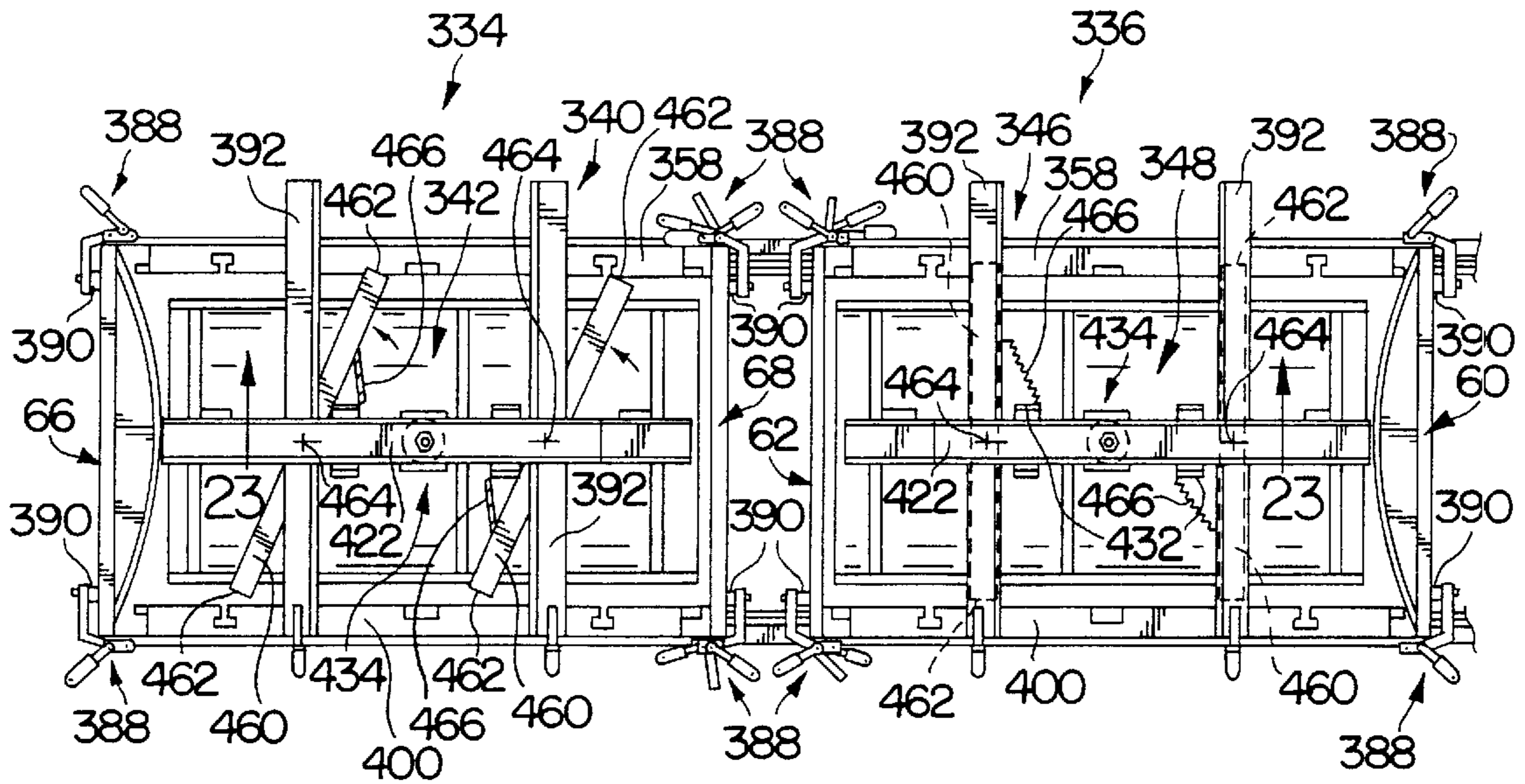
FIG. 22
