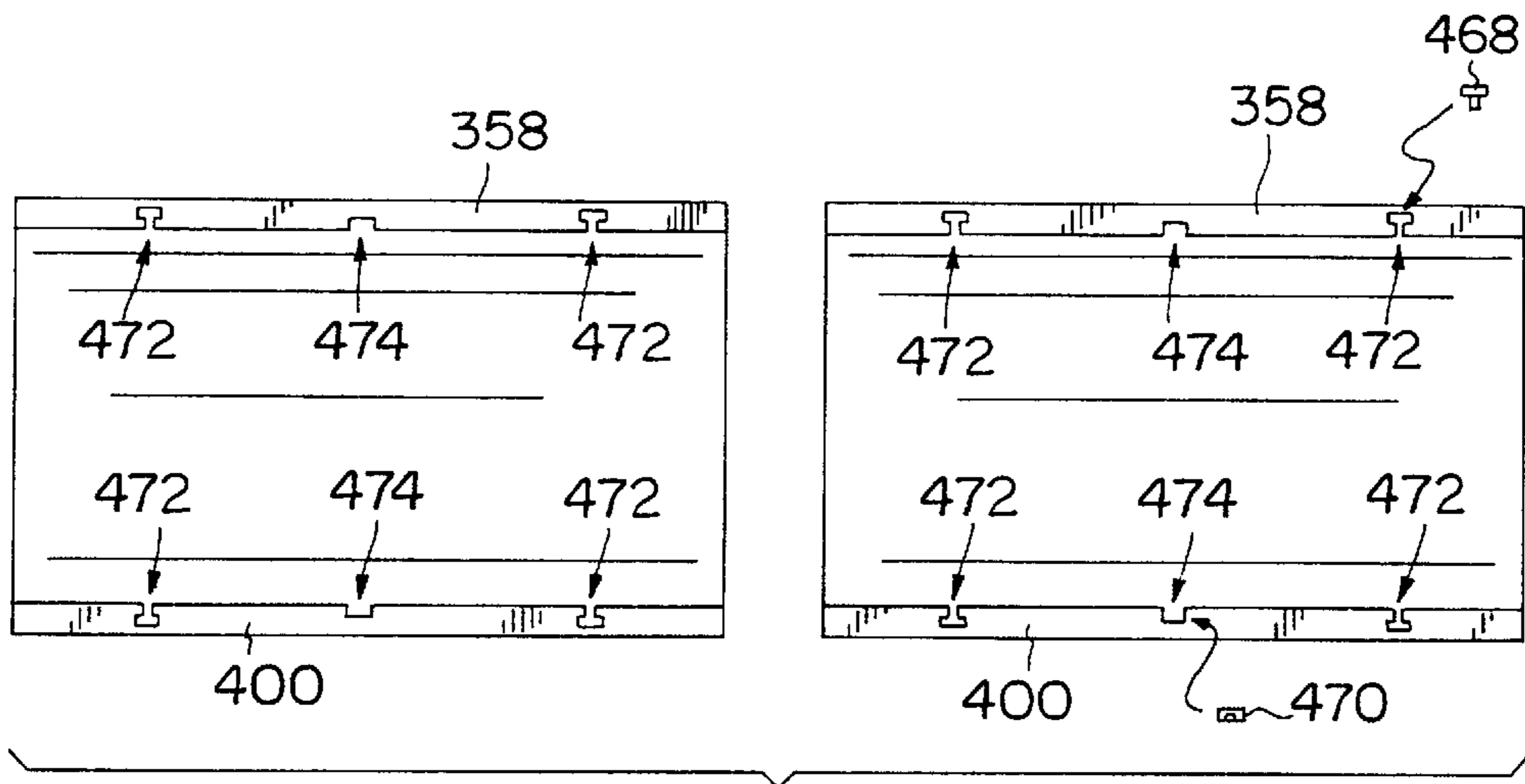
FIG. 24
