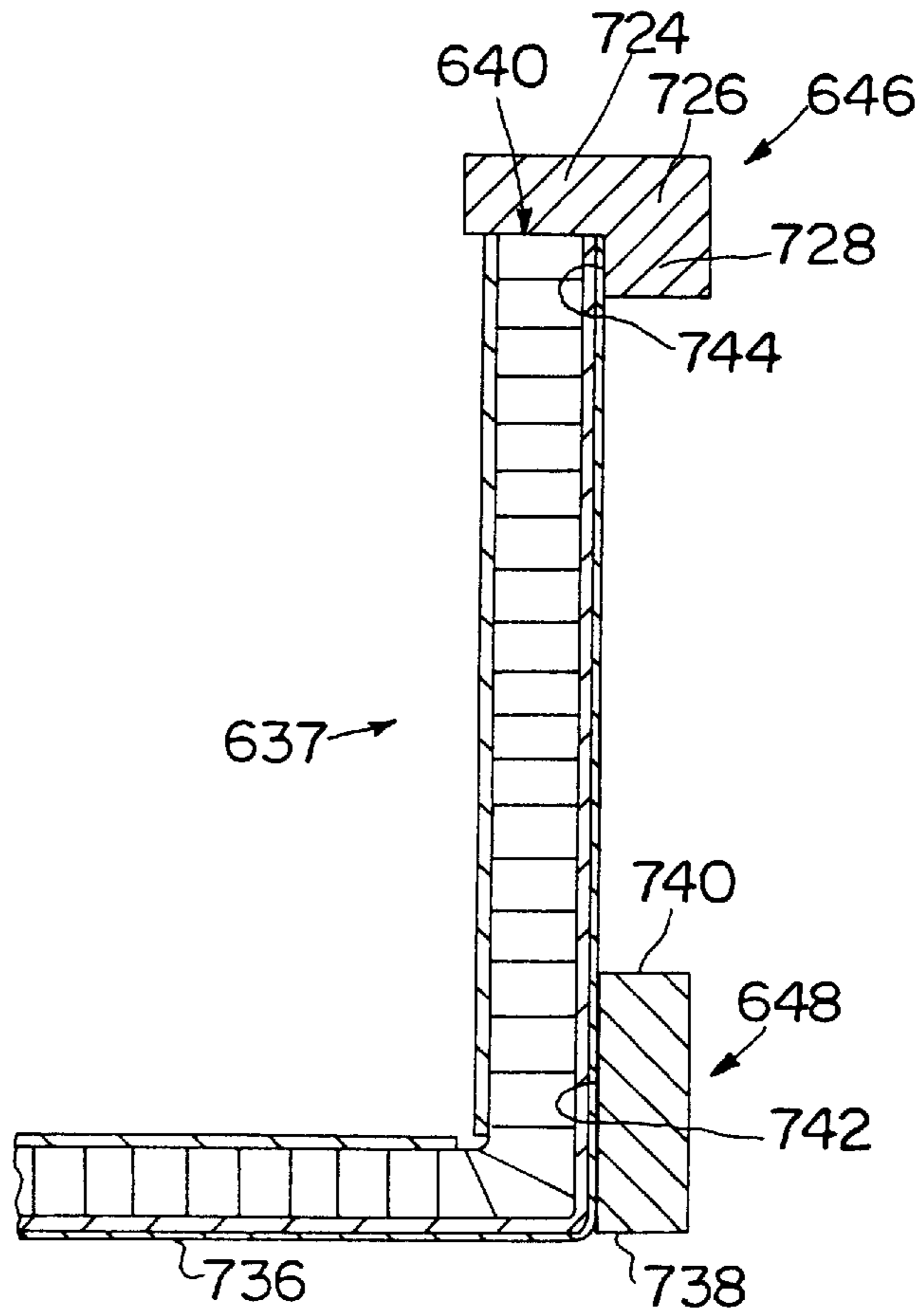
FIG. 37
