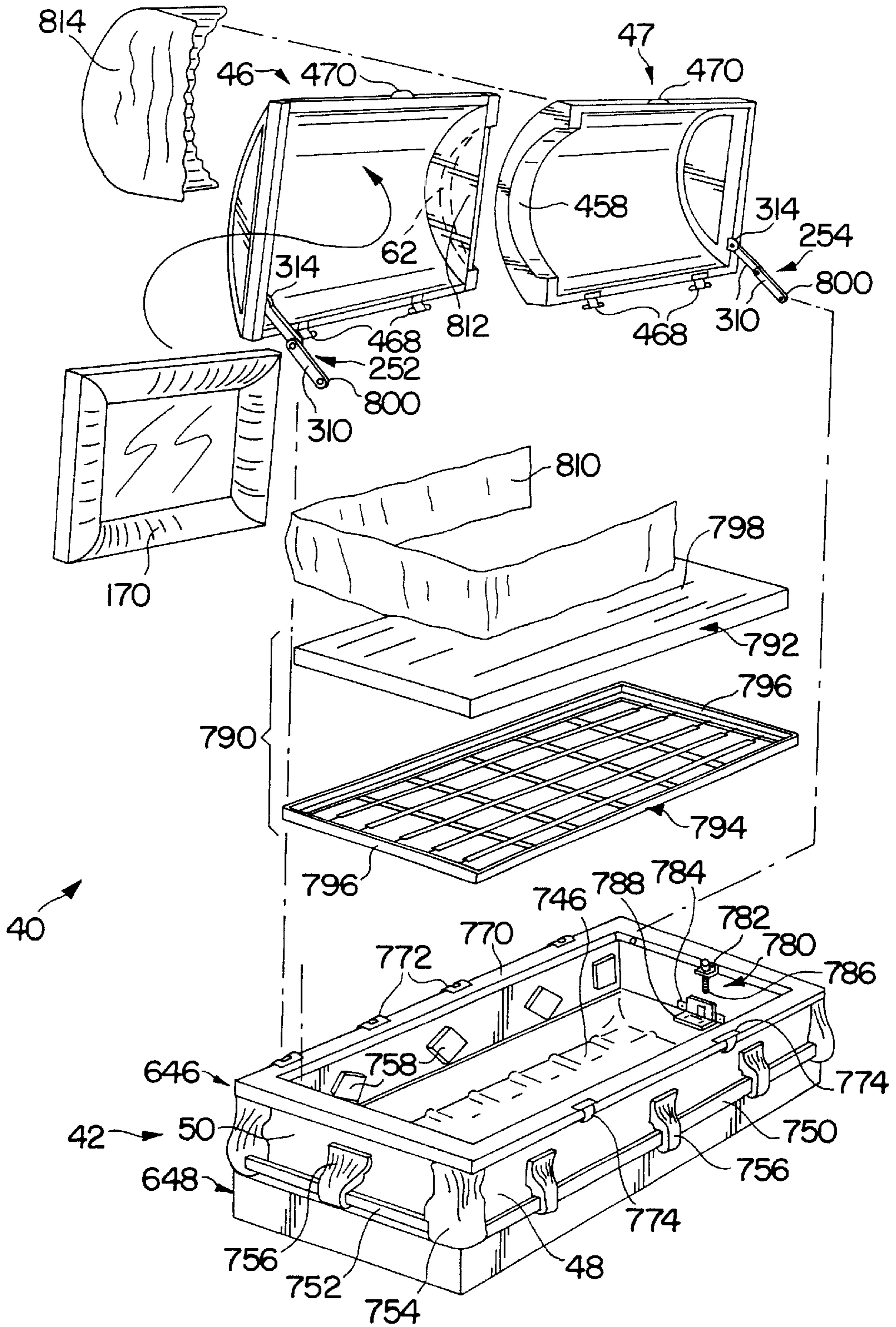
FIG. 39
