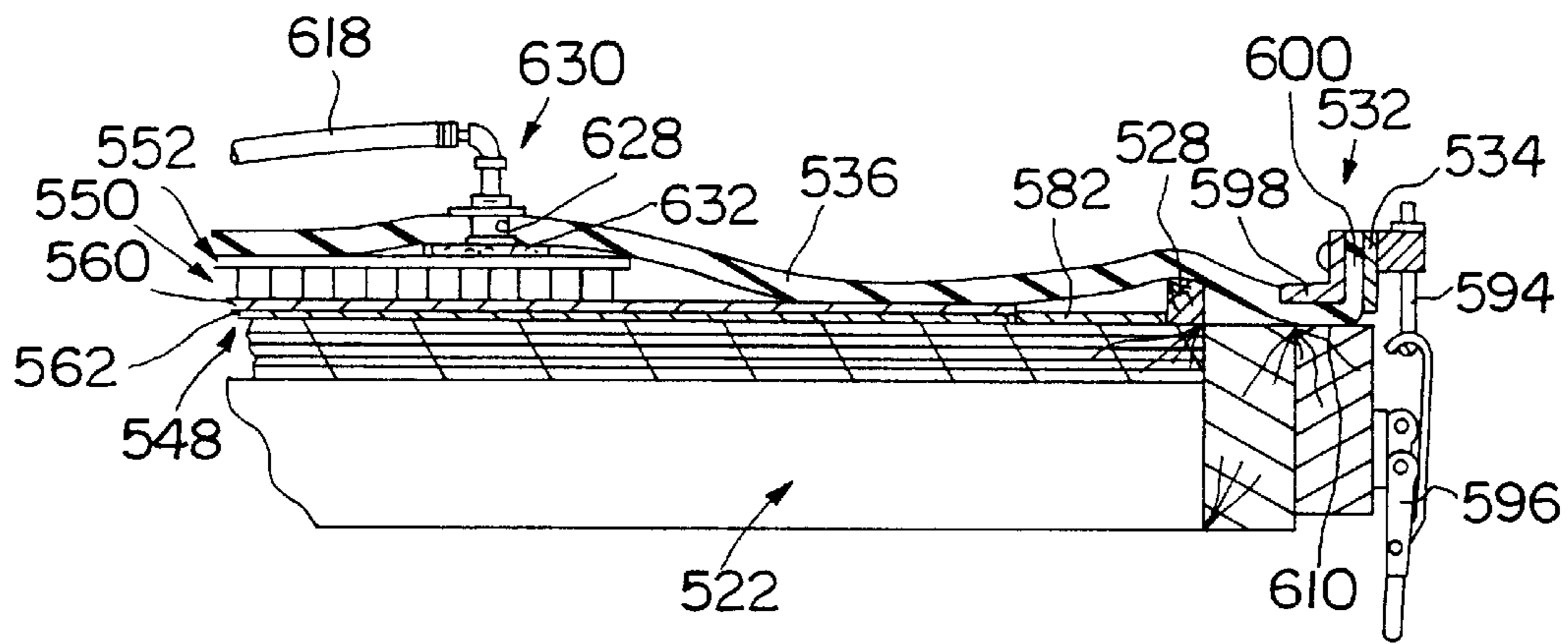
FIG. 30
