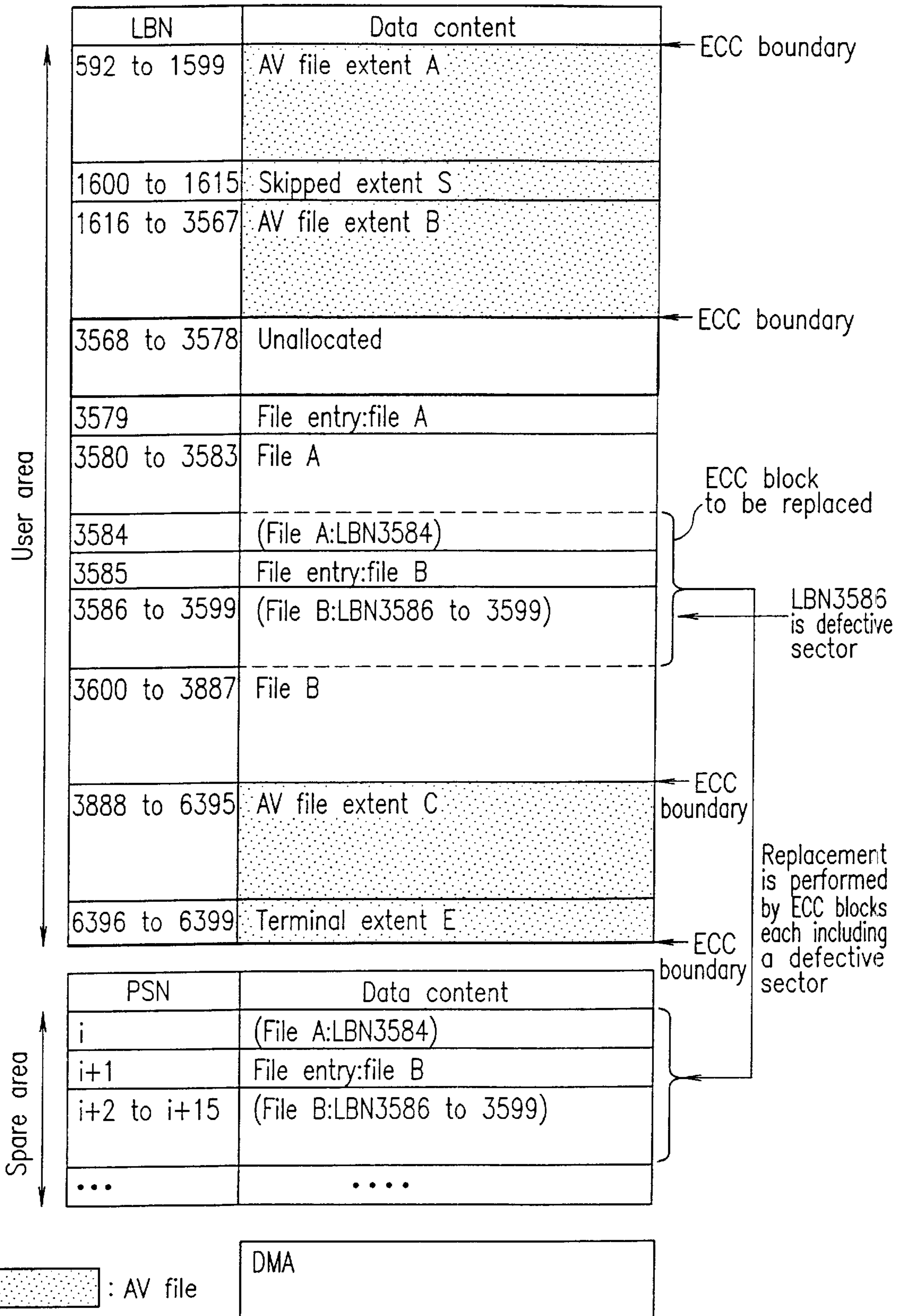
FIG. 12
