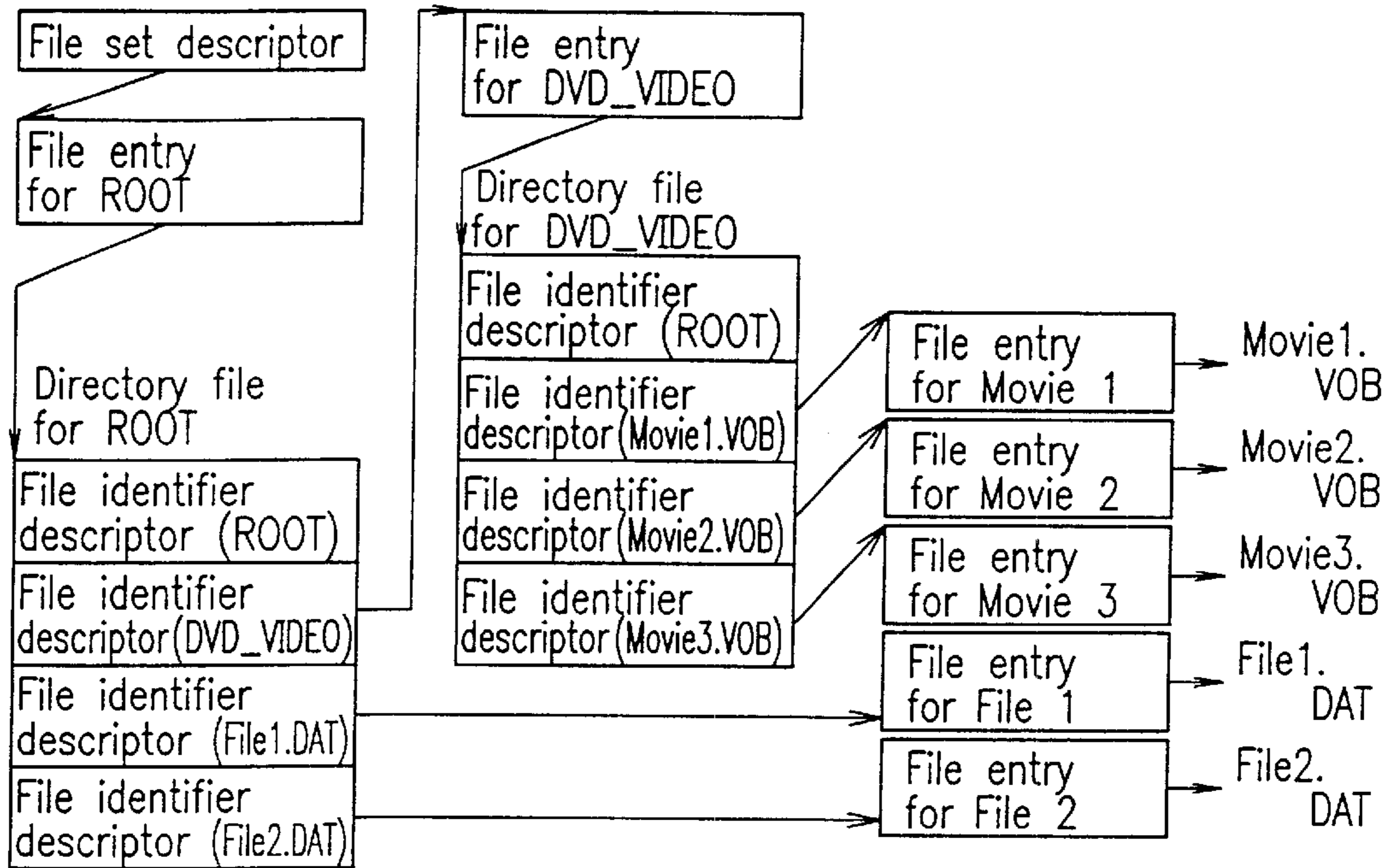
FIG. 23
