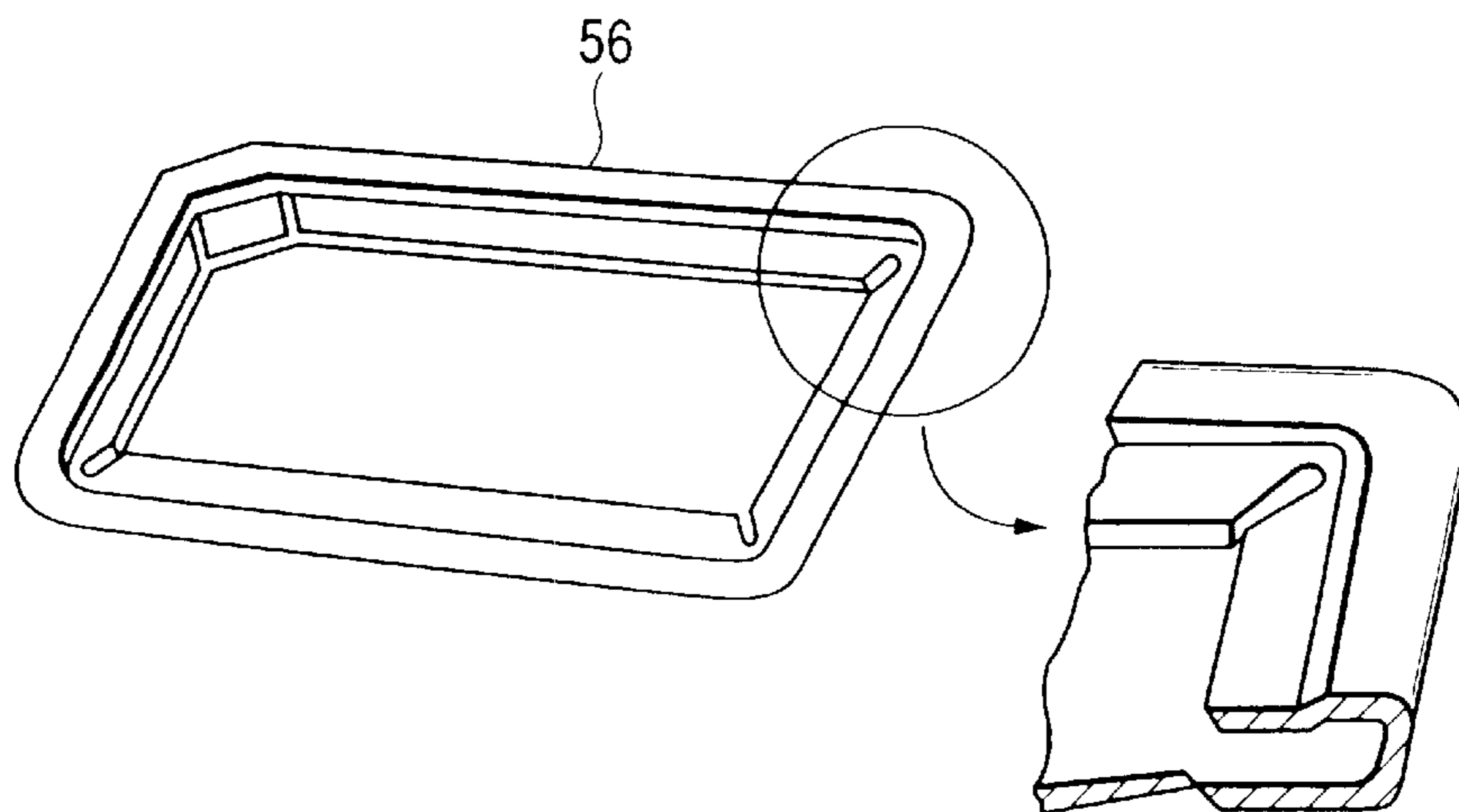
FIG. 25(D)
