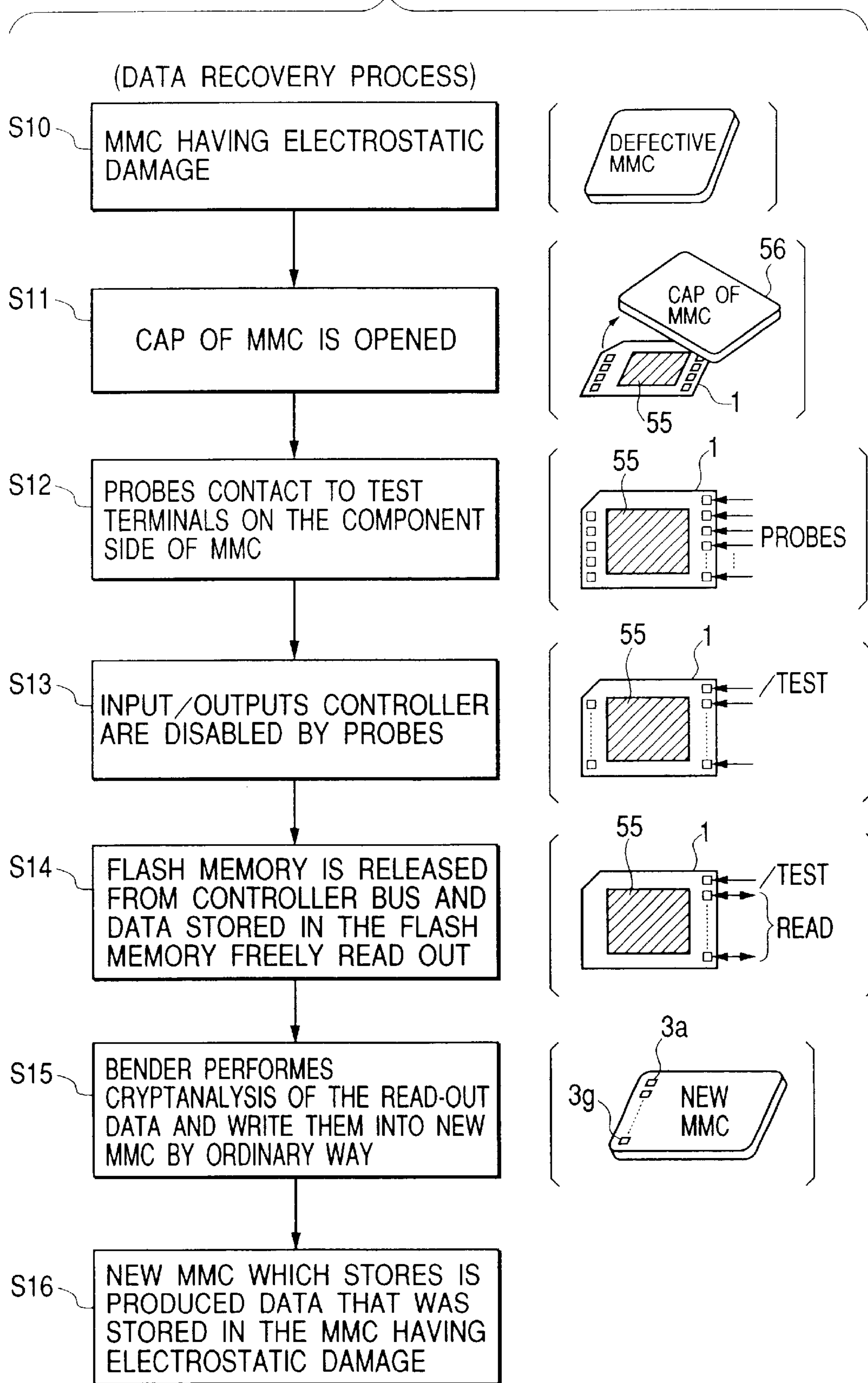
FIG. 24
