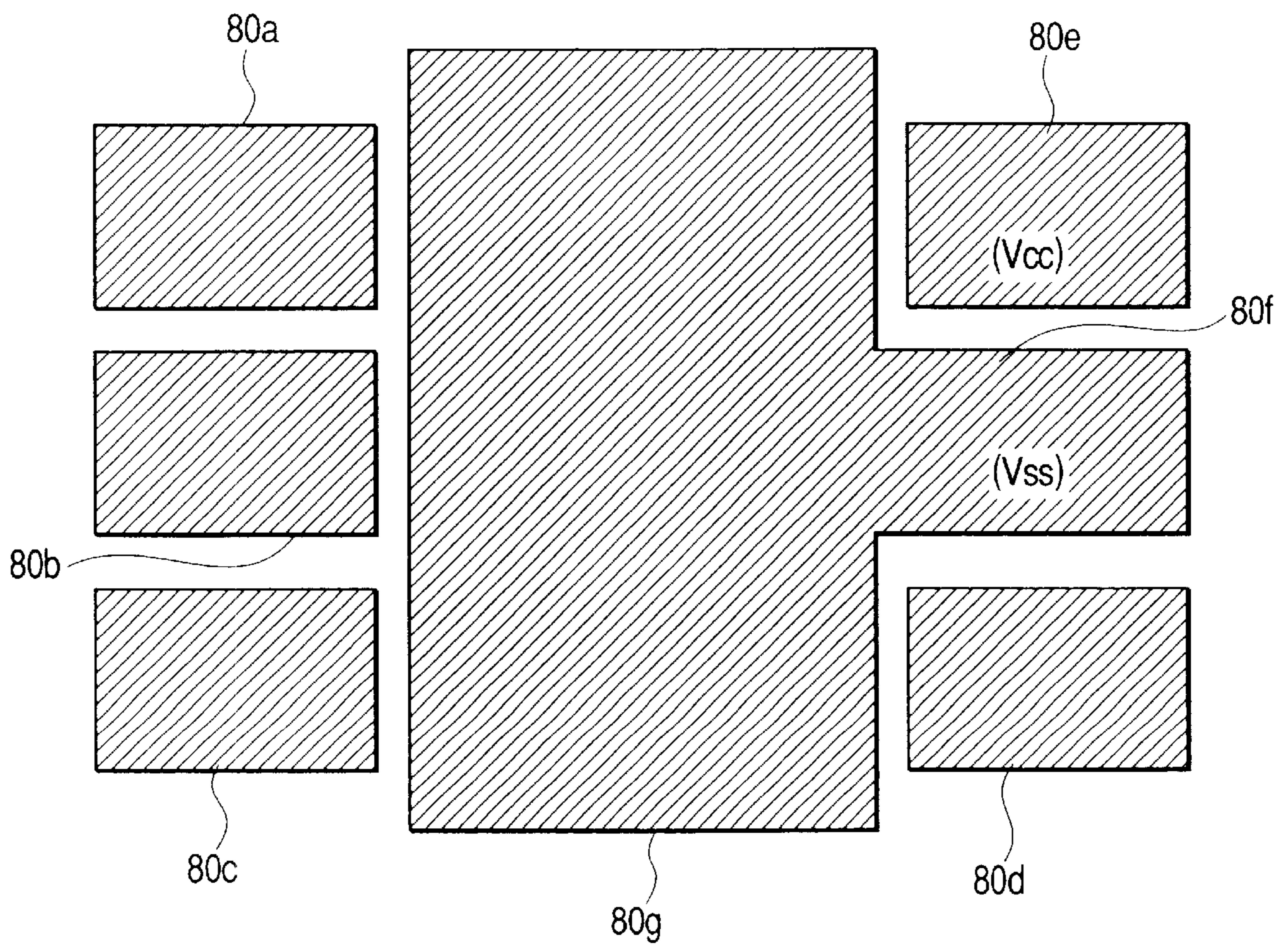
FIG. 20
