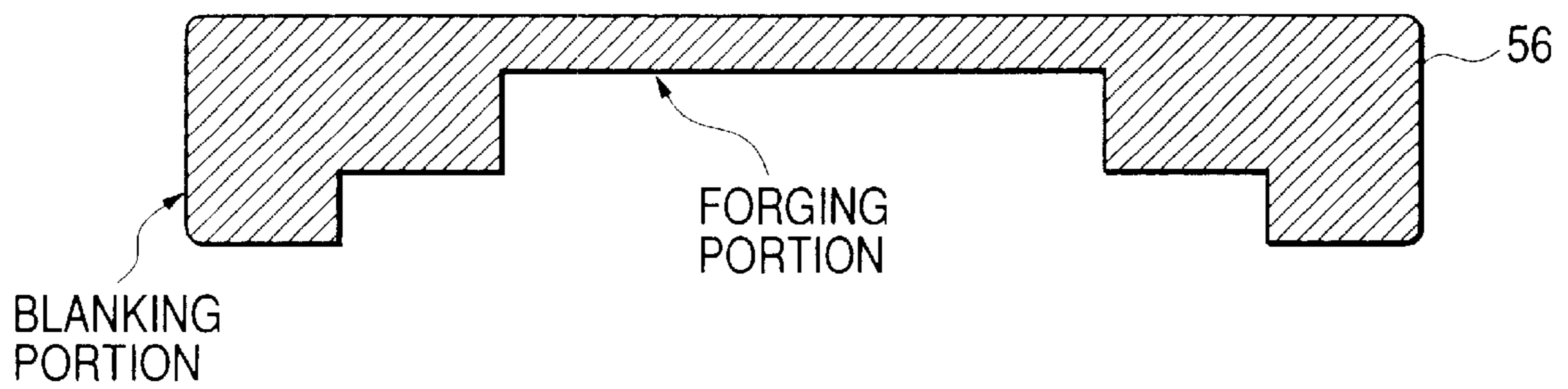
FIG. 25(B)
