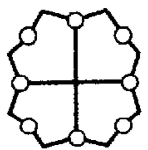
CHABAZITE
