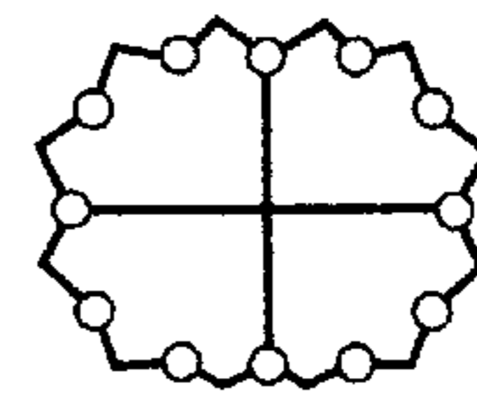
MORDENITE
