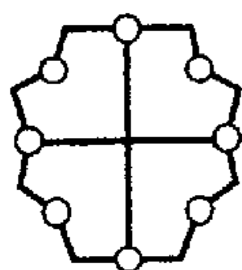
ERONITE
