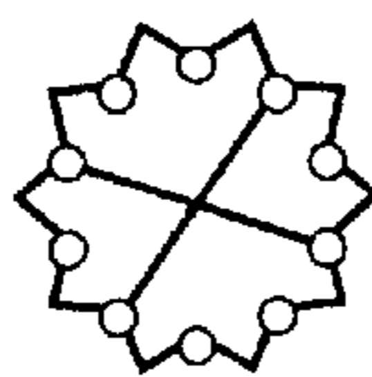
ZSM-5
