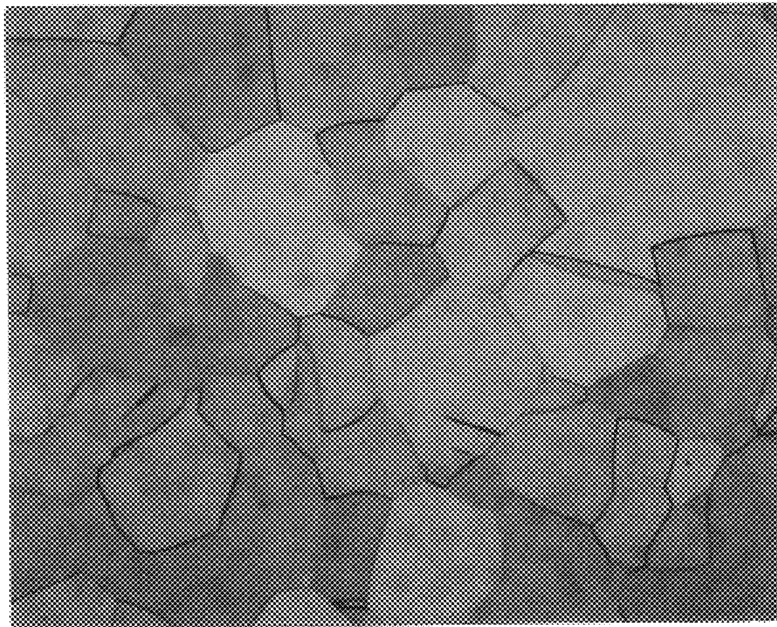
PURE Ti, ANNEALING T-RE 675° C, X200
