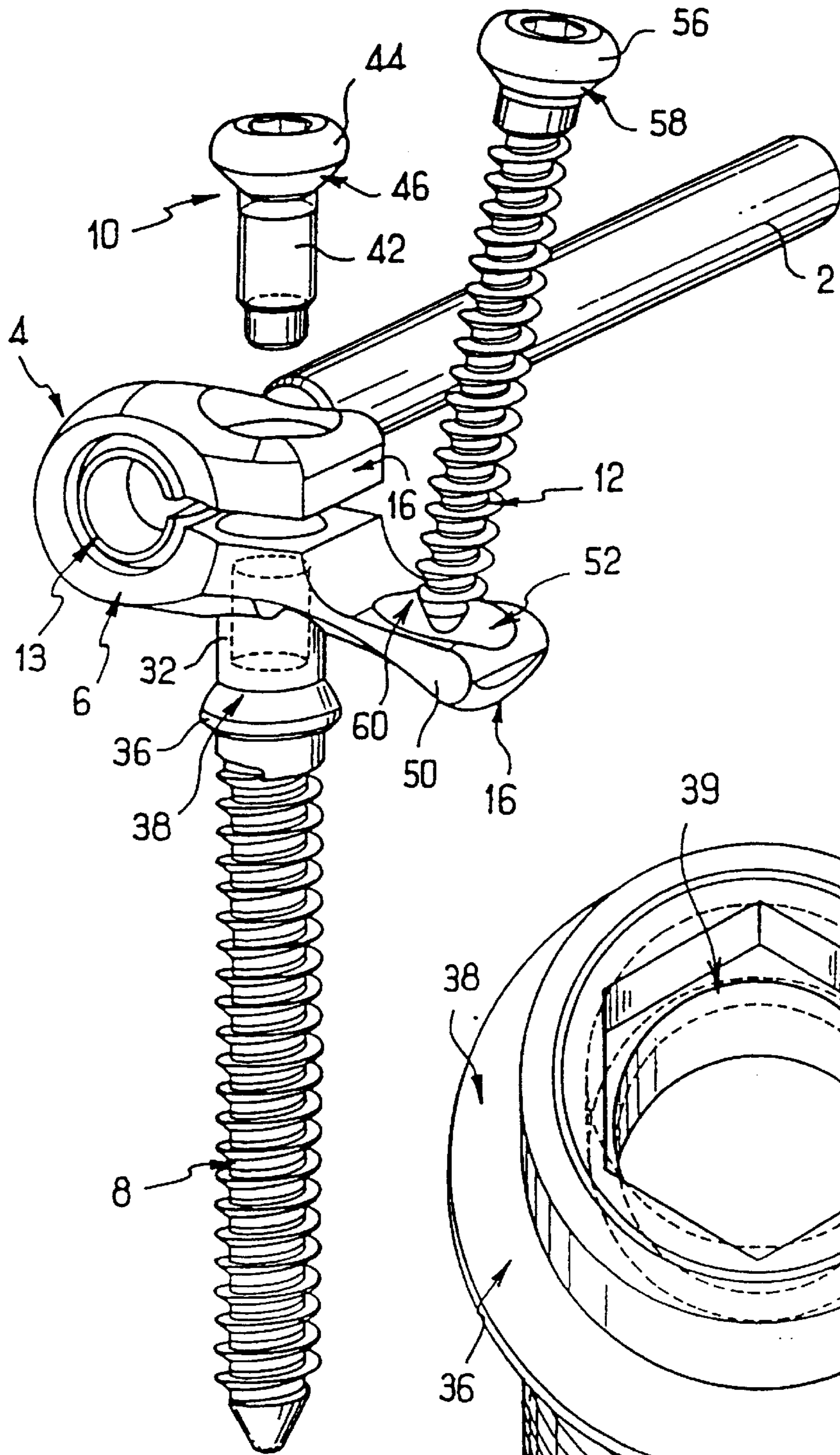
FIG. 7
