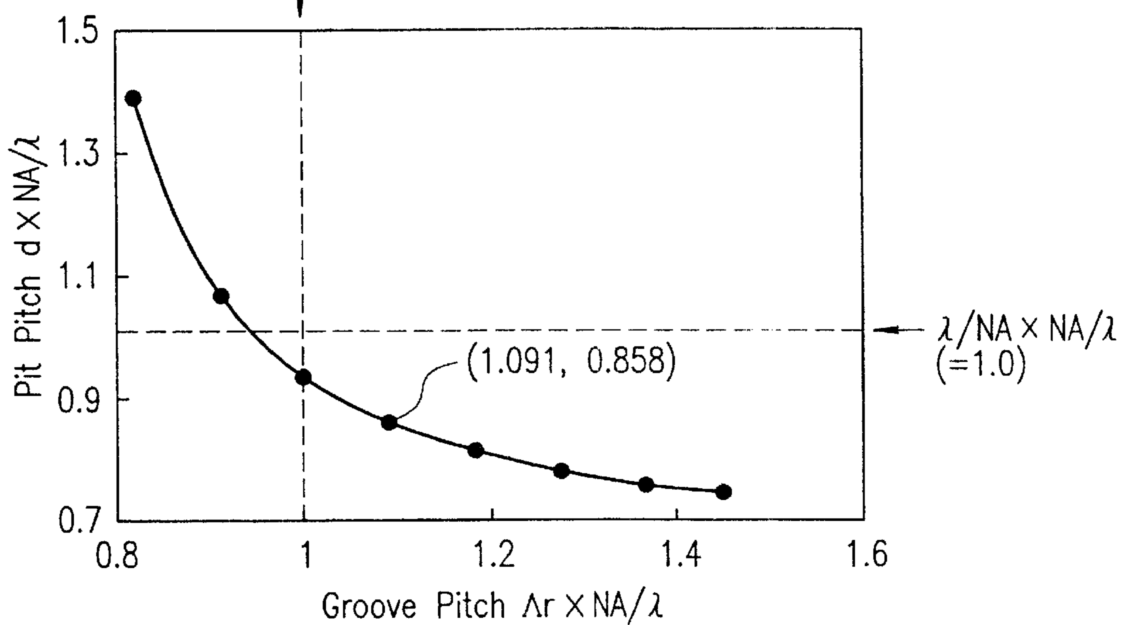
FIG. 6 \lambda/NA \times NA/\lambda (=1.0)
