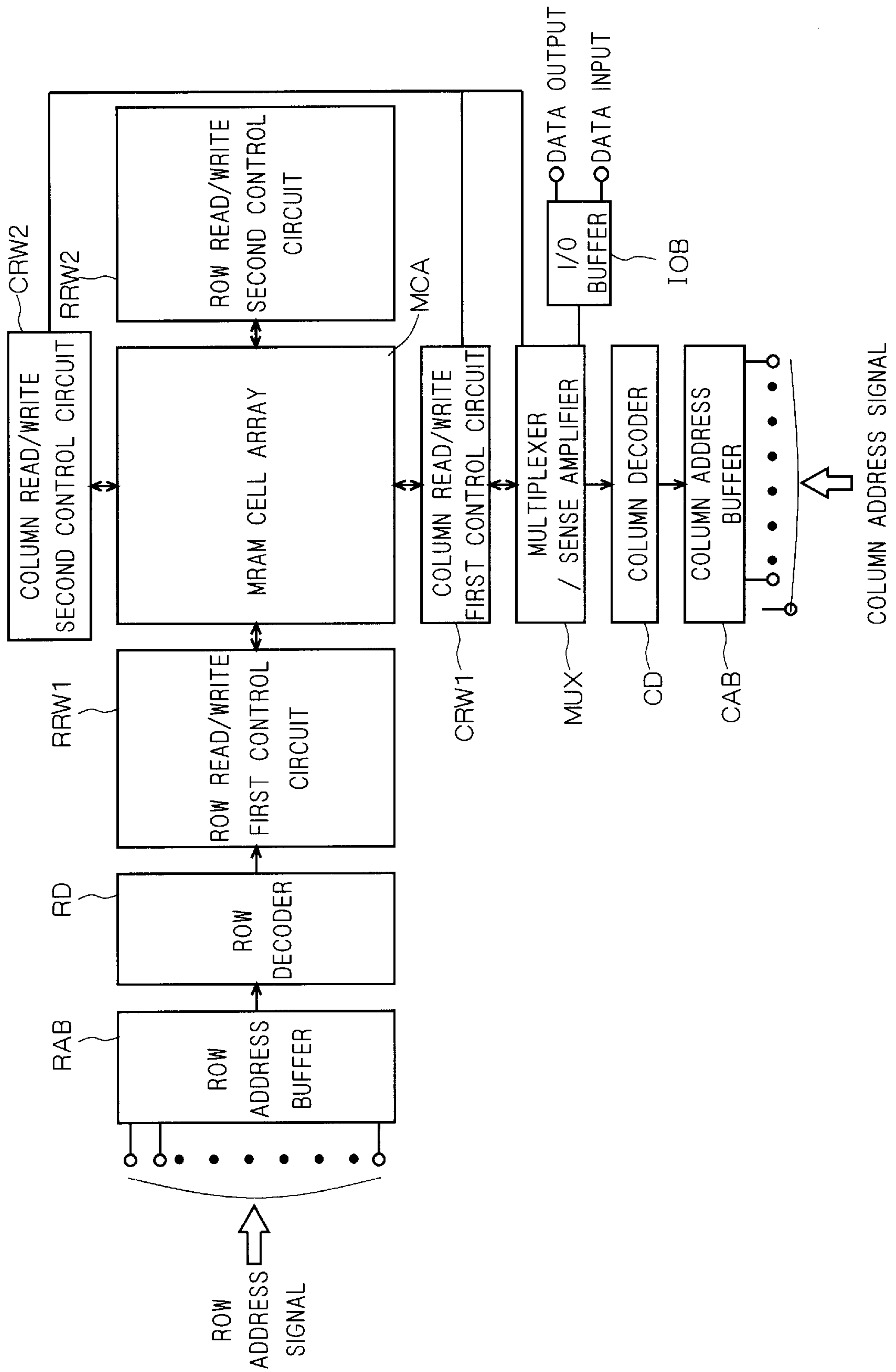
FIG. 26
