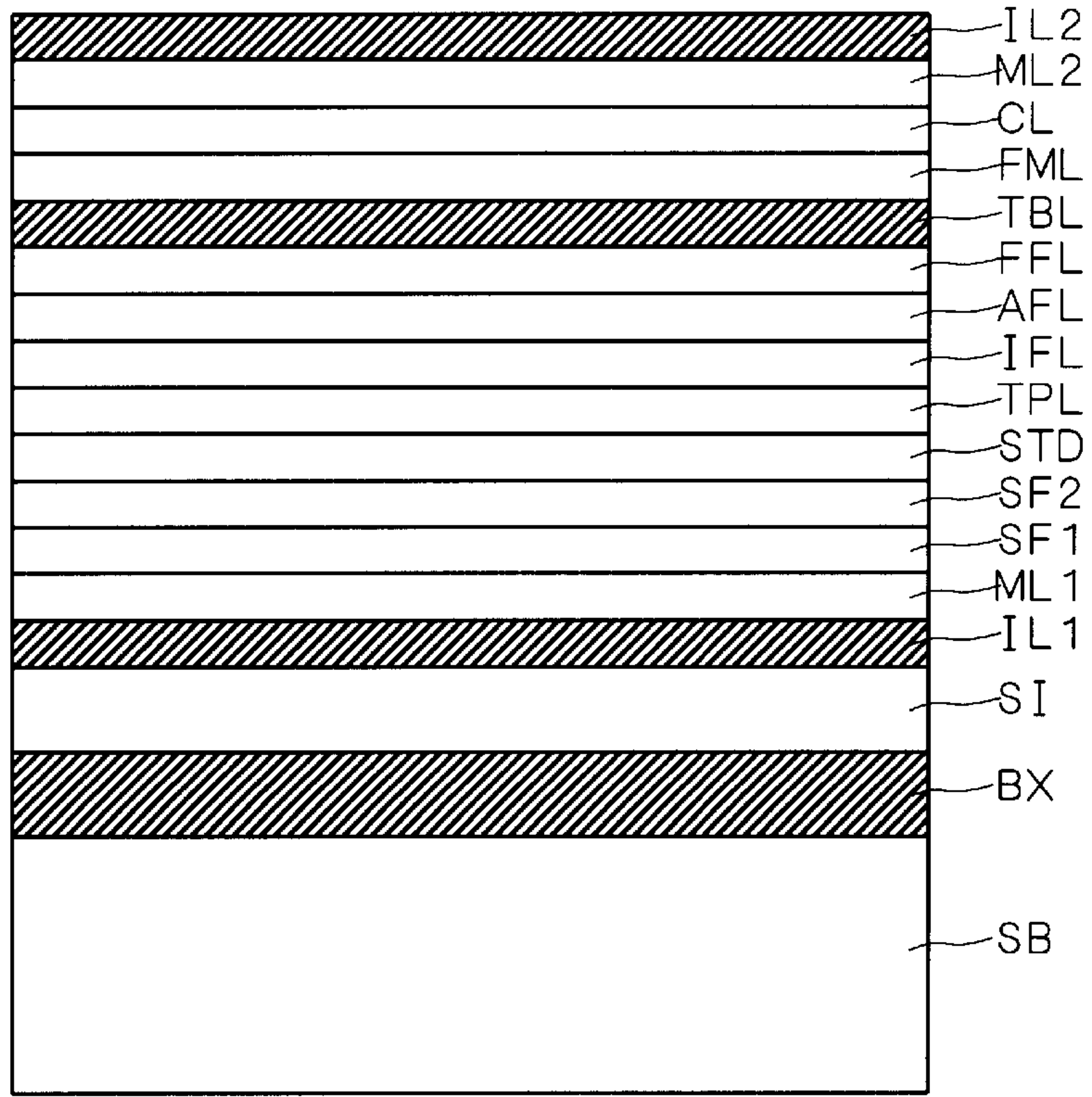
FIG. 50
