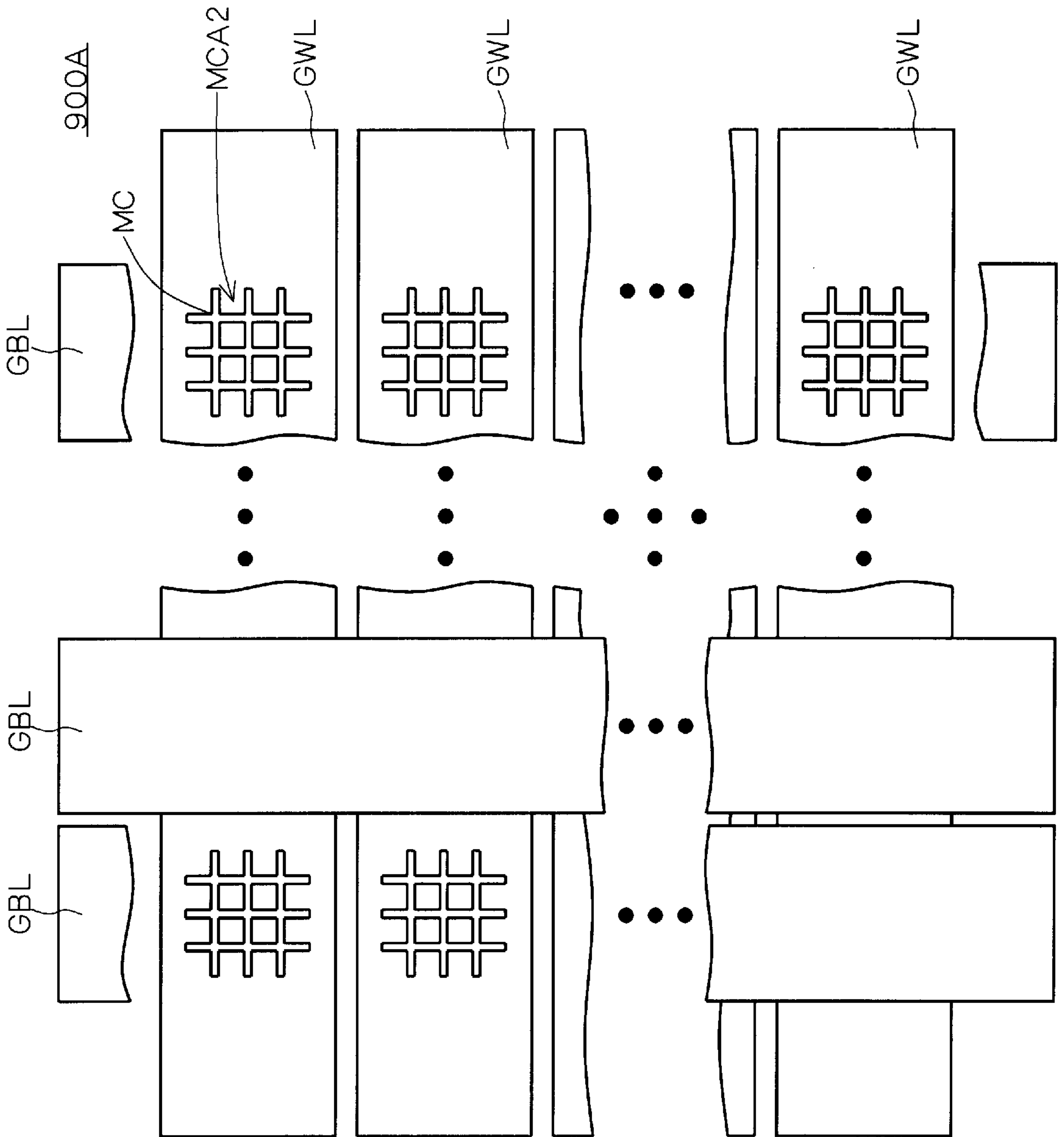
FIG. 46
