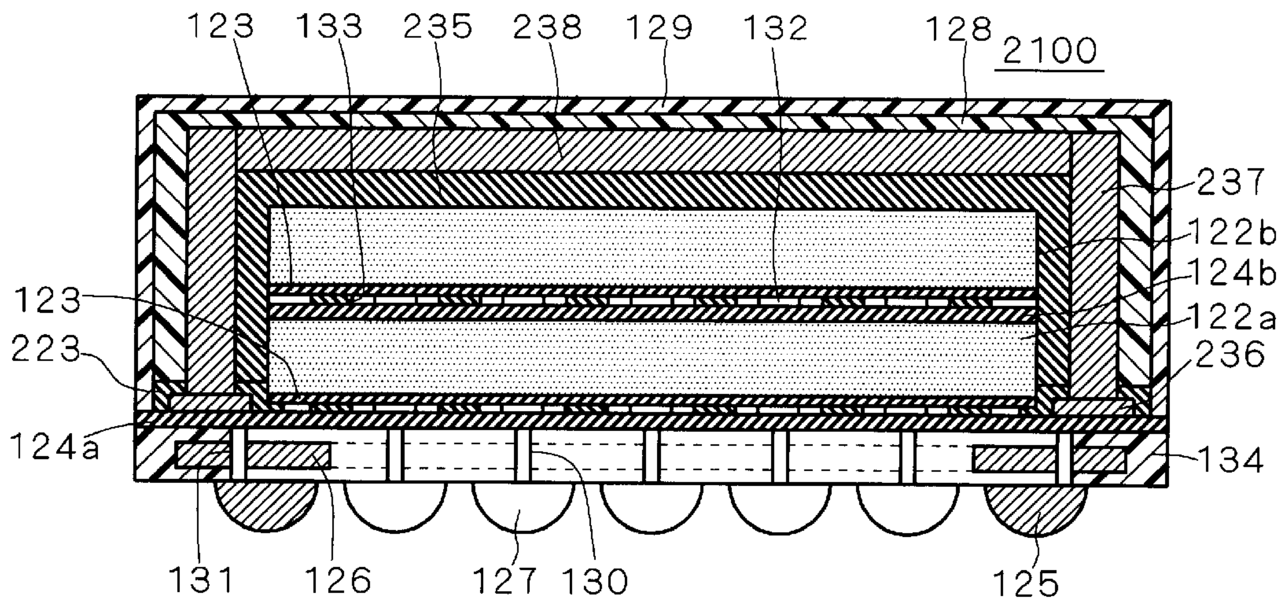
FIG. 66
