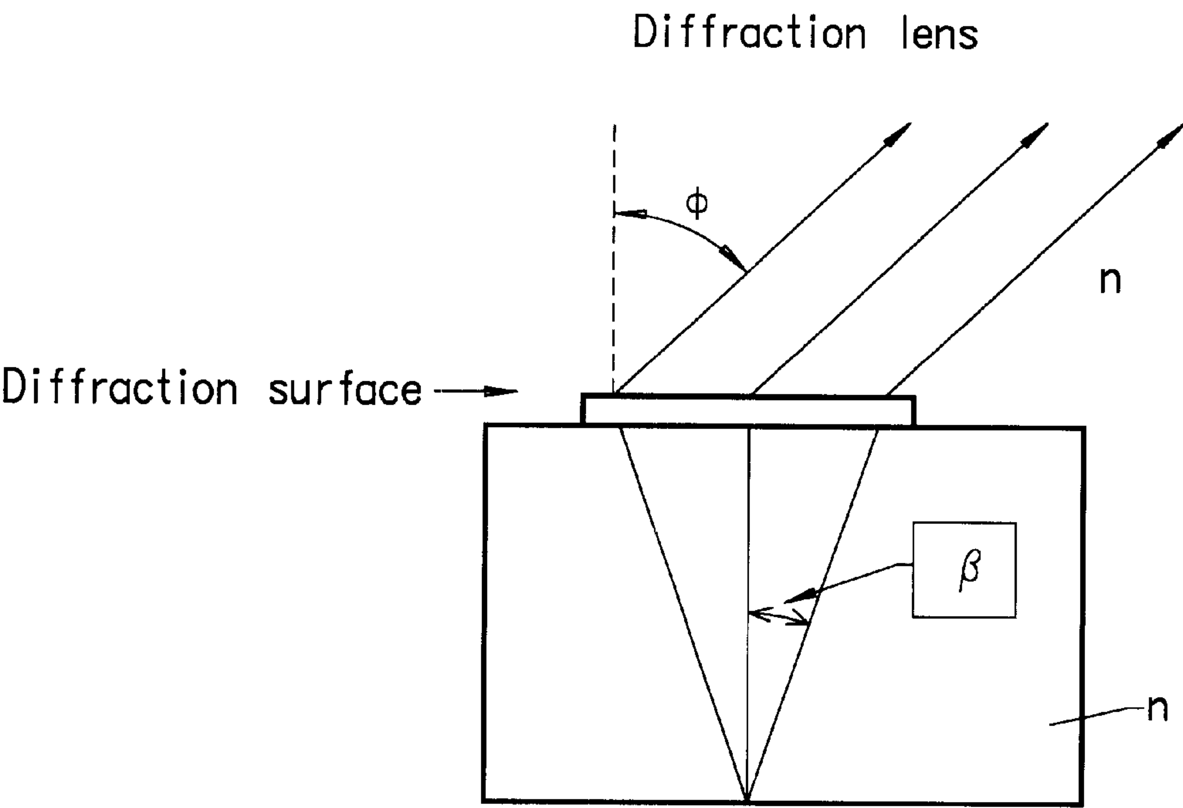
FIG. 4B
