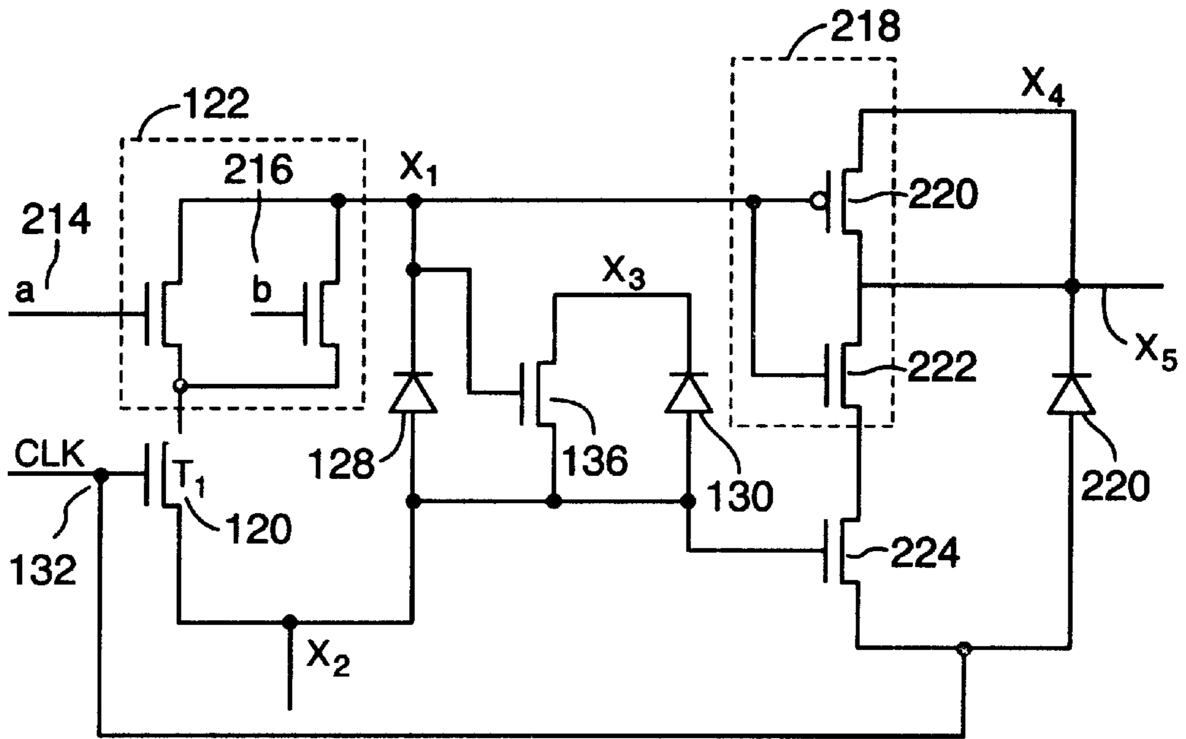
FIG. 7C OR-2 GATE
