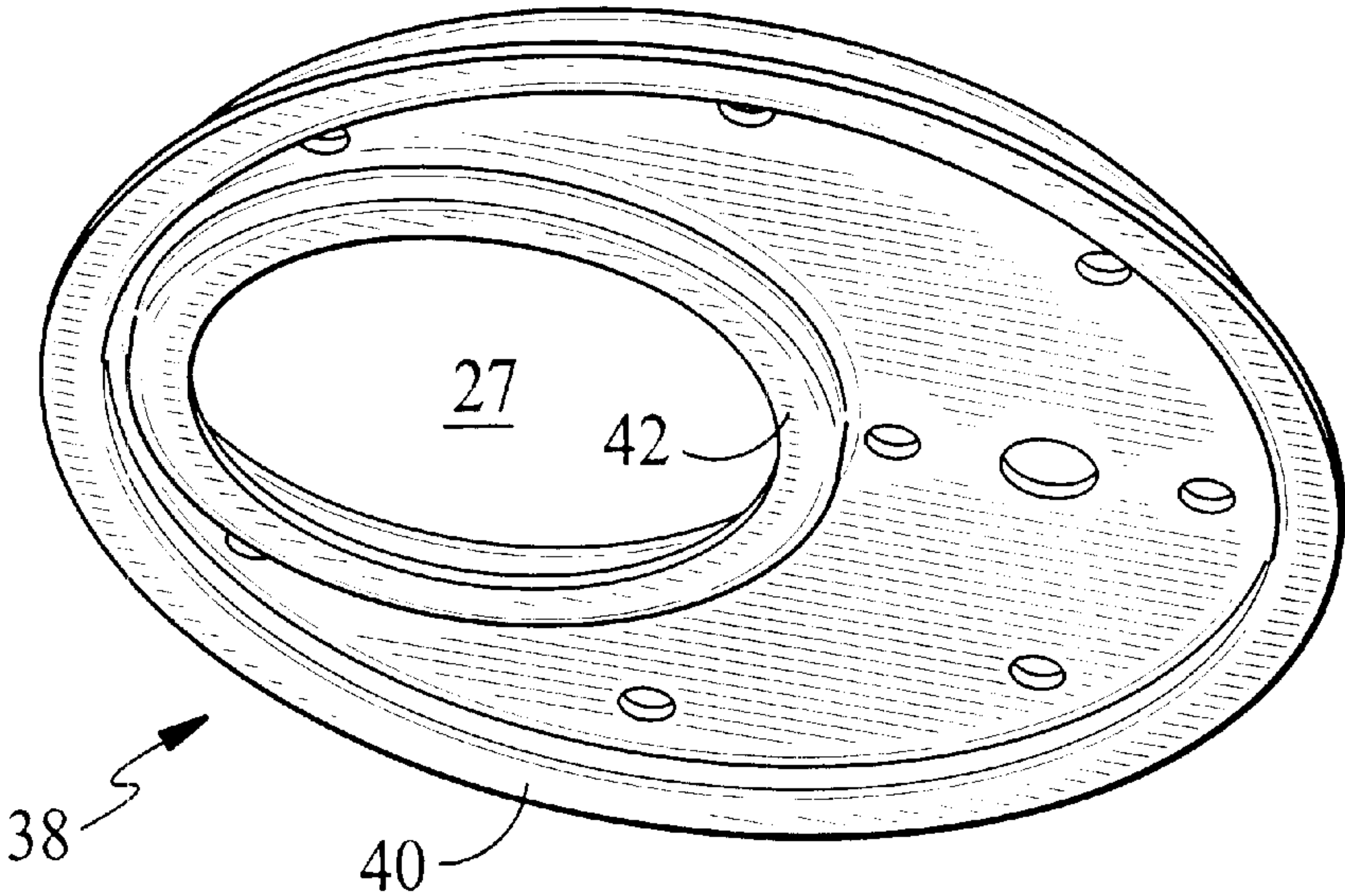
FIG. 15
