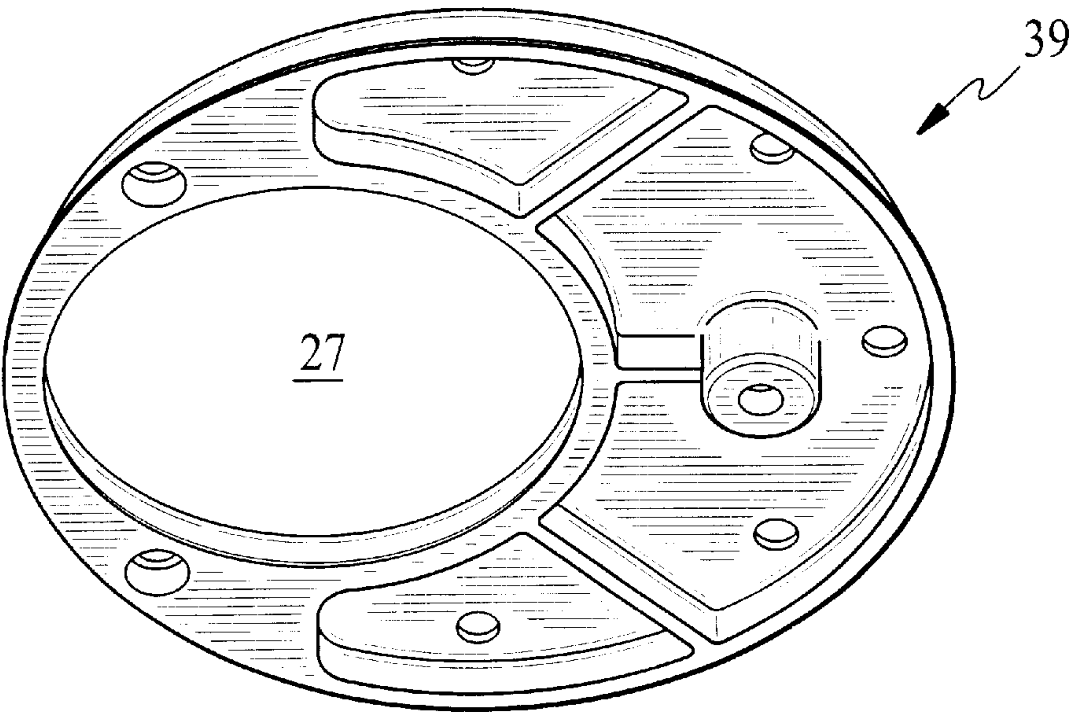
FIG. 20
