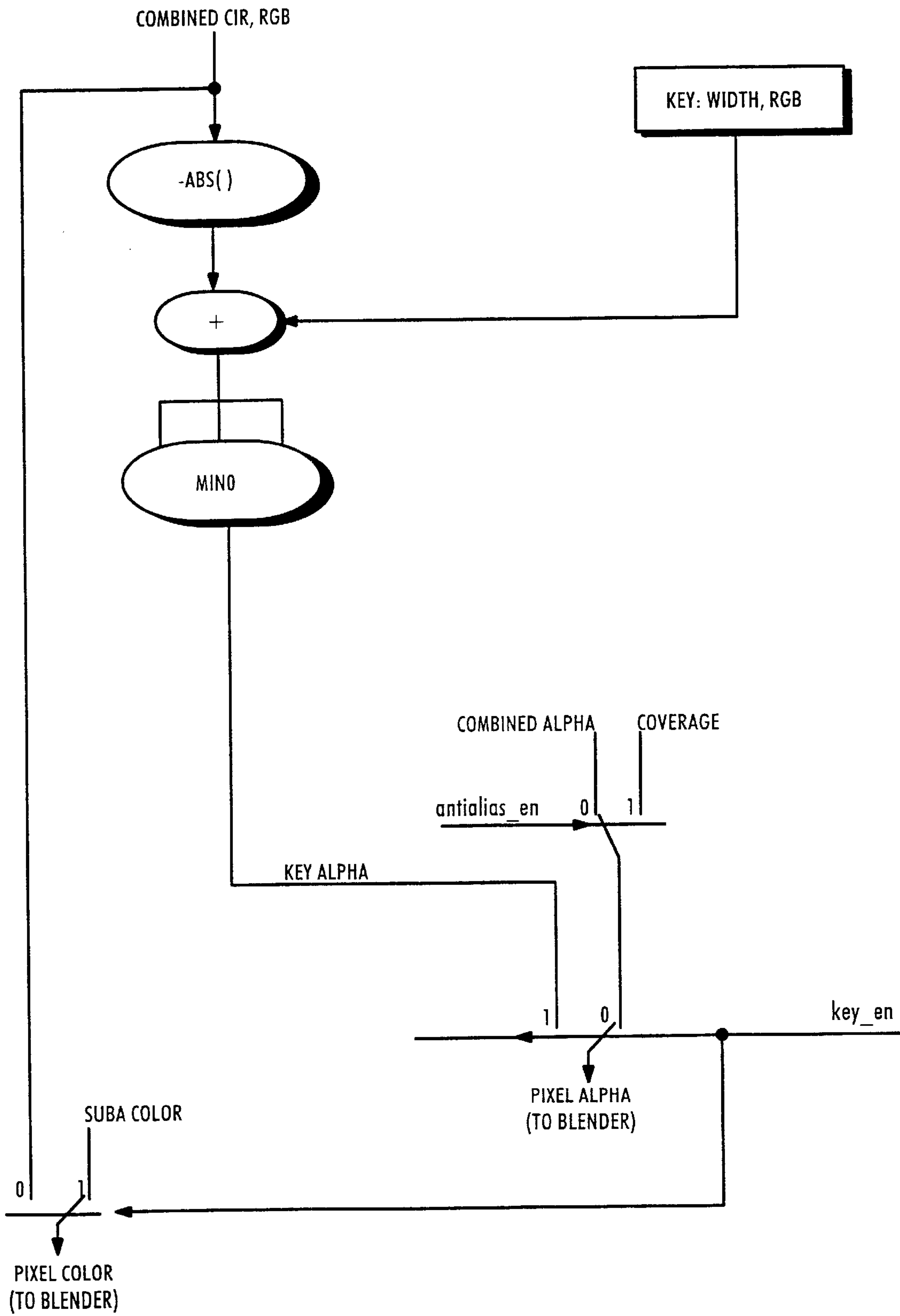
Fig. 29 ALPHA FIXUP
