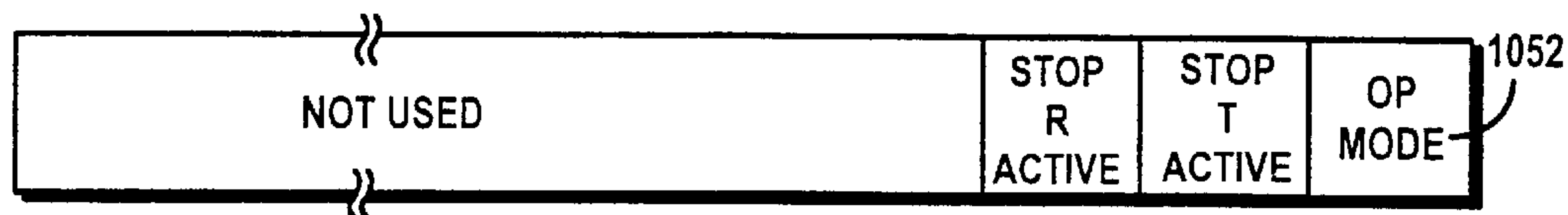
Fig. 37A MI MODE REGISTER(R/W)
