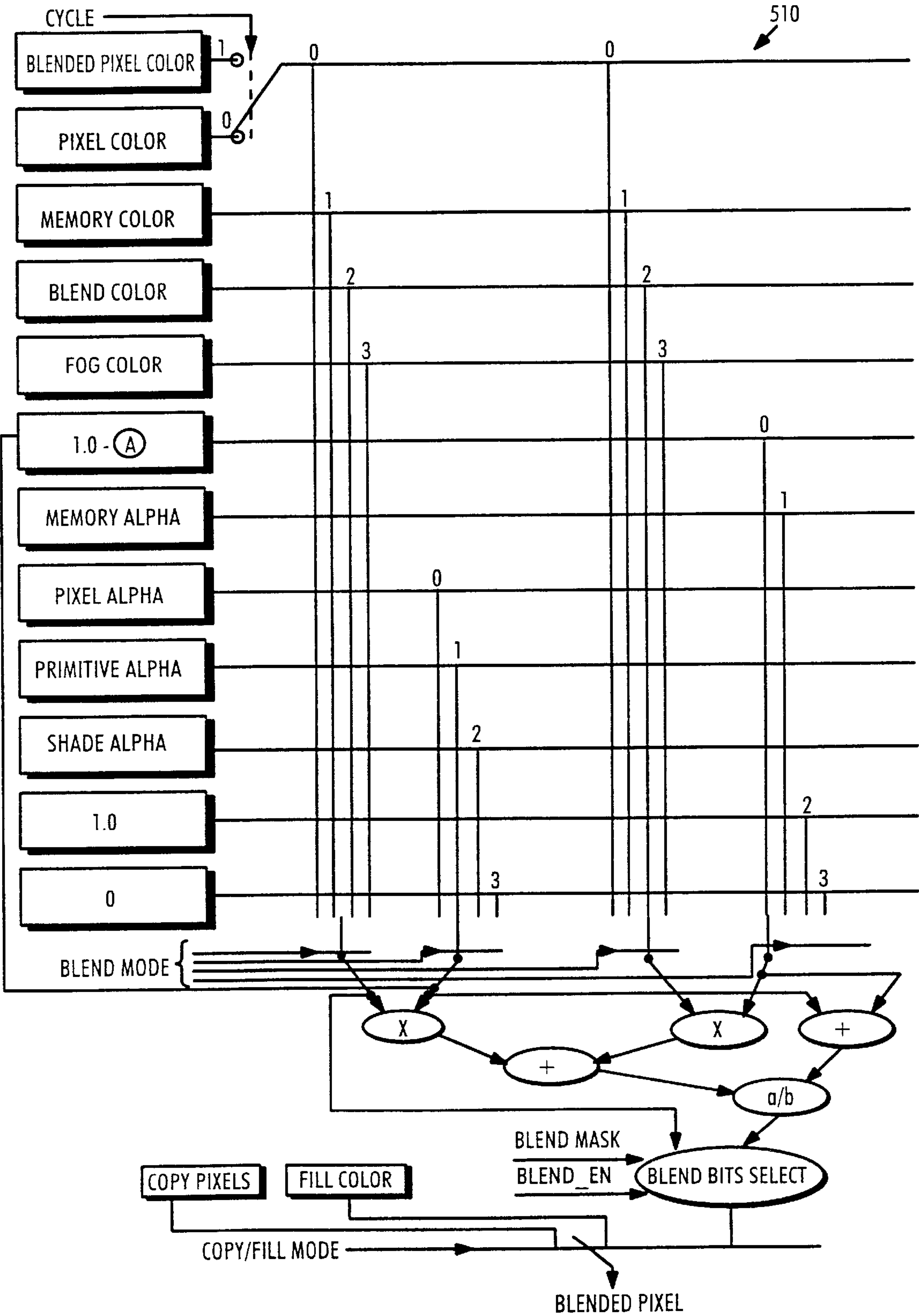
Fig. 31 BLENDER
