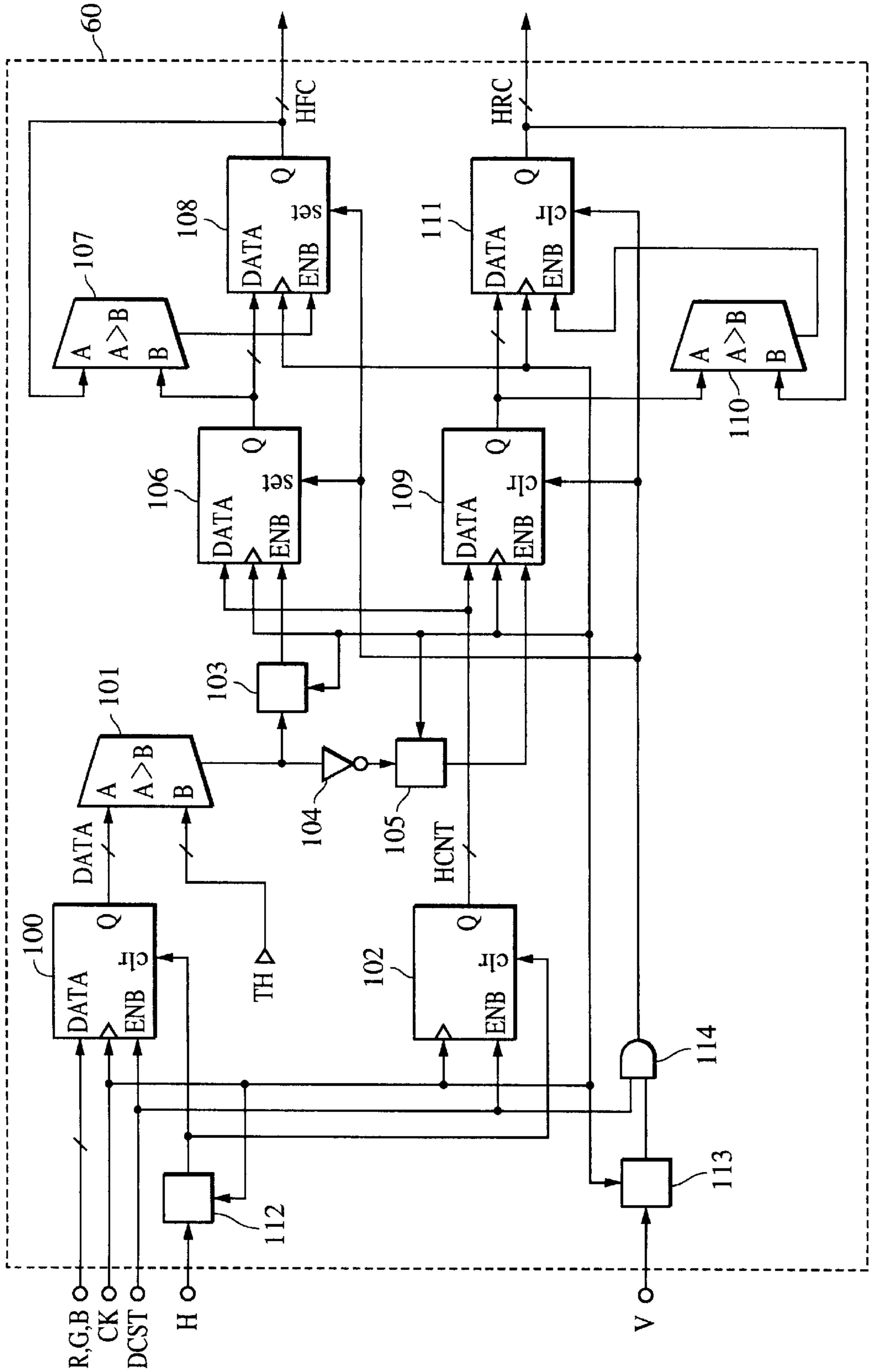
FIG. 4
