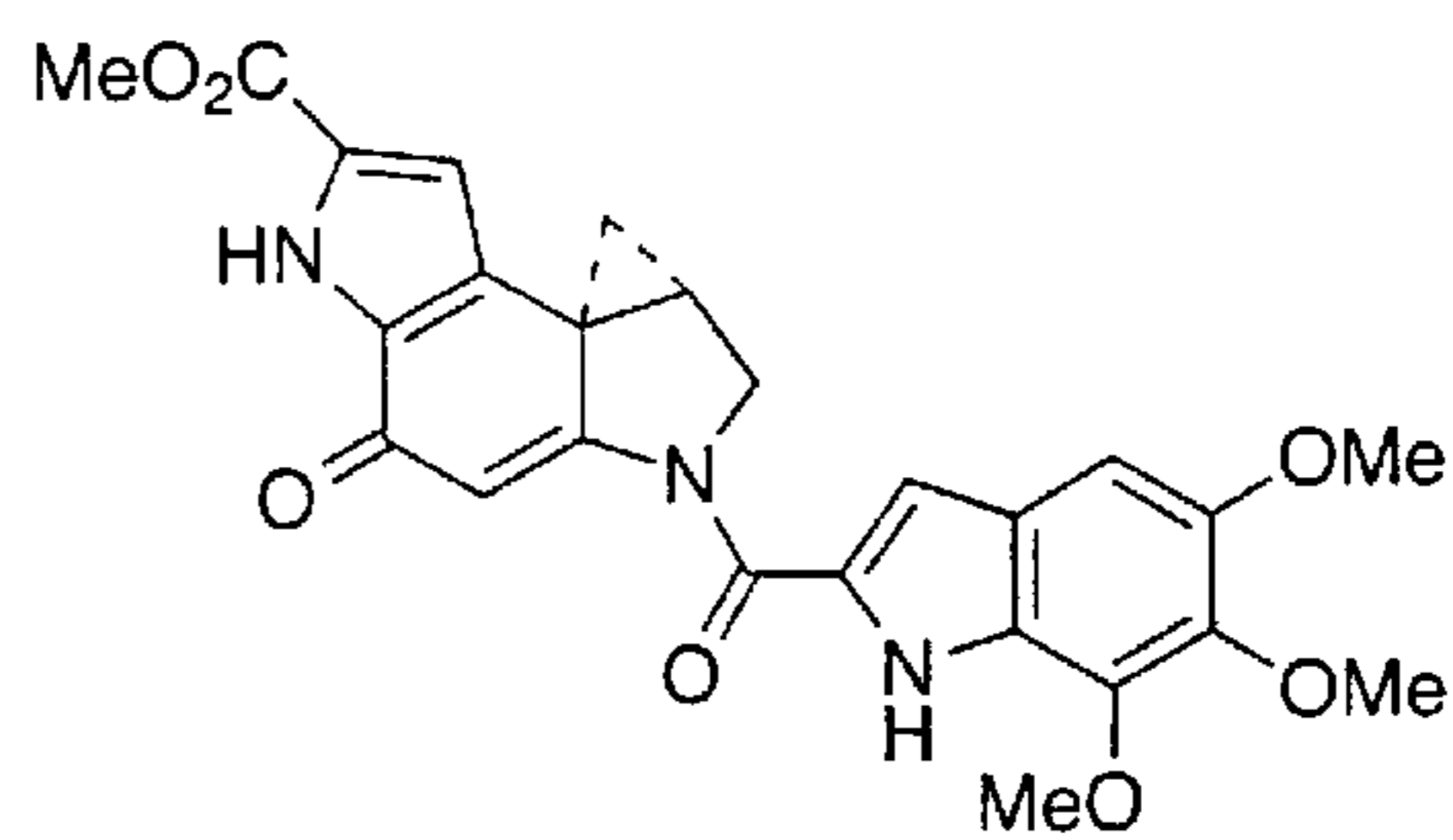
(+)- Duocarmycin SA
