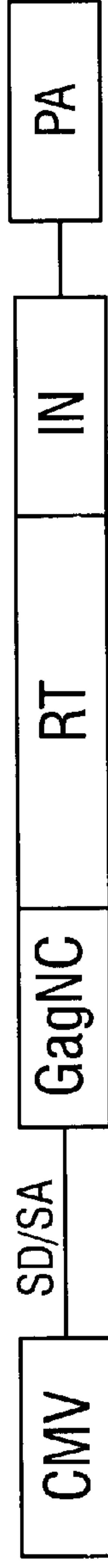
FIG. 21B pCMV, GagNC-RT-IN
