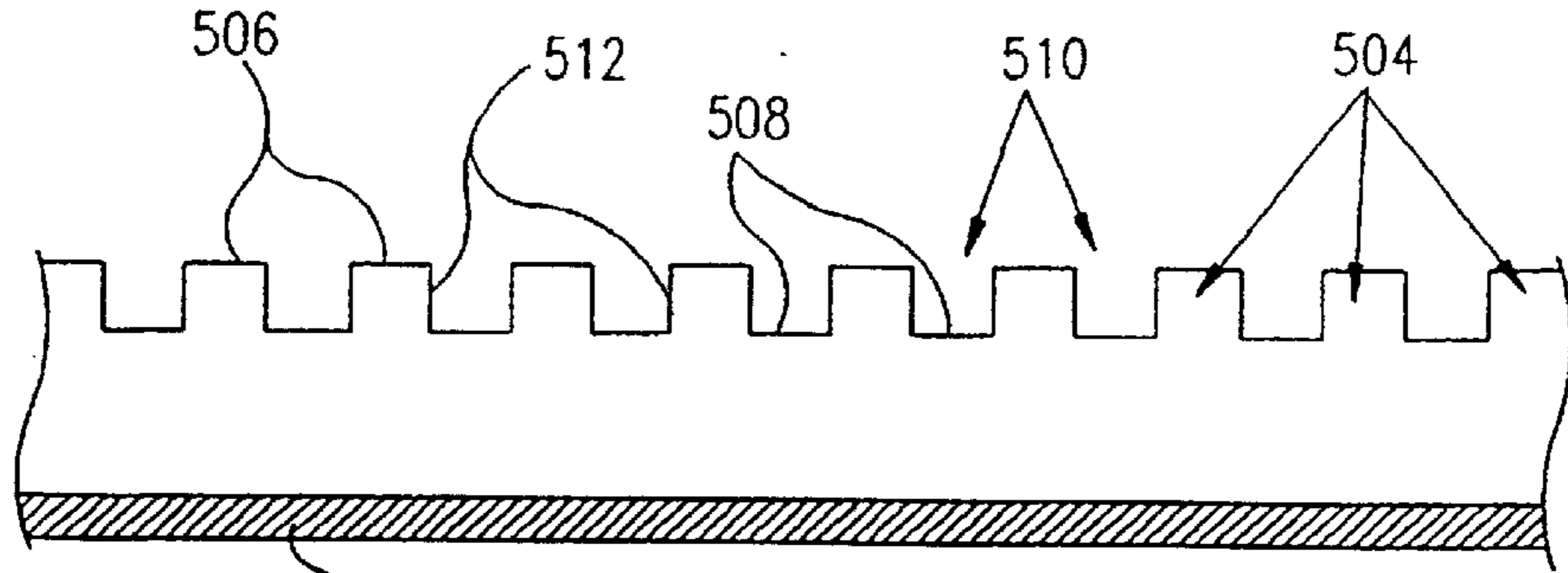
FIG. 14B
