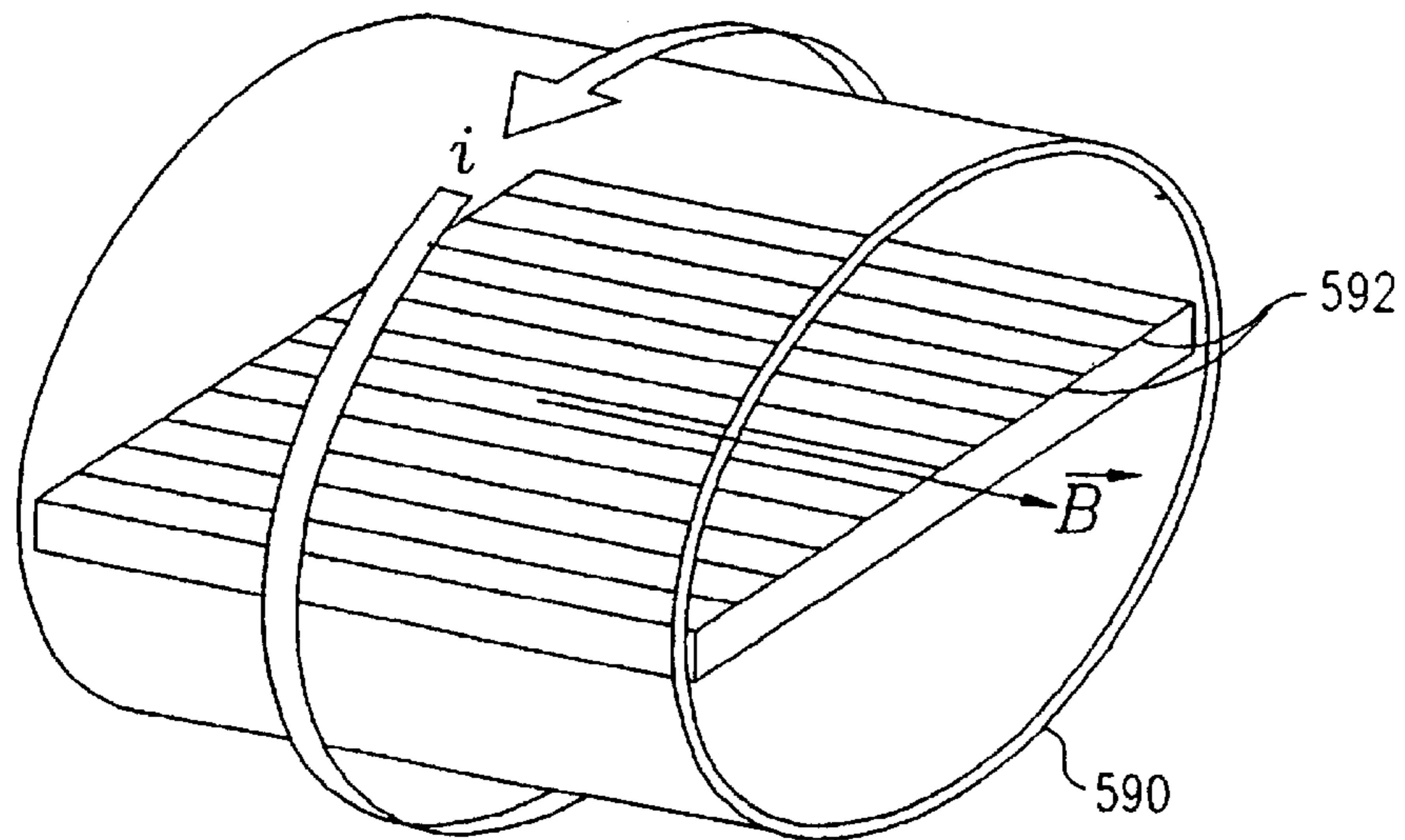
FIG. 19
