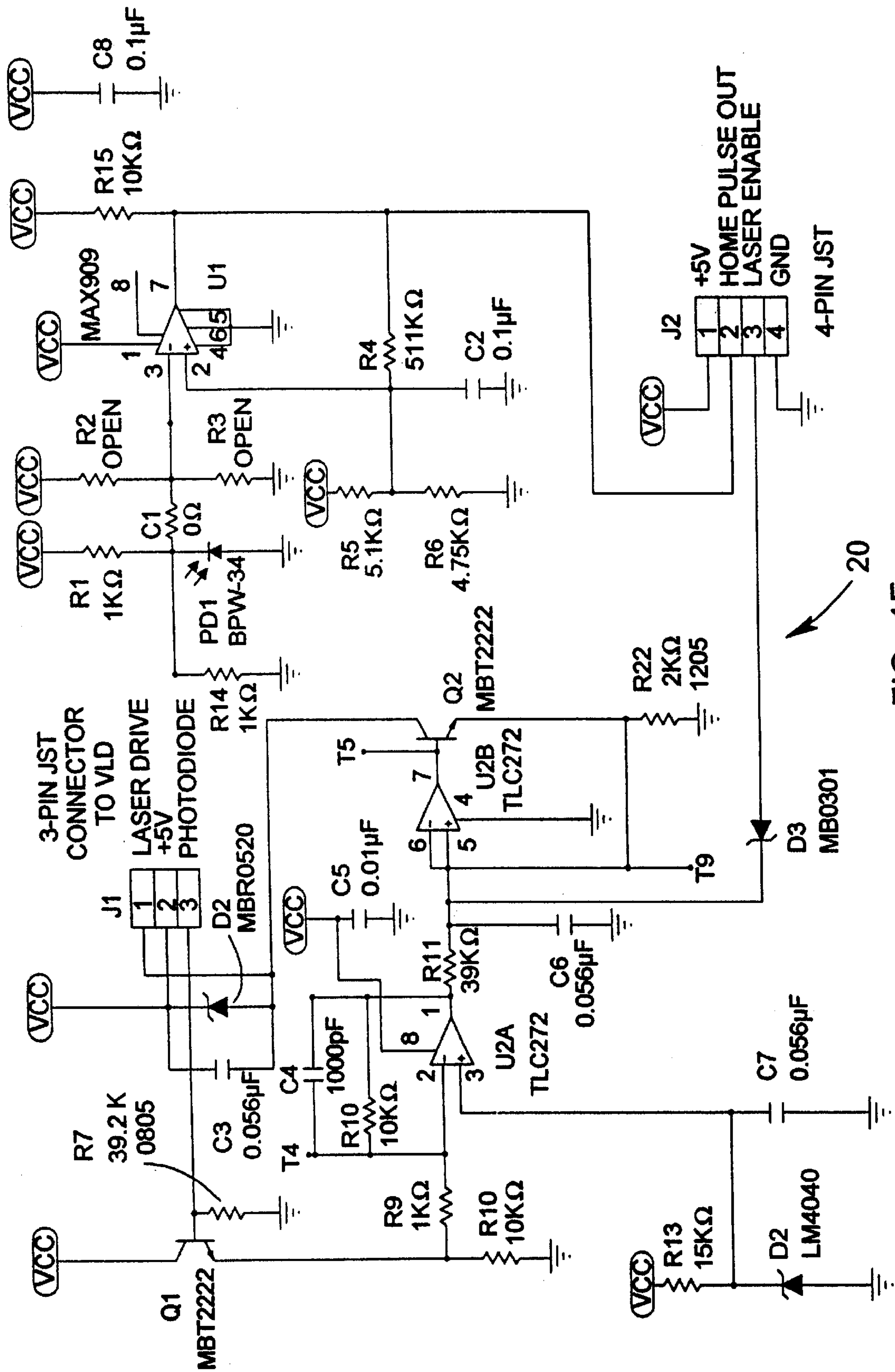
FIG. 1F
