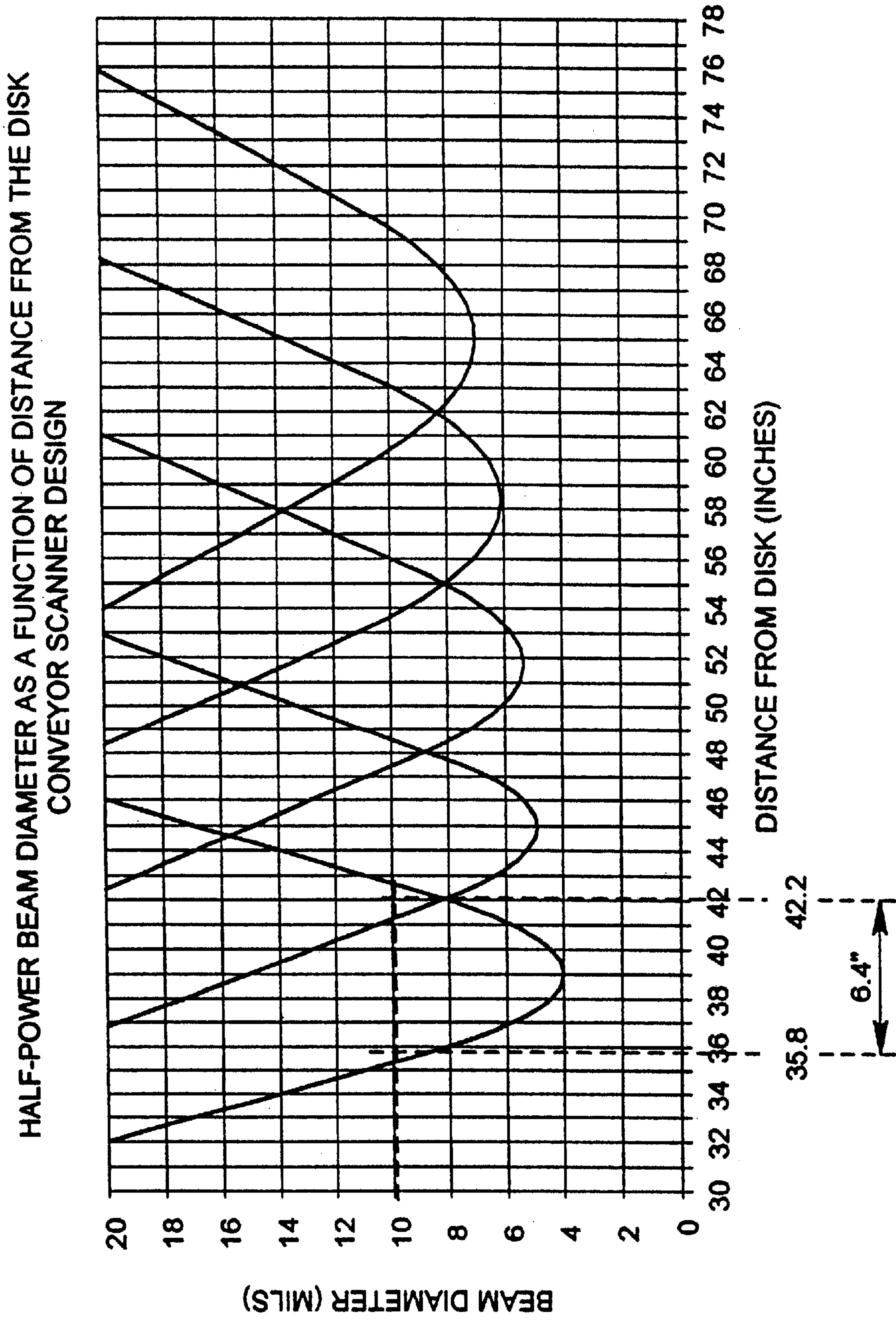
FIG. 5A
