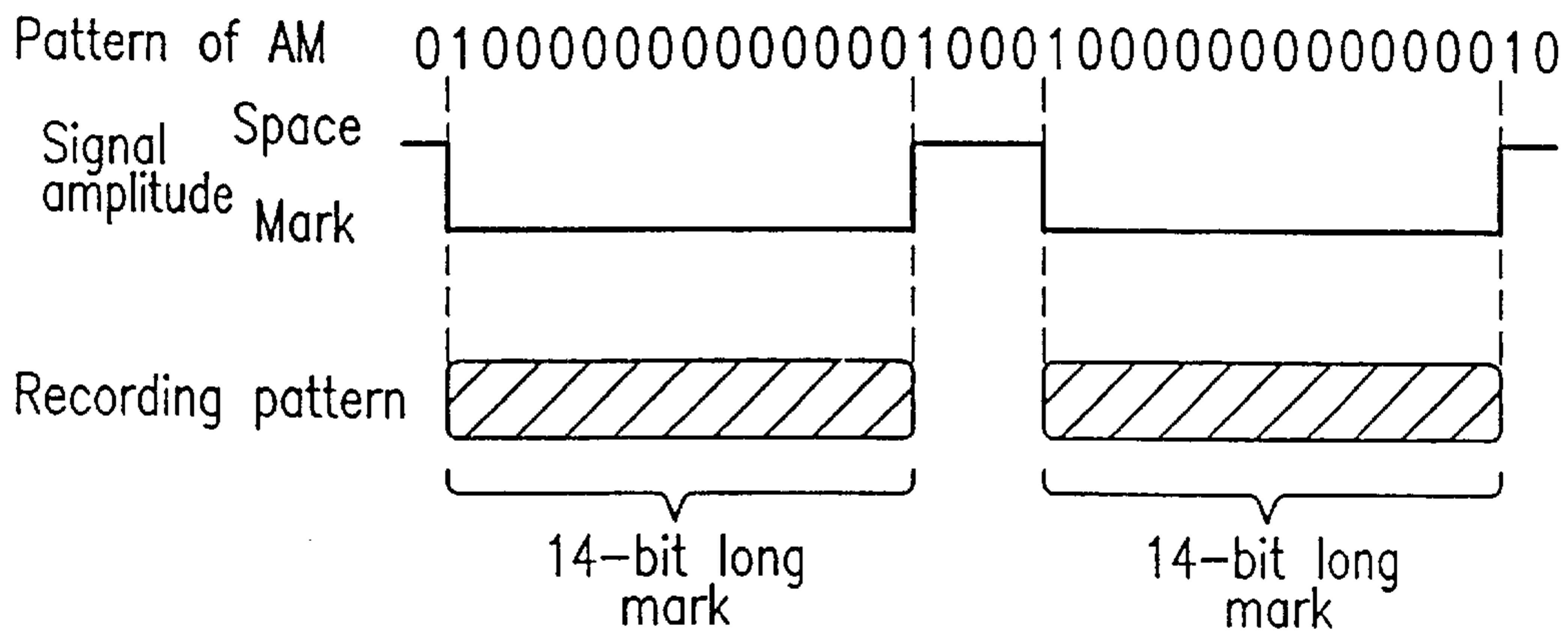
FIG. 7B
