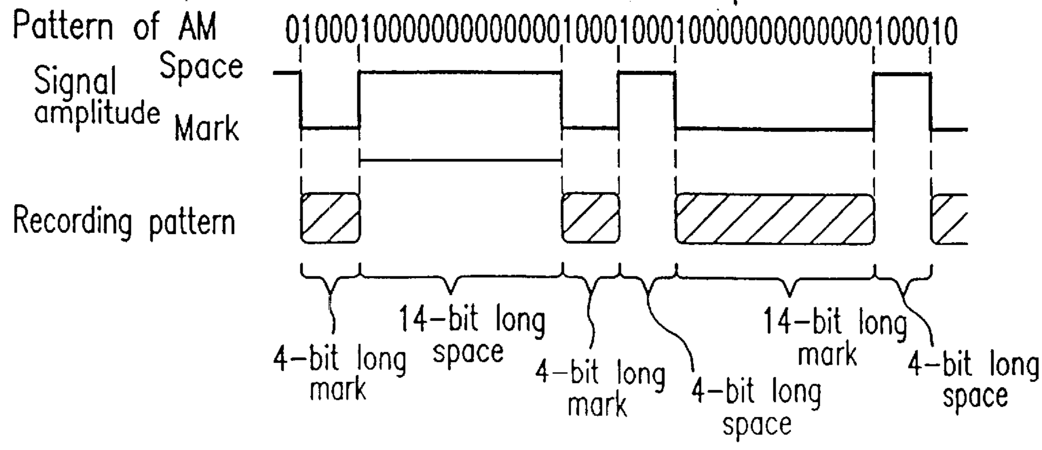
FIG. 8D
