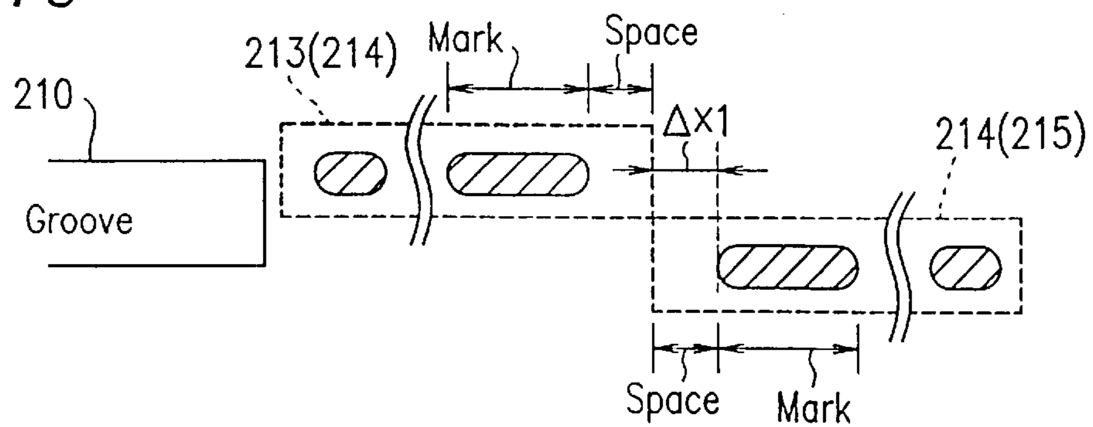
FIG. 21C
