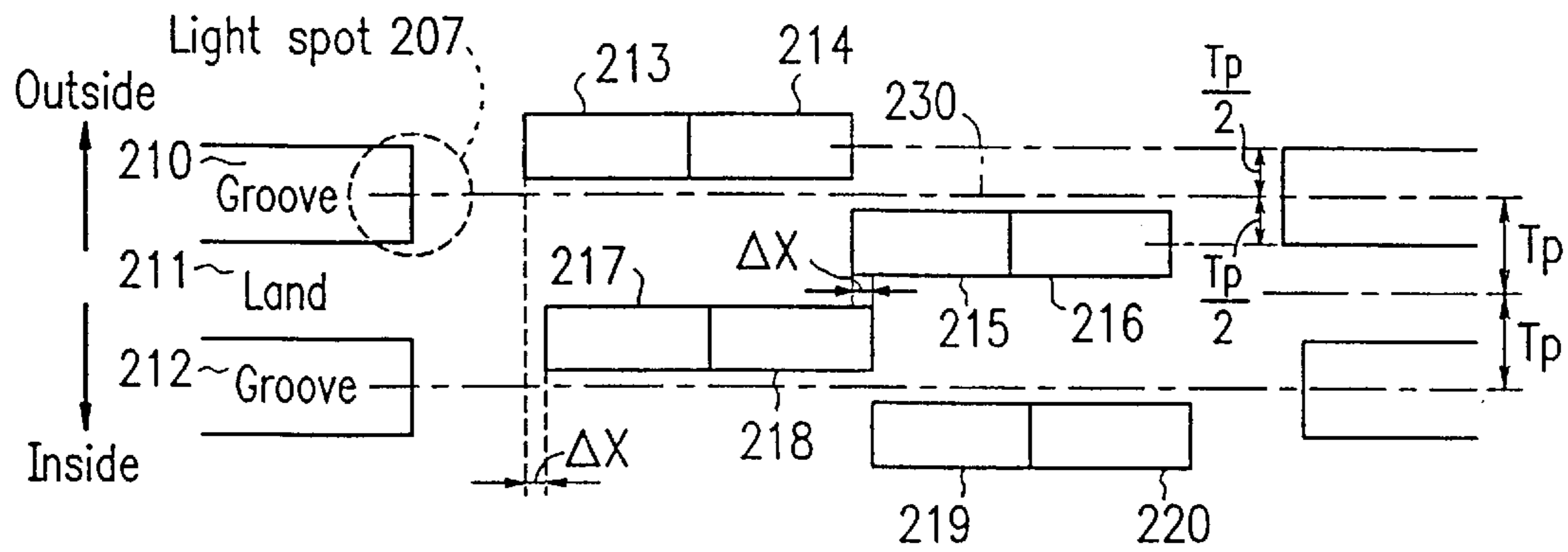
FIG. 21B
