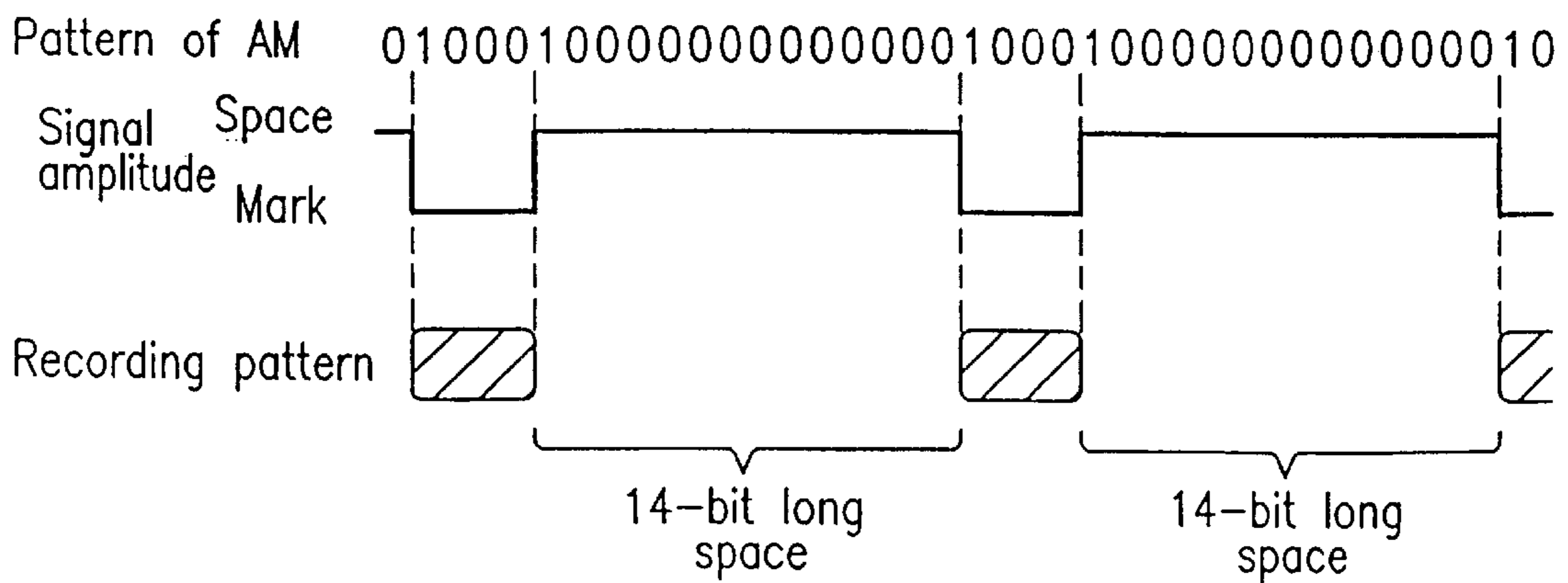
FIG. 7C
