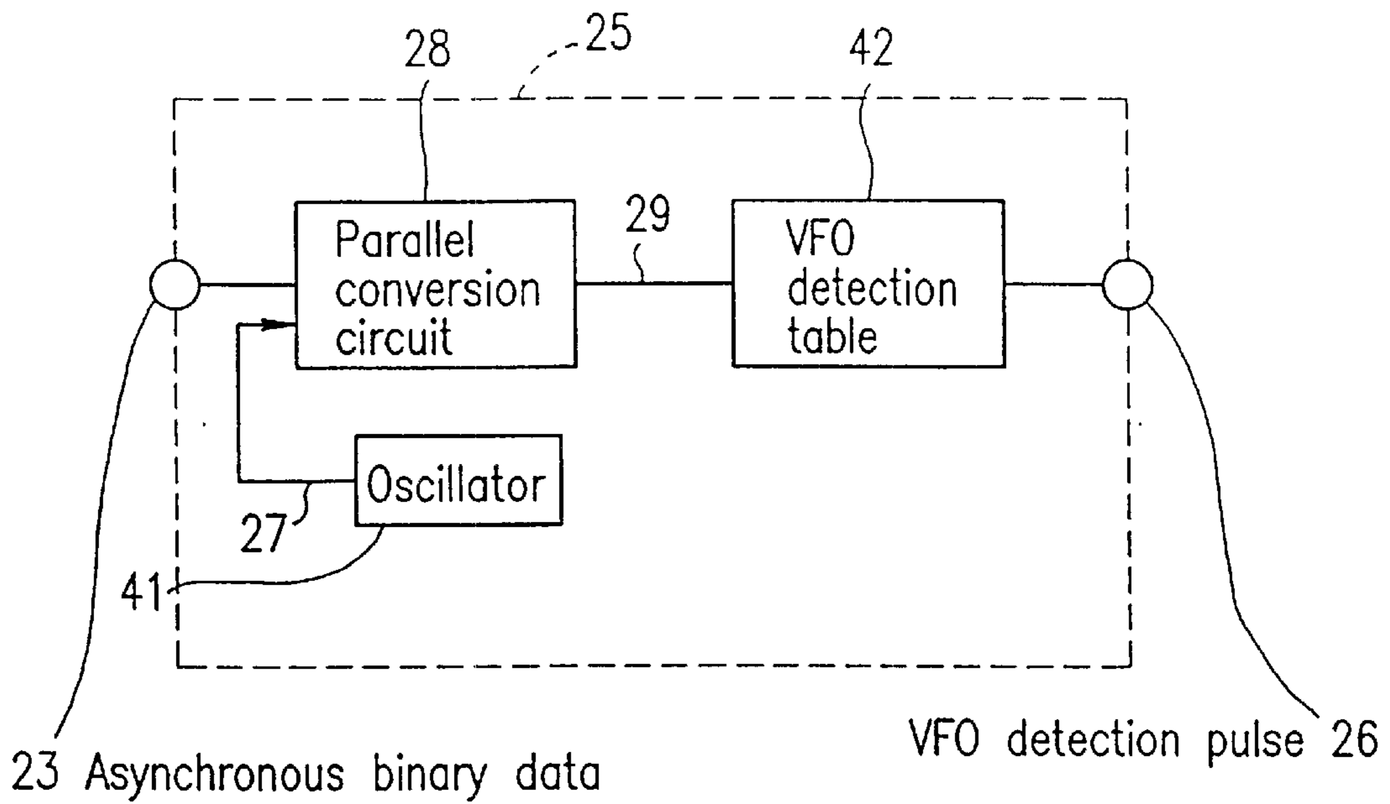
FIG. 12A
