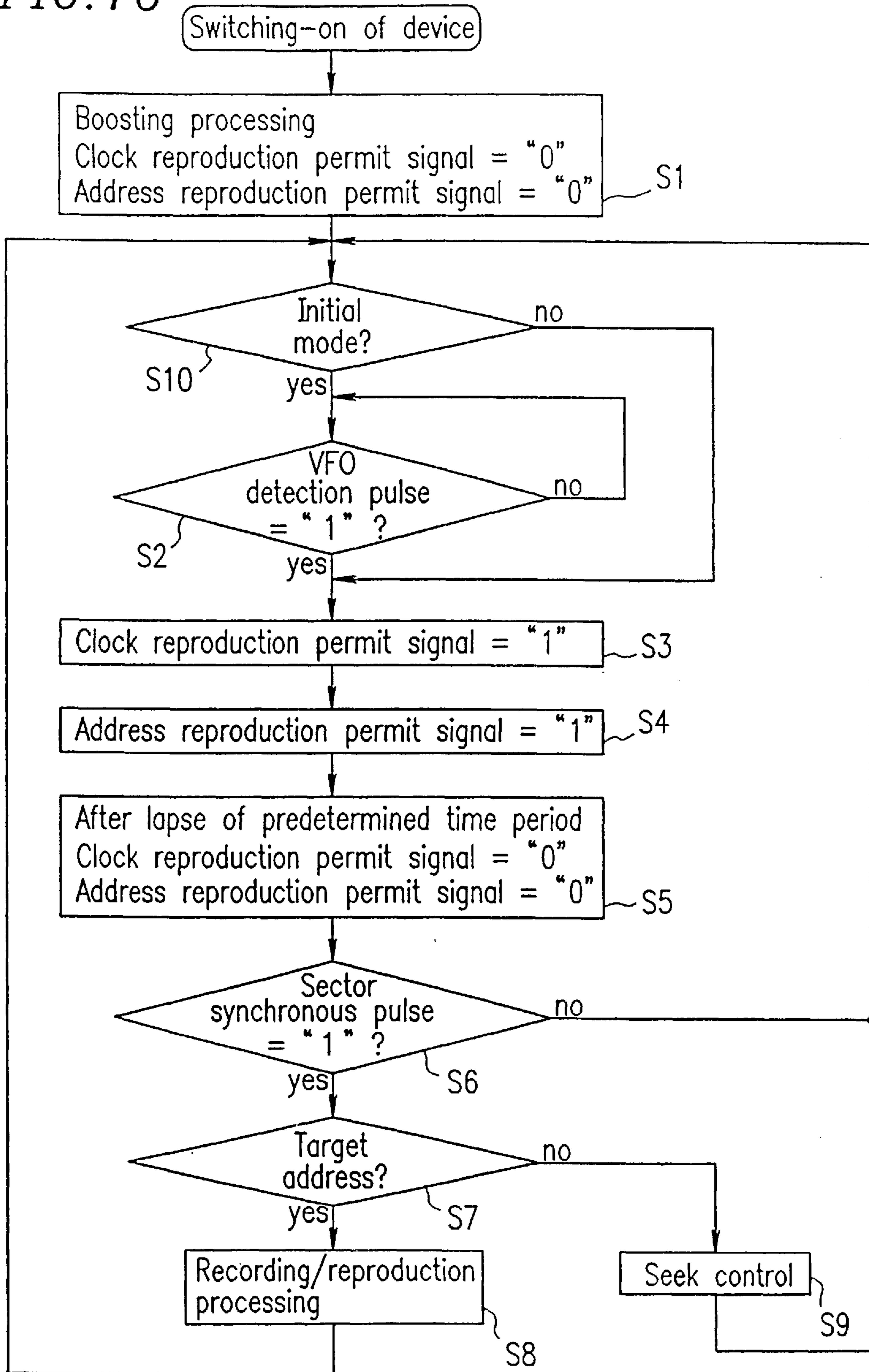
FIG. 16
