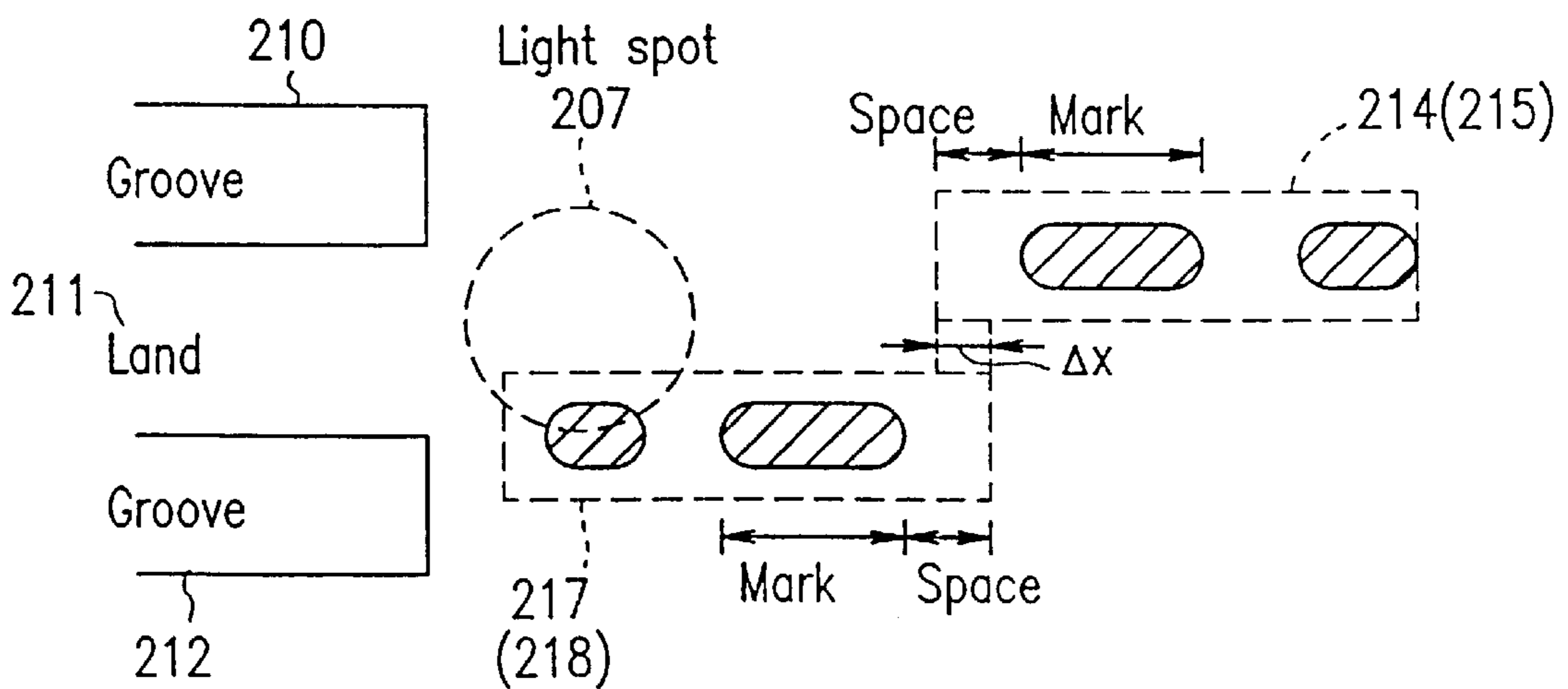
FIG. 23B
