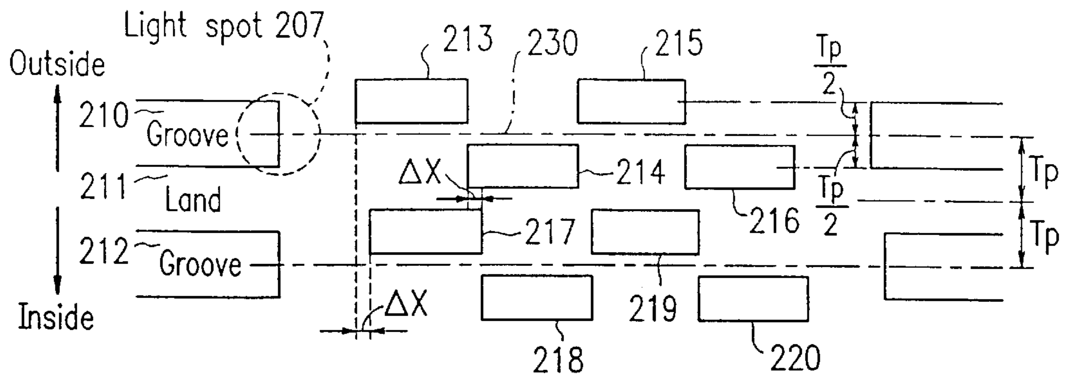
FIG. 21A
