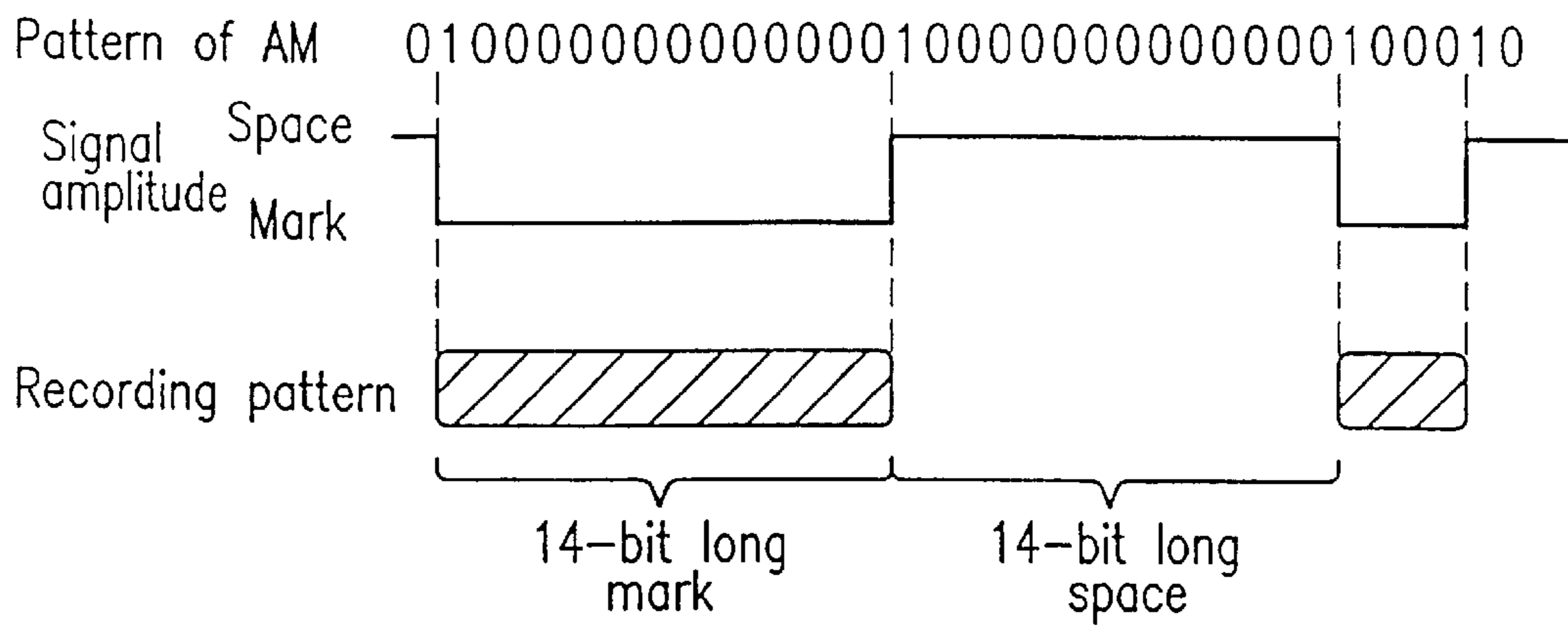
FIG. 7A
