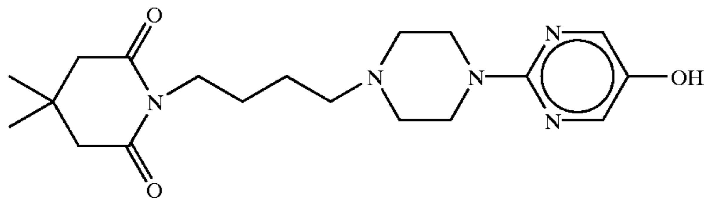
5-OH gepirone
