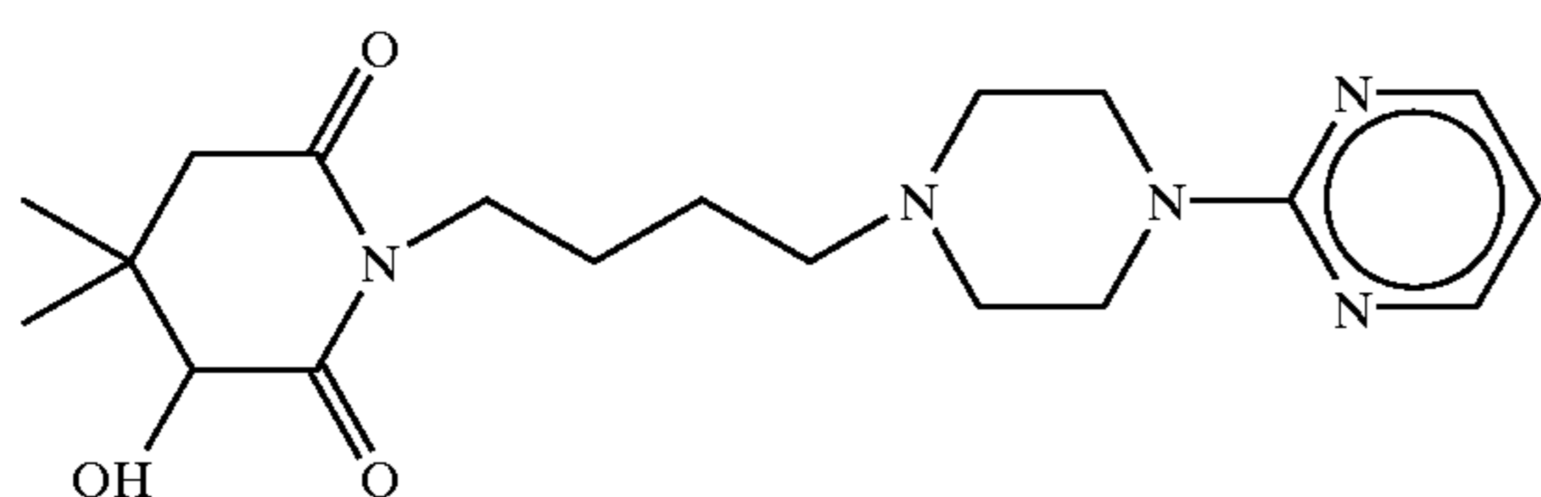
3-OH gepirone
