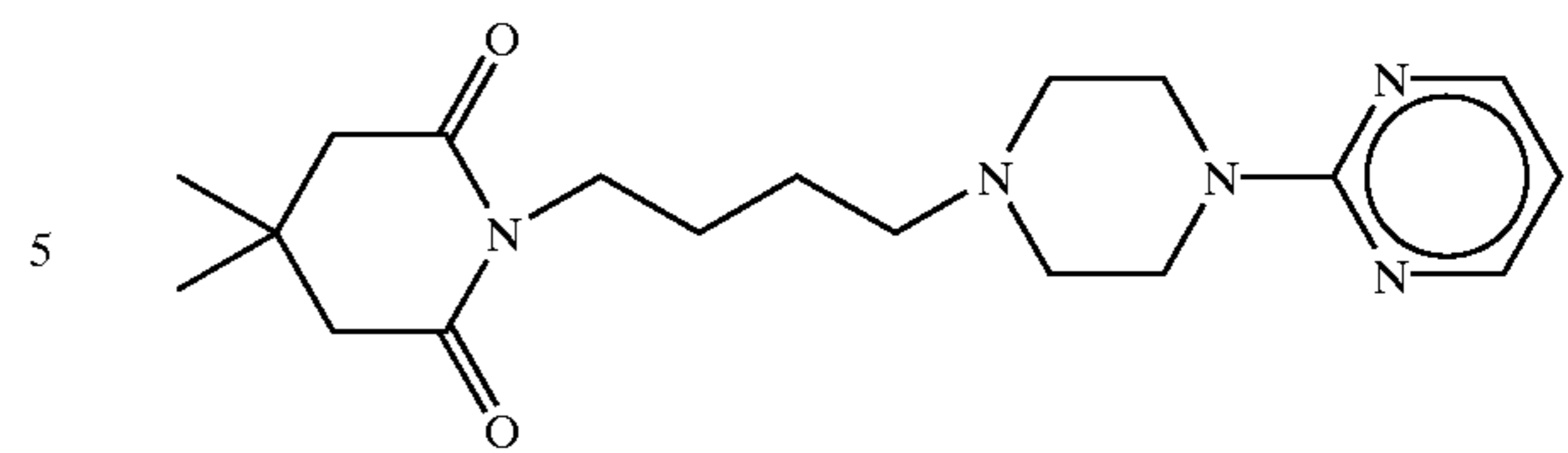
gepirone
