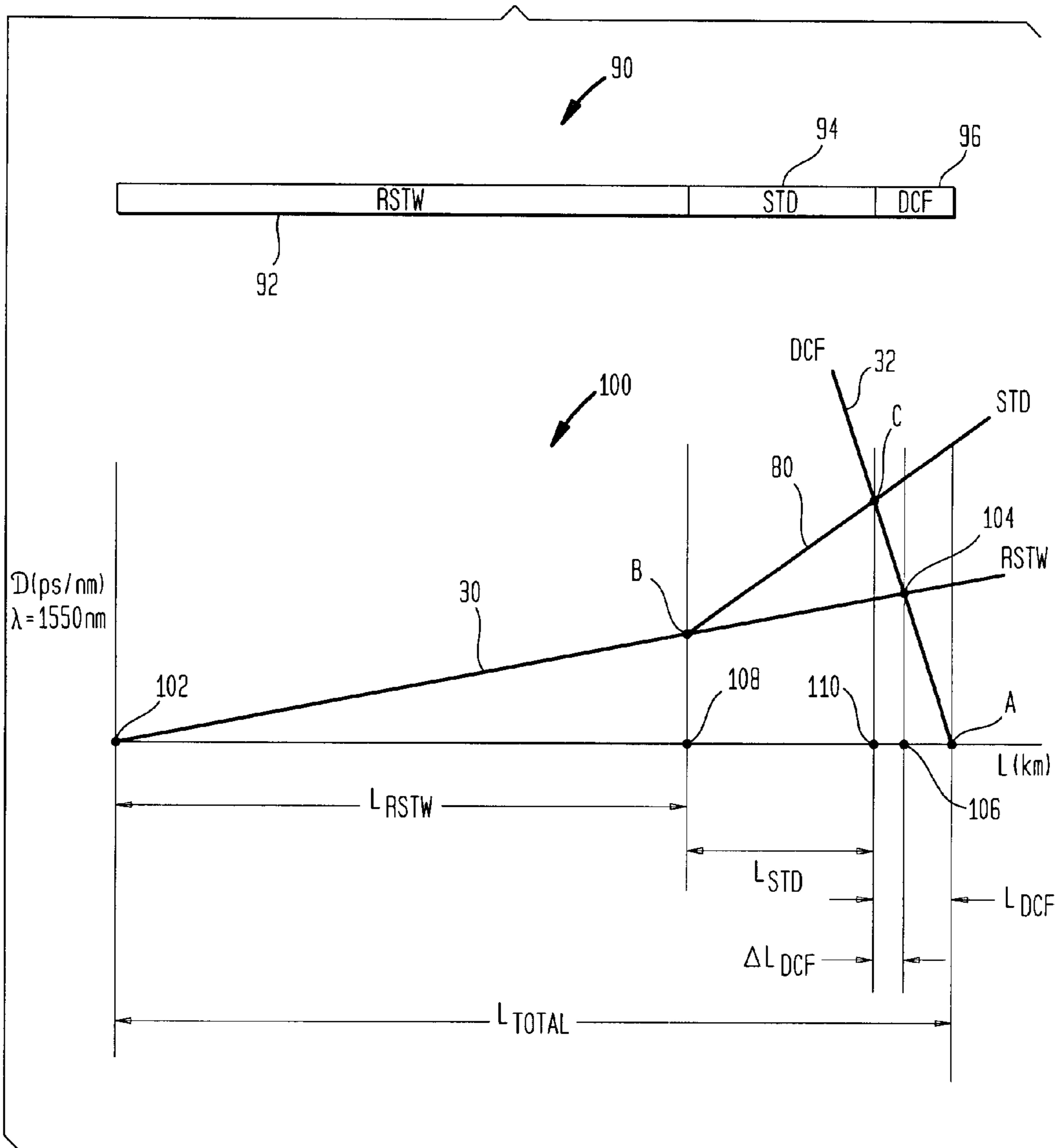
FIG. 15
