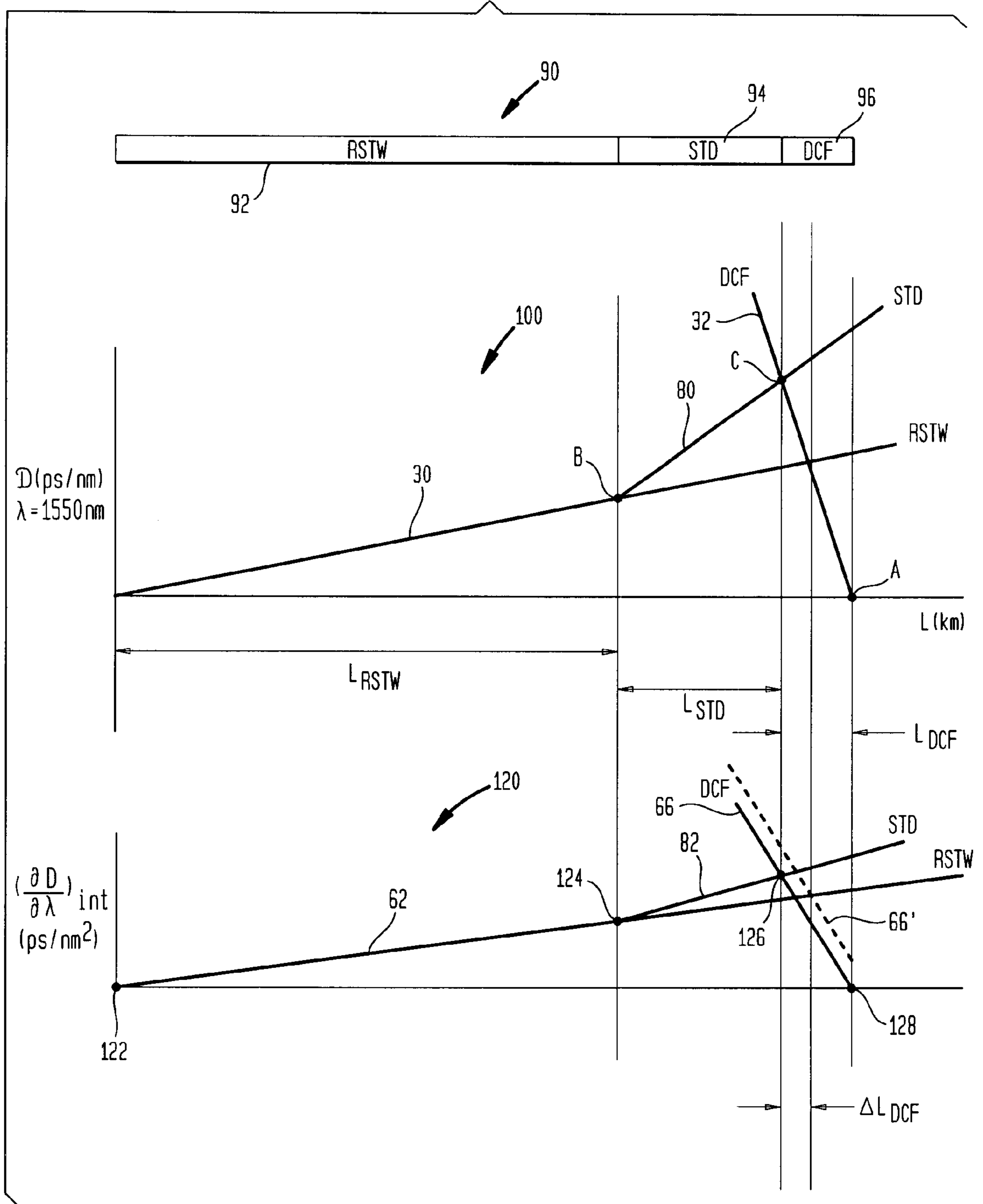
FIG. 16
