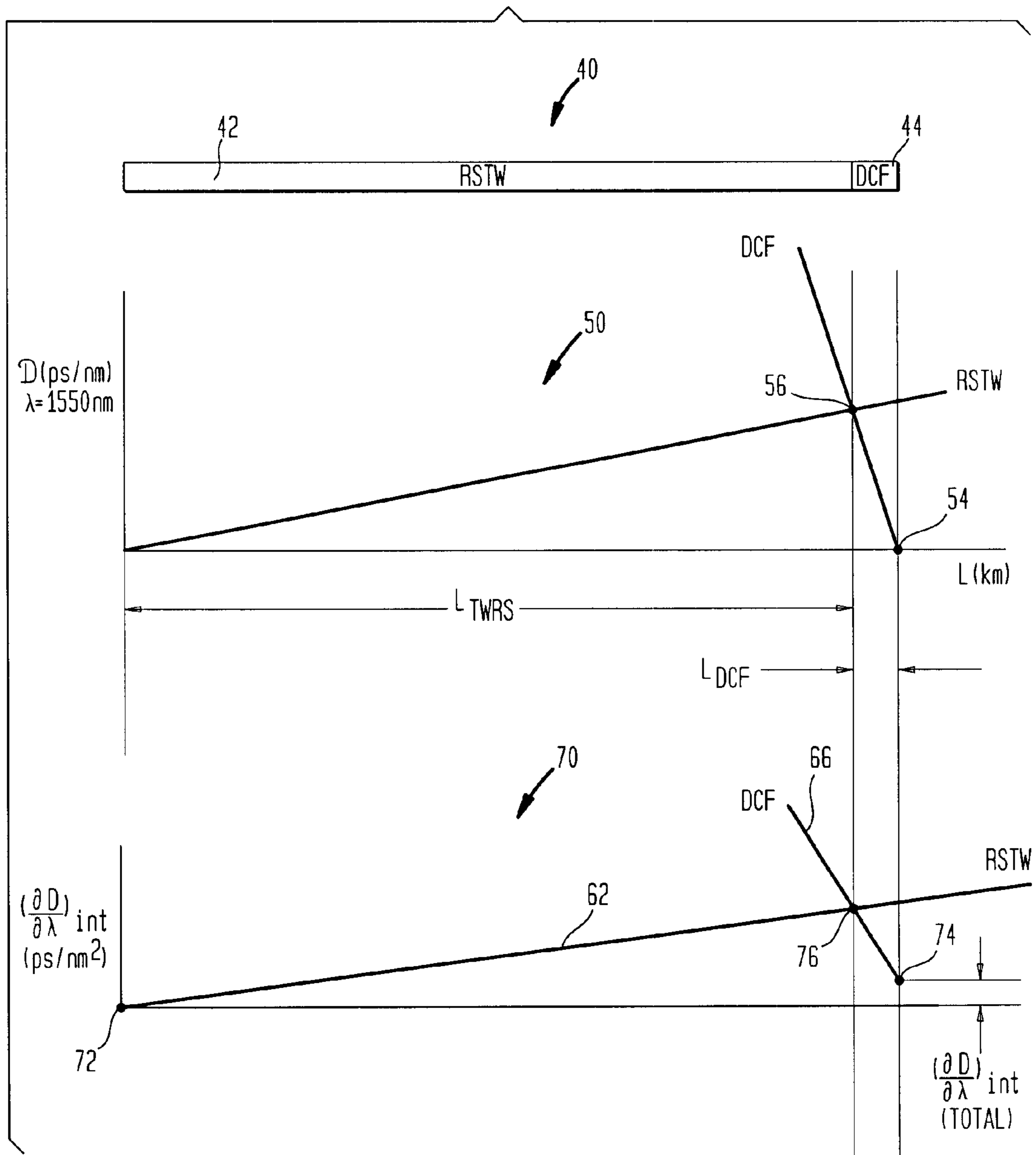
FIG. 12
