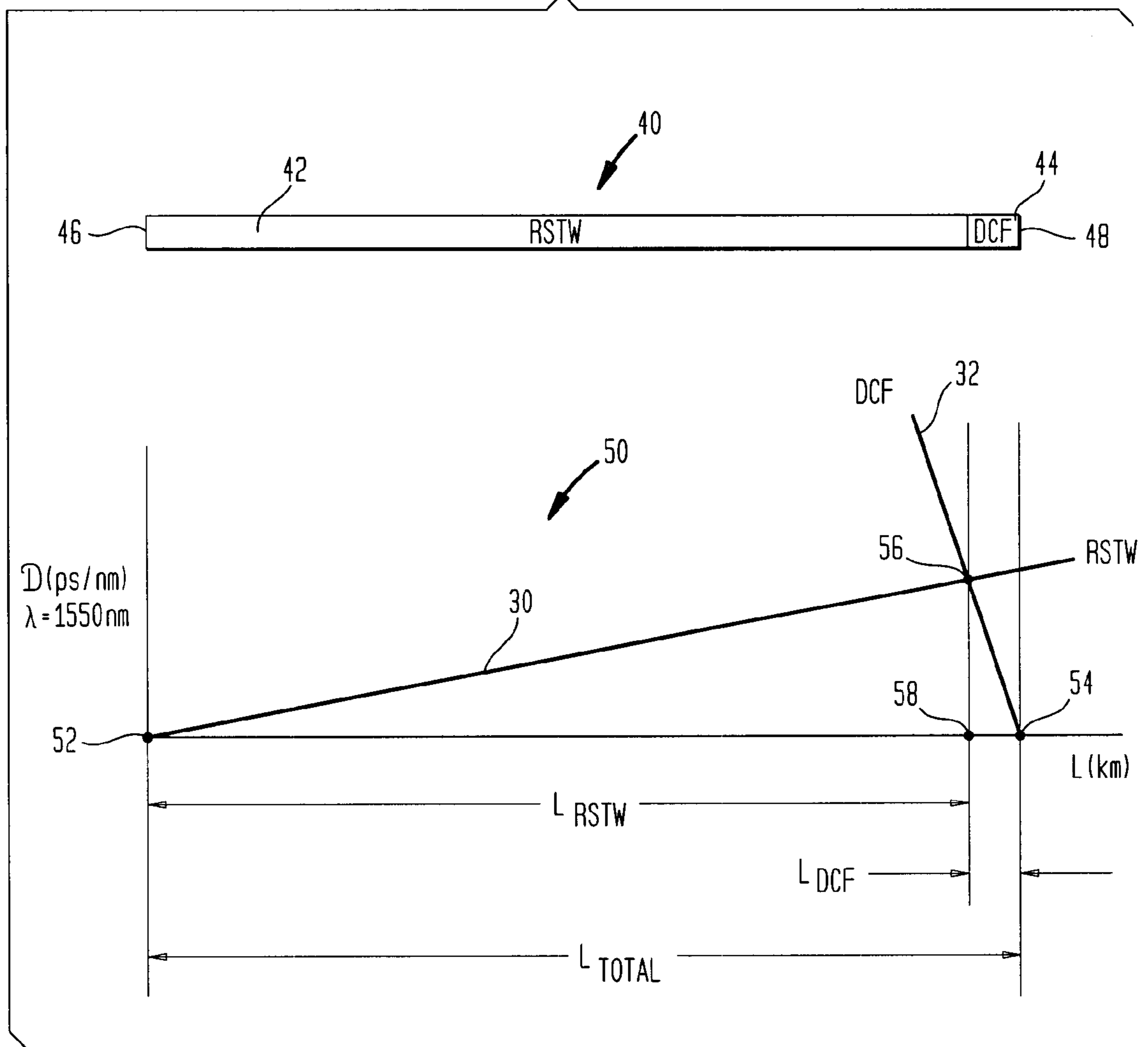
FIG. 7
