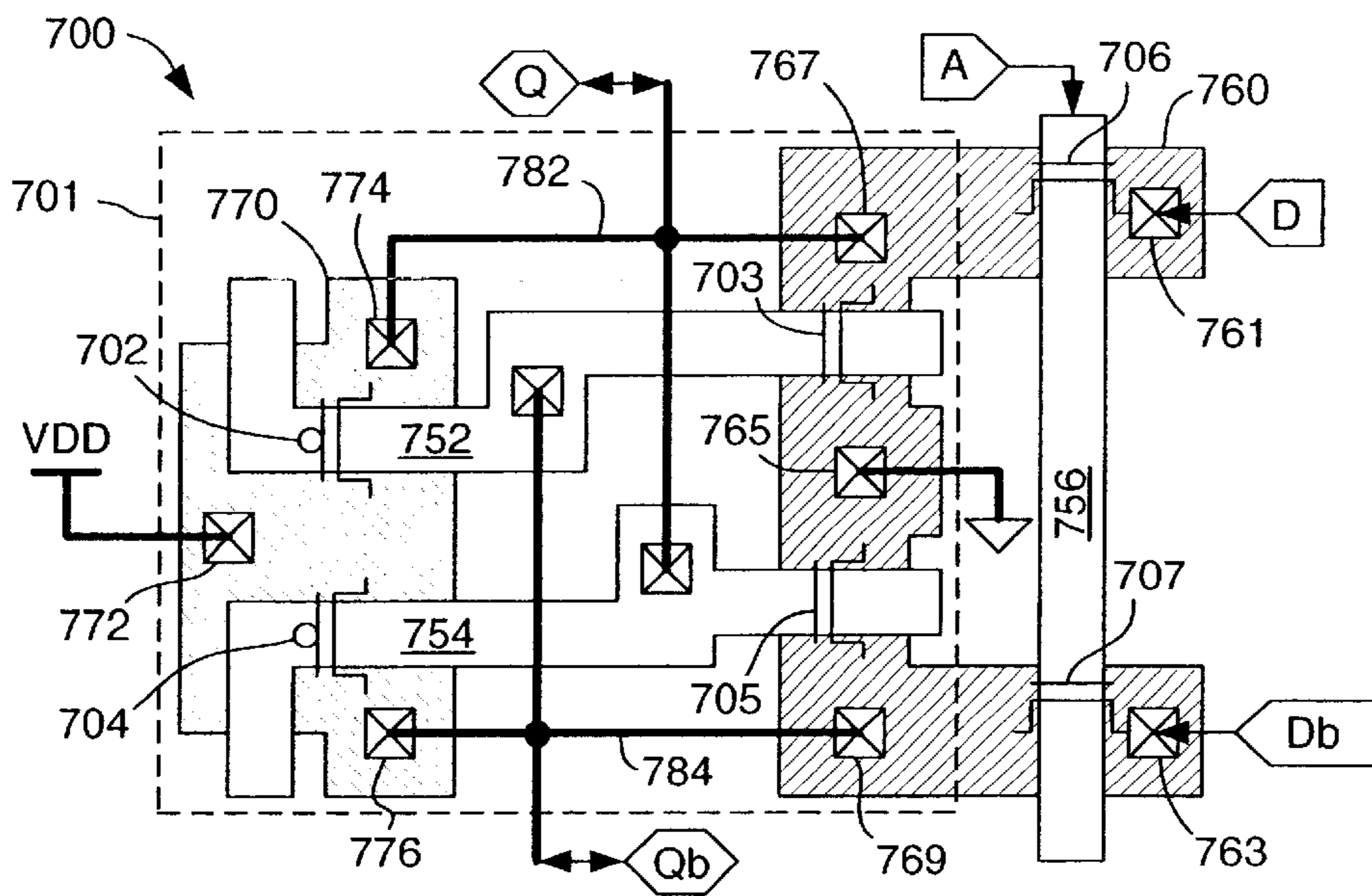
FIG. 7D
