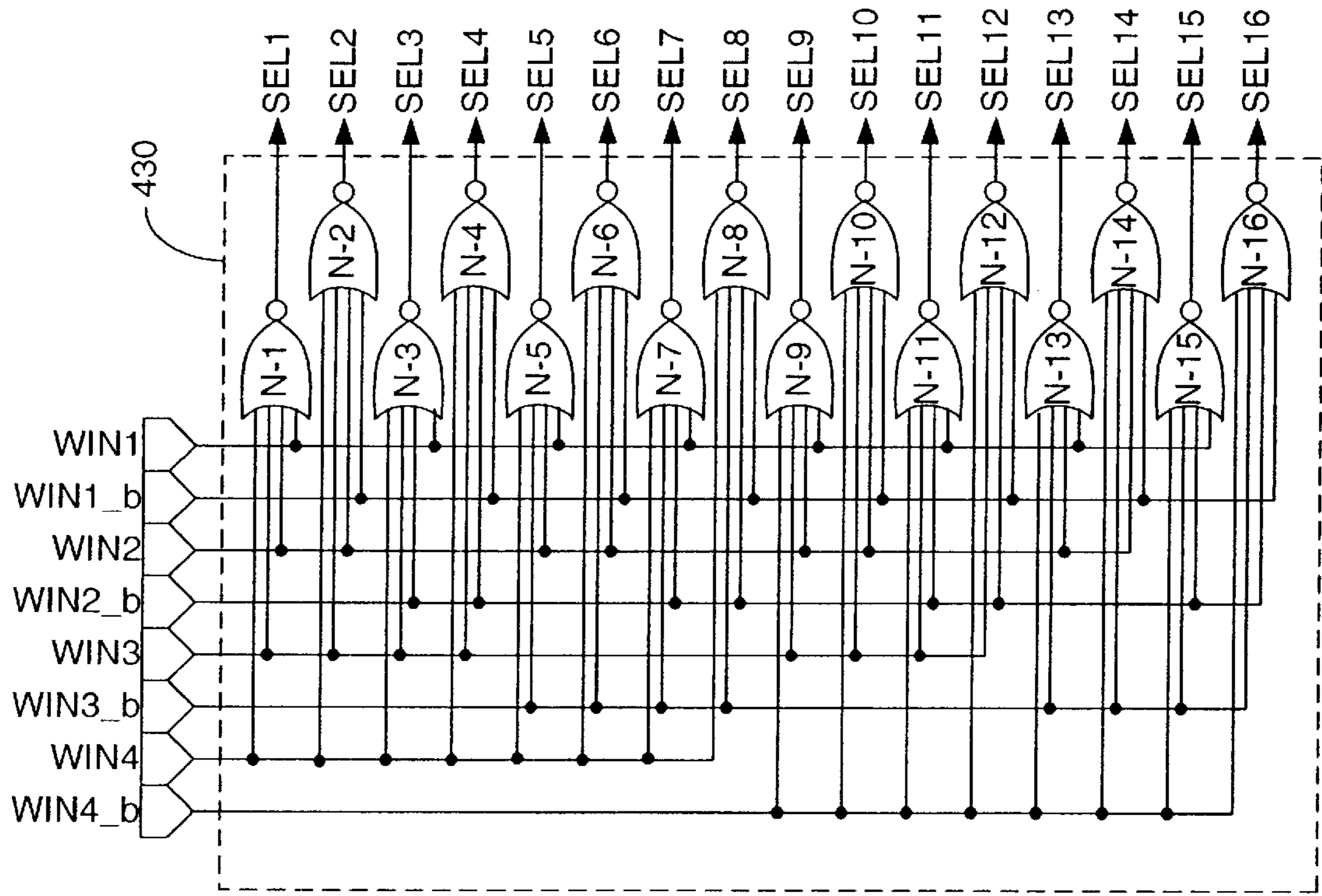
FIG. 6A
