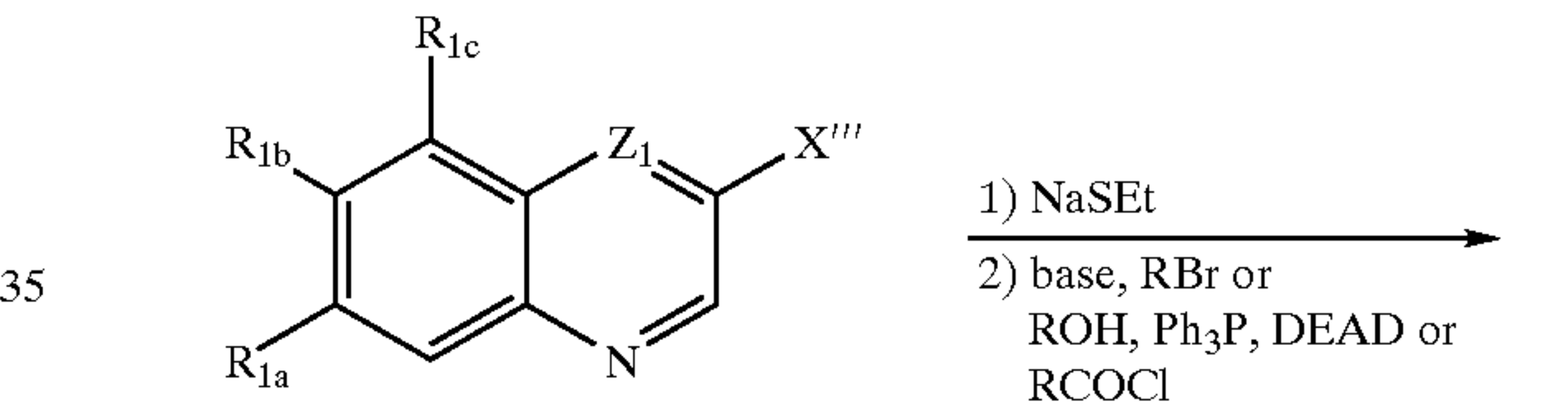
Scheme VI
