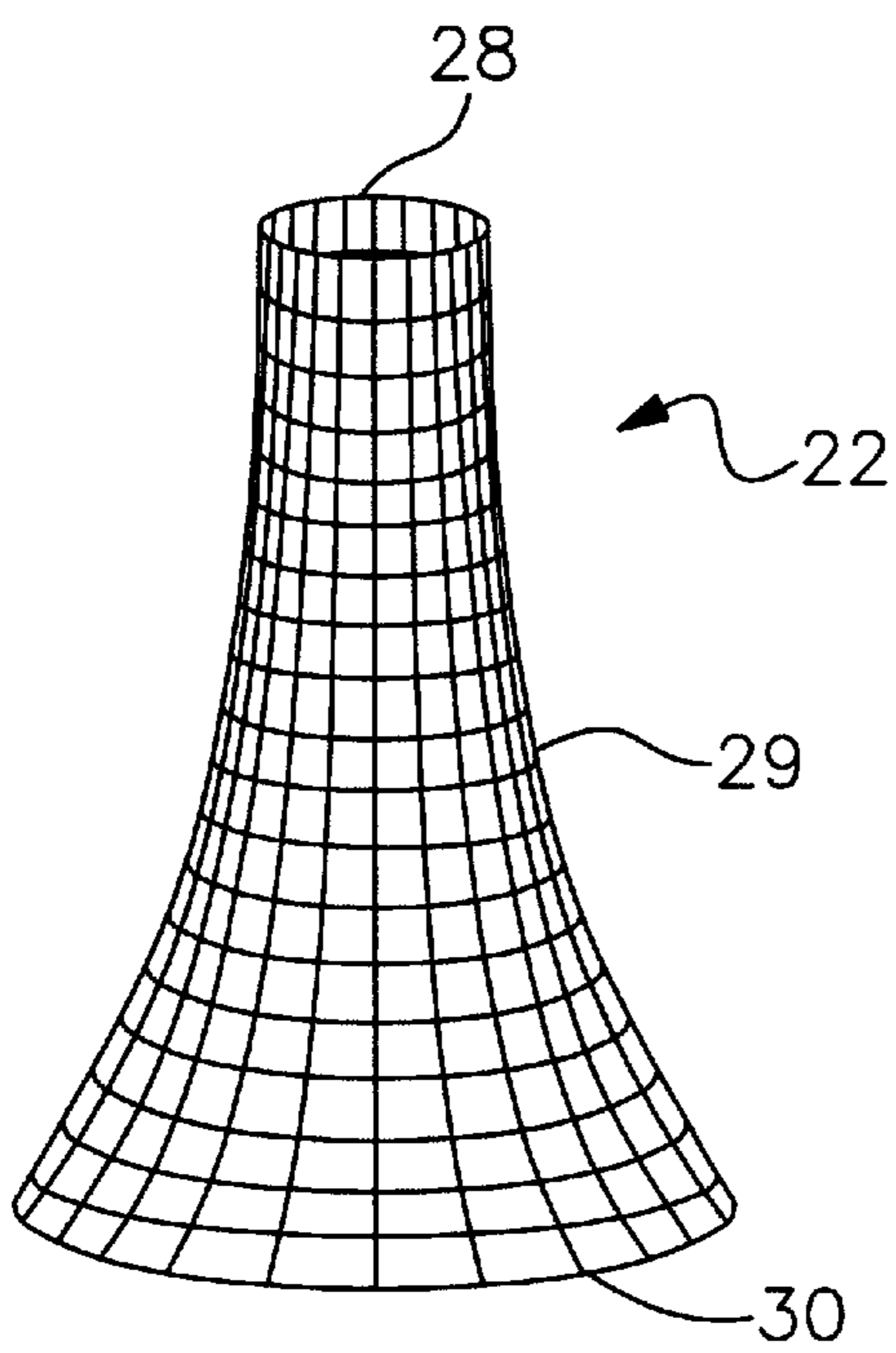
Fig. 6C
