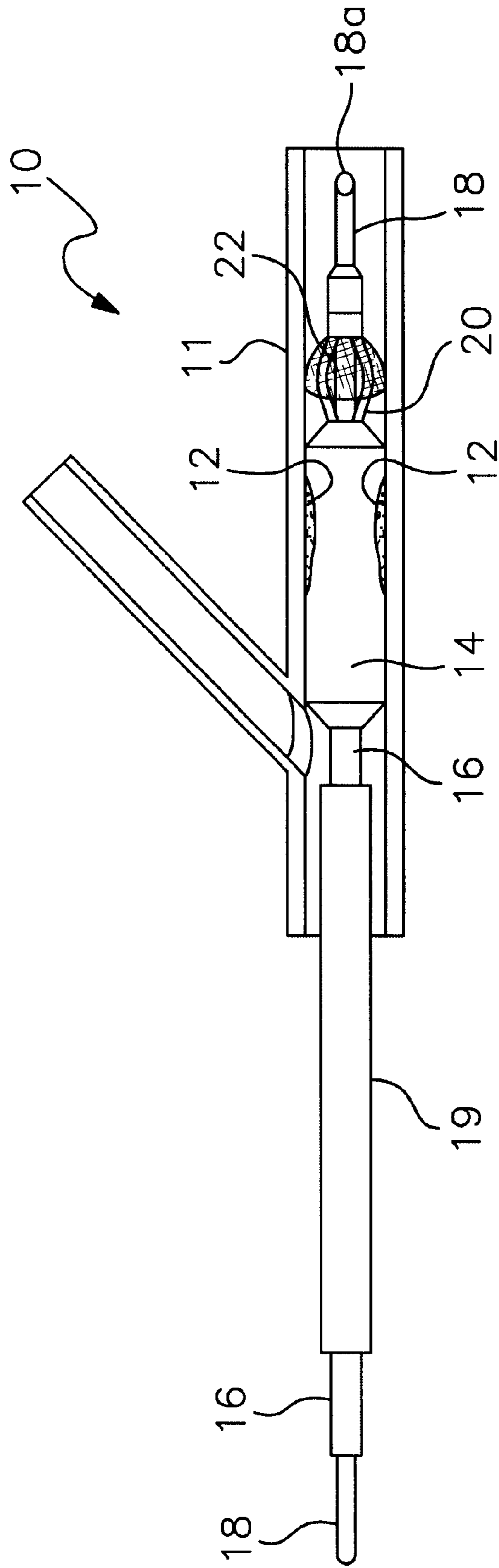
Fig. 1E
