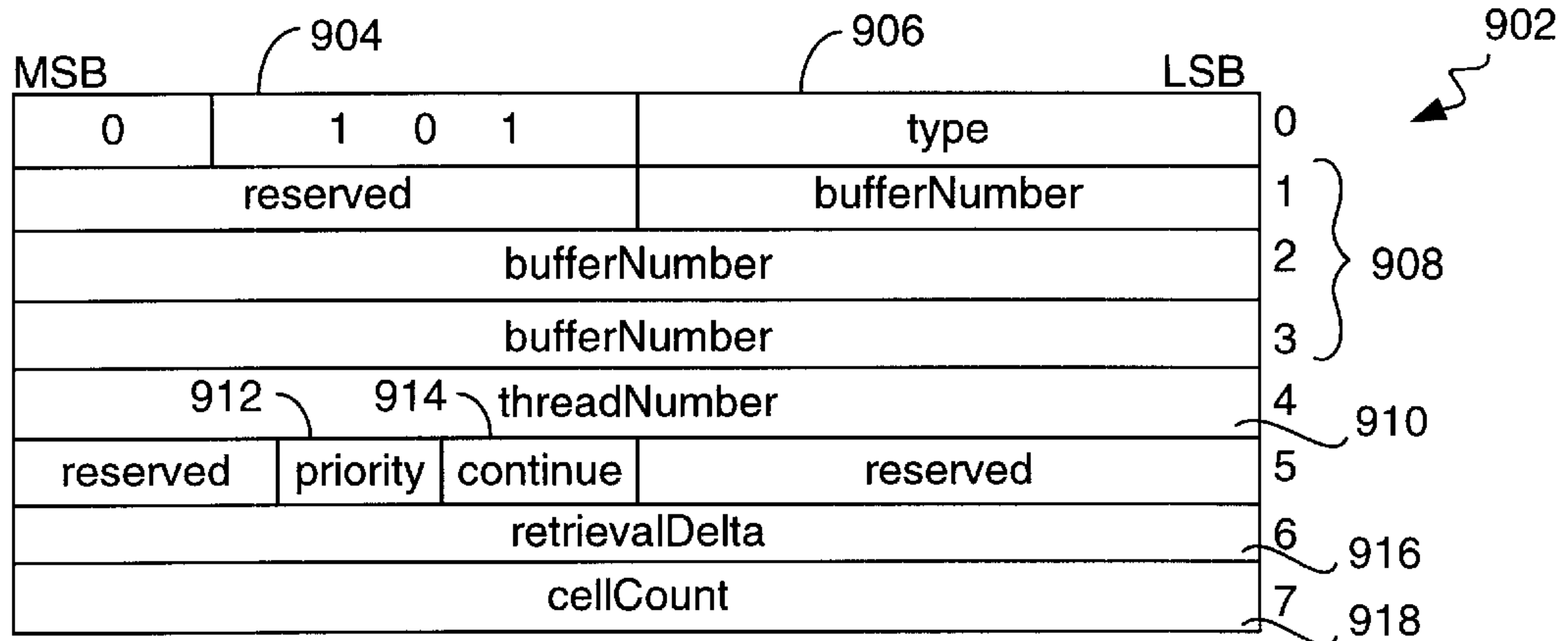
FrameRetrieval Molecule Format
