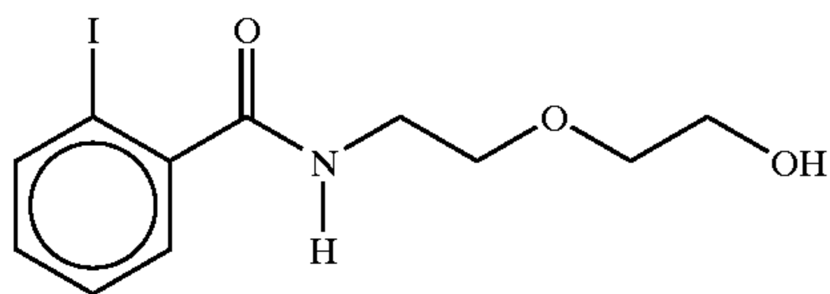
2-[N-(2-iodobenzoyl)aminoethoxy]ethanol
