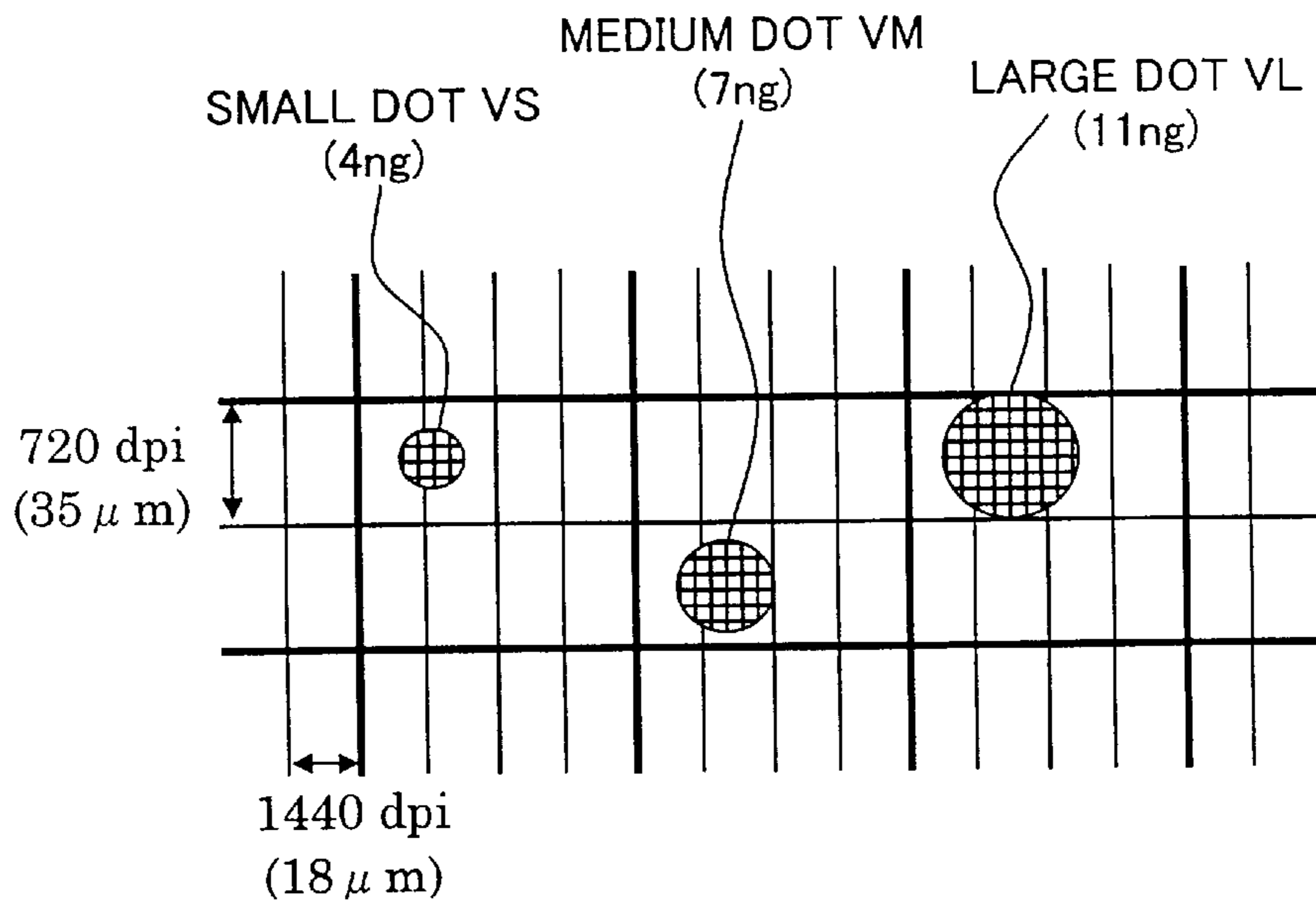
Fig. 11(B) VARIABLE DOTS
