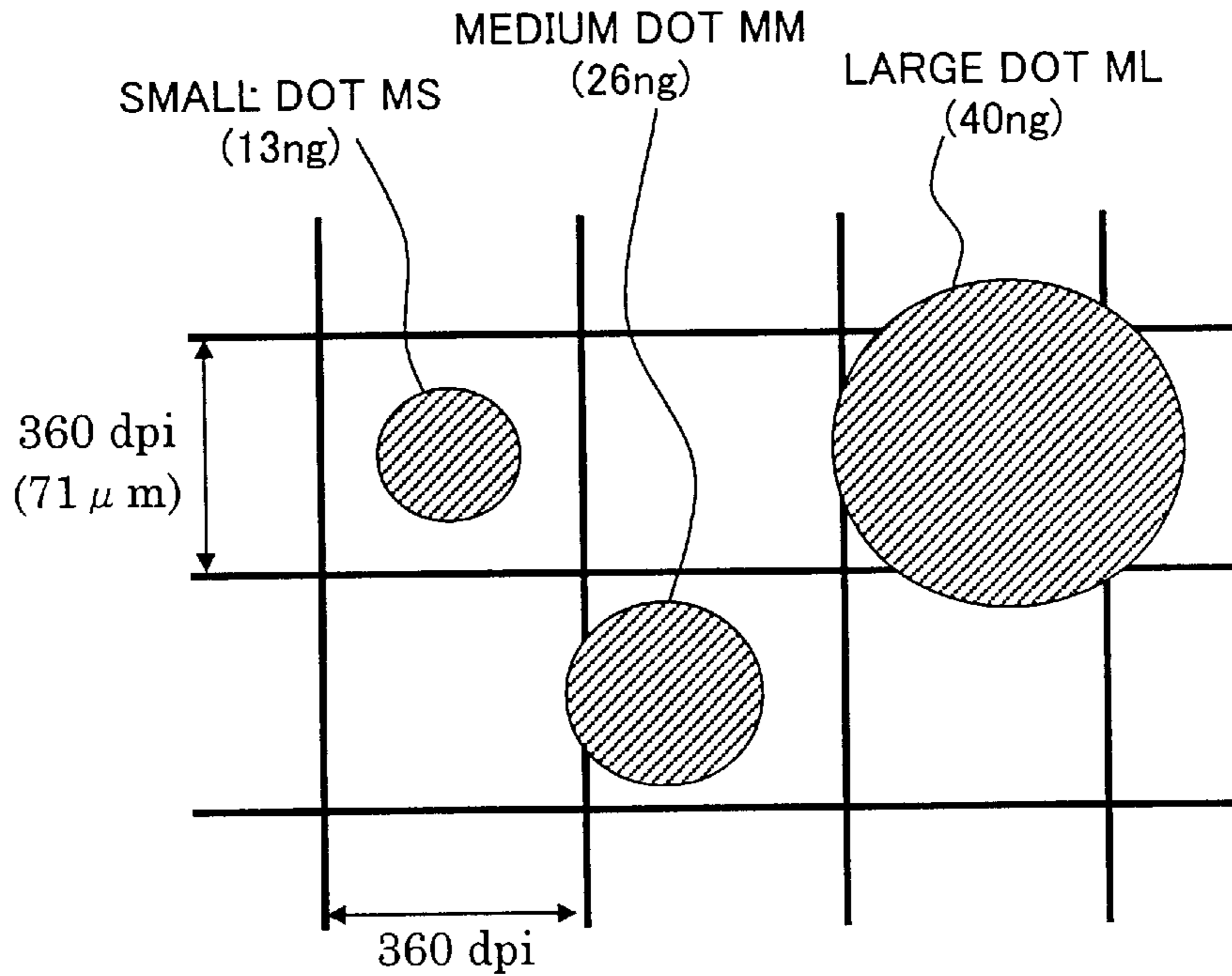
Fig. 11(B) VARIABLE DOTS
