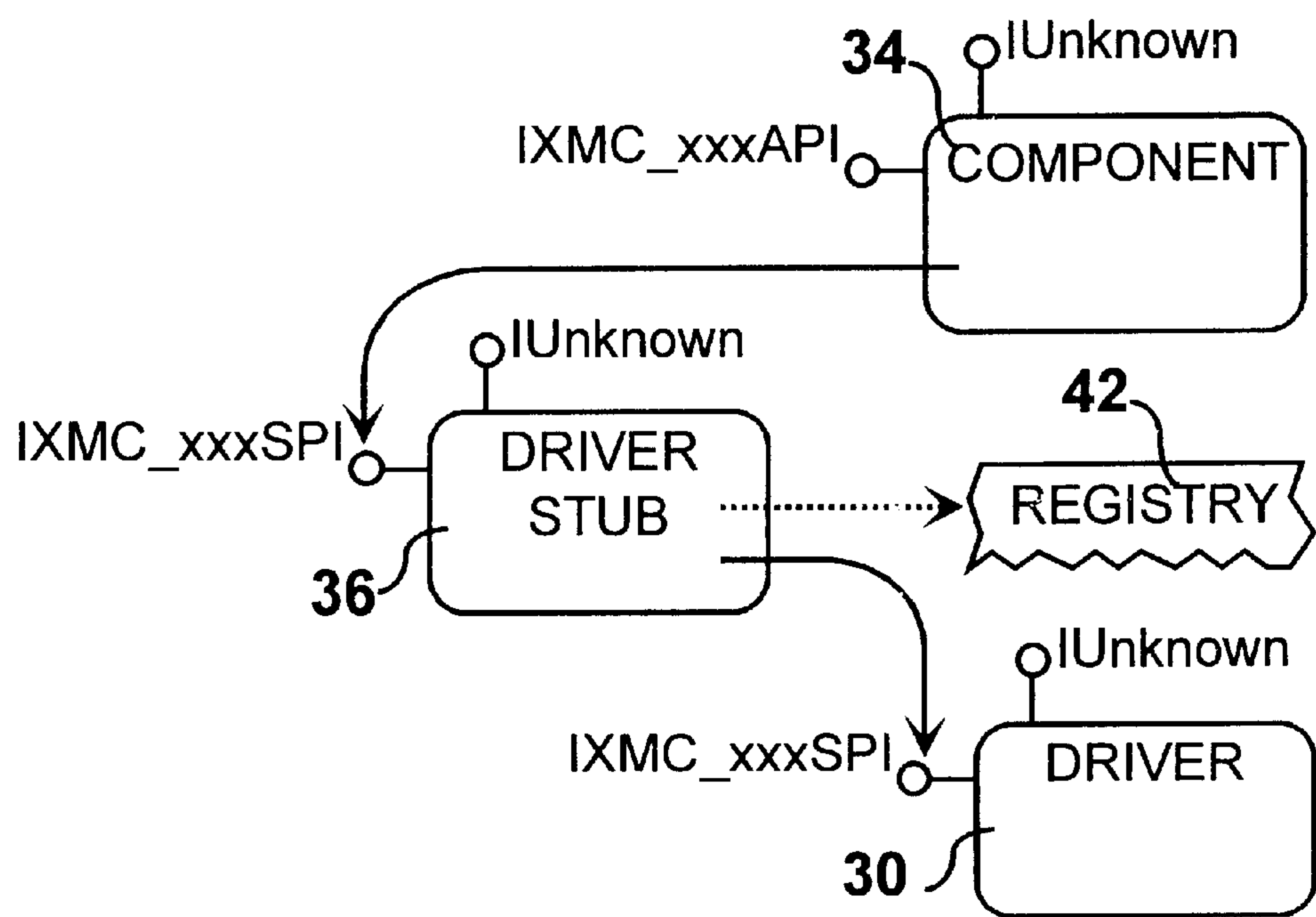
FIG. 34 Module Interaction-Map.
