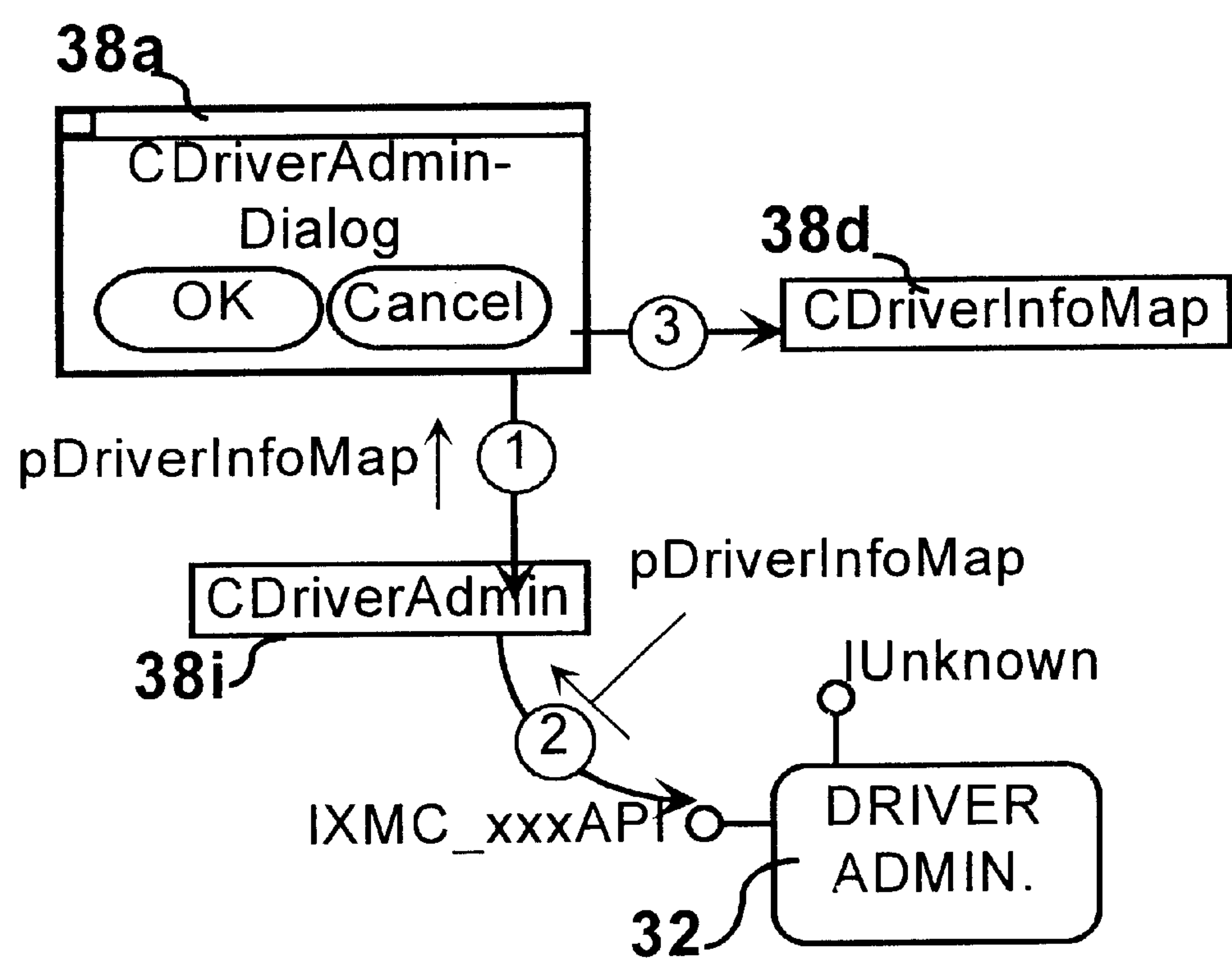
FIG. 54 Scenario-Map - Main Dialog Init.
