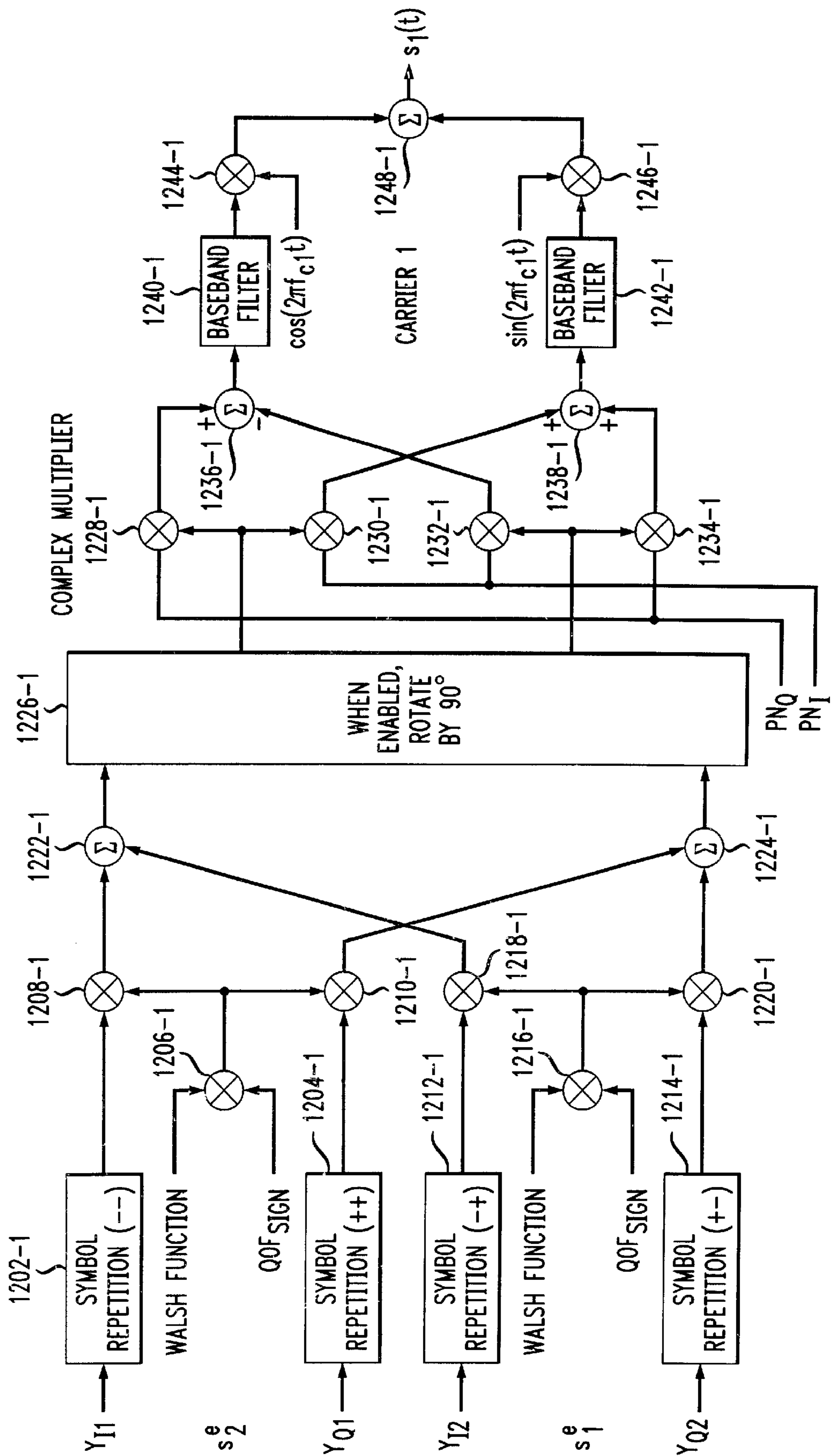
FIG. 12A P/O ANTENNA 2
