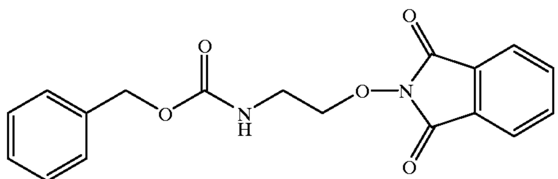
a. N-[2-(Benzyloxycarbonylamino)ethoxy]phthalimide
