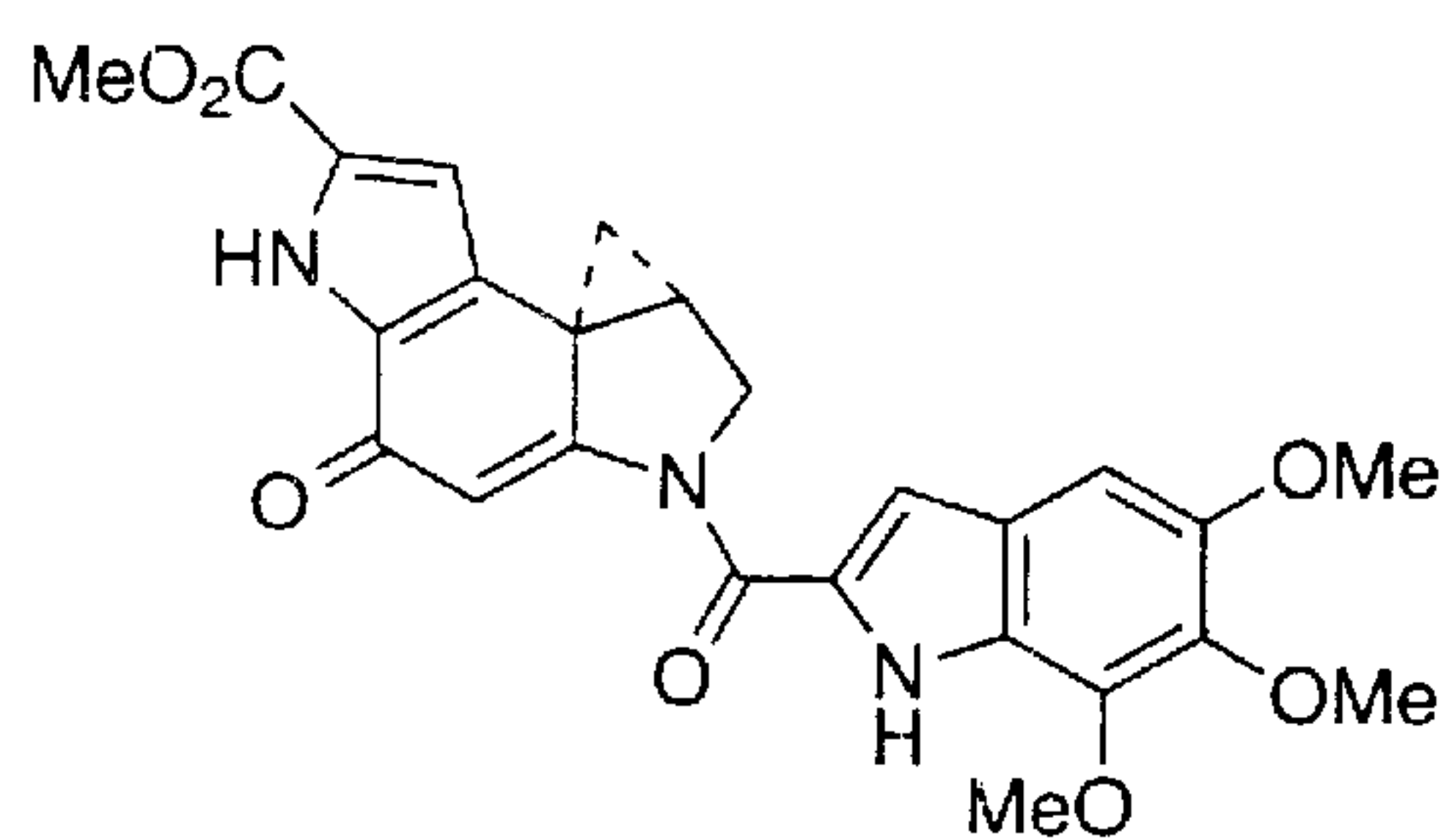
(+)- Duocarmycin SA
