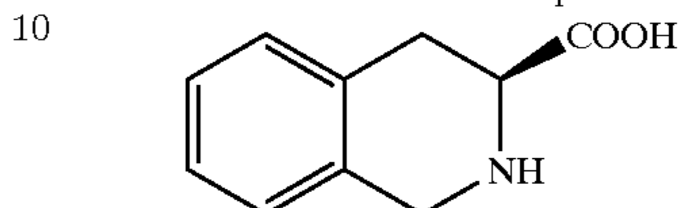
L-Tic
