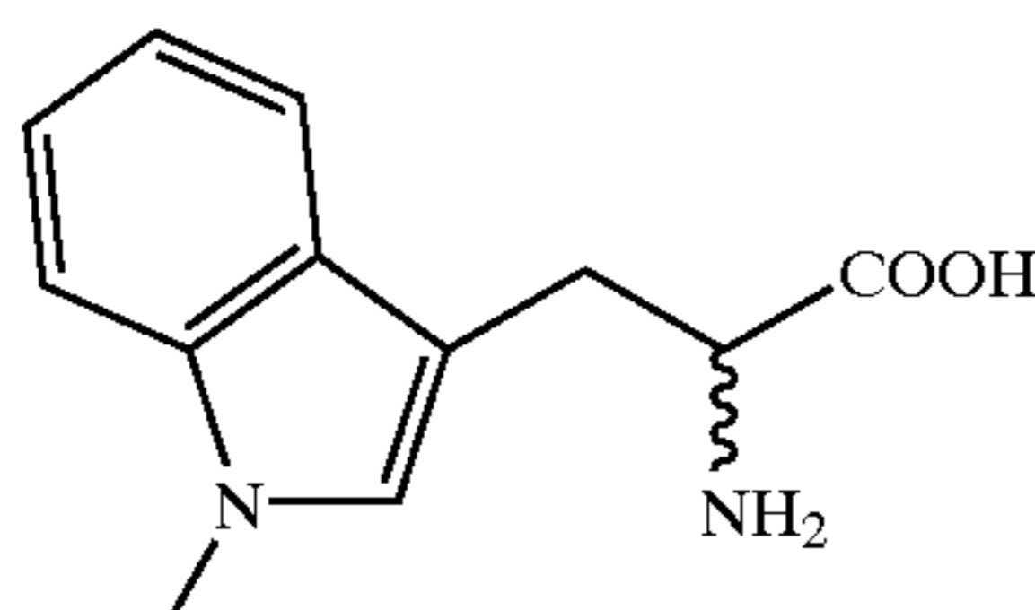
DL-1-Me-Trp
