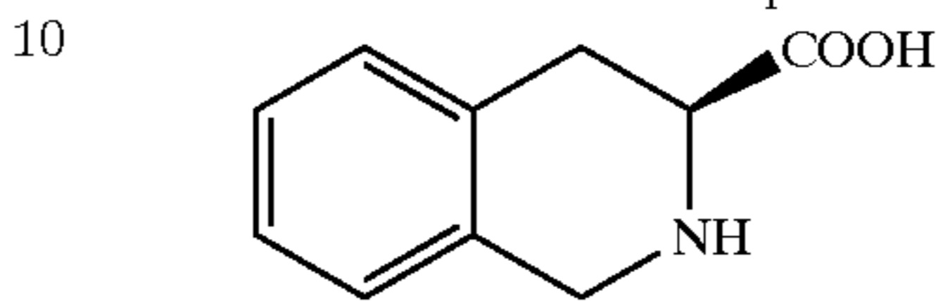
L-Tic
