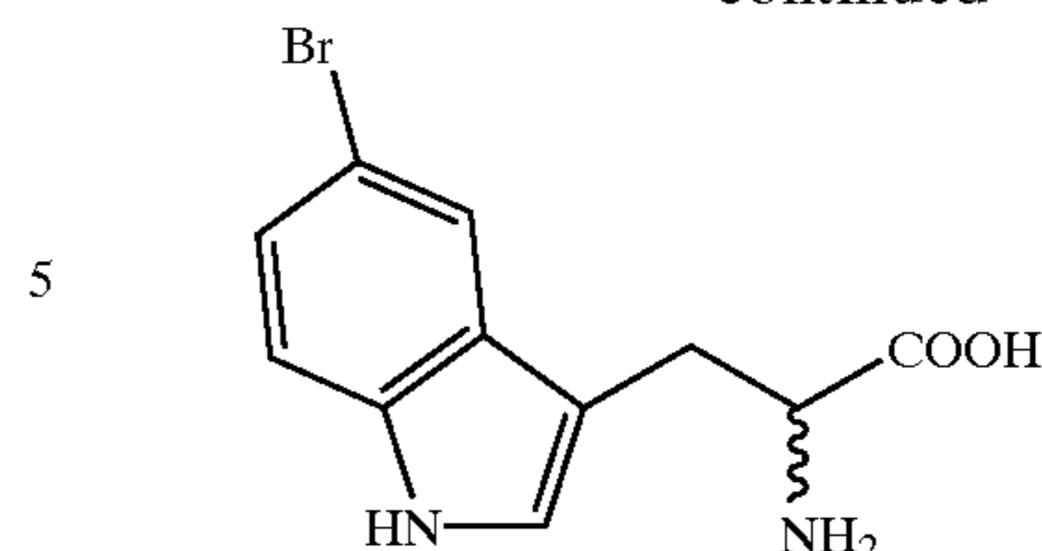
DL-5-Br-Trp
