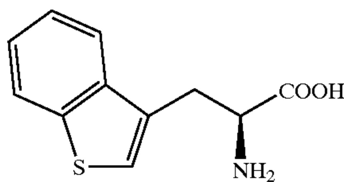
L-(Benzothieryl)-alanine
