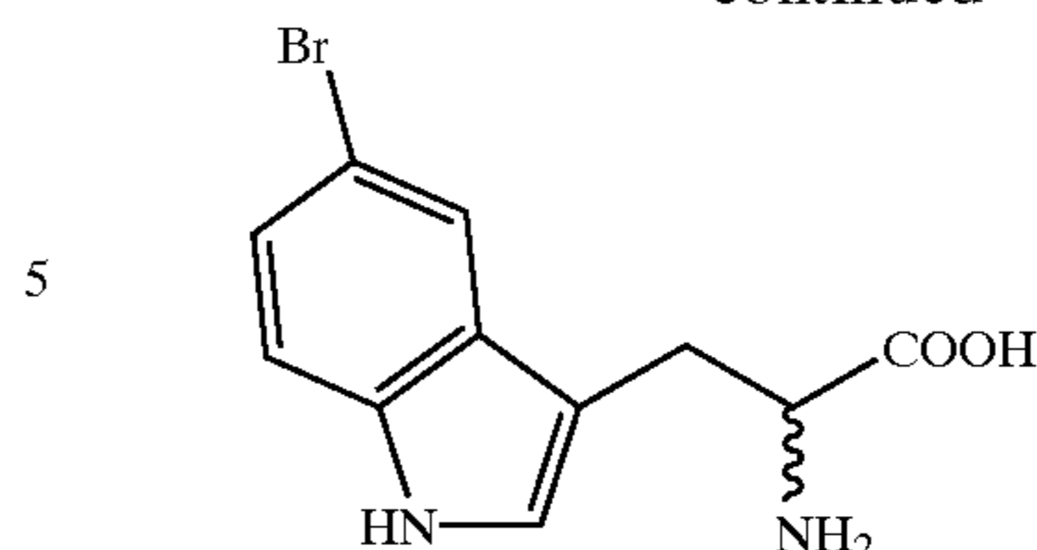
DL-5-Br-Trp
