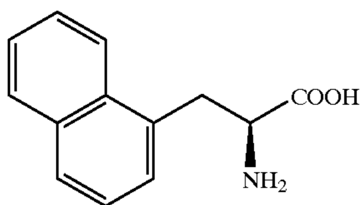
L-1-Nal
