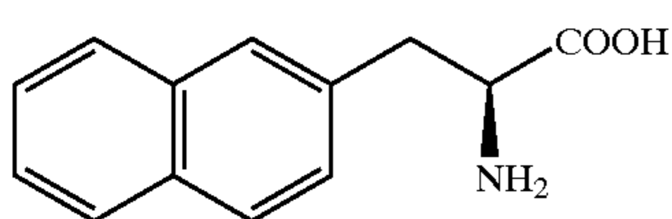
L-2-Nal
