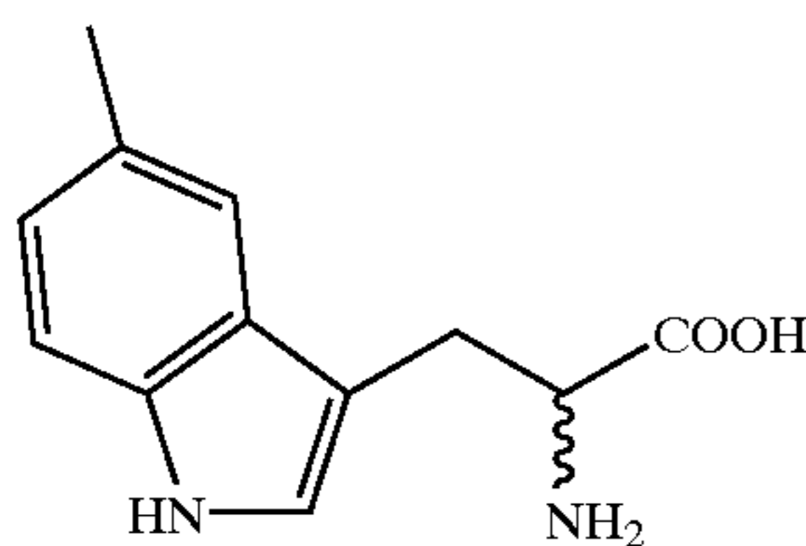
DL-5-Me-Trp
