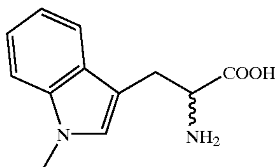
DL-1-Me-Trp
