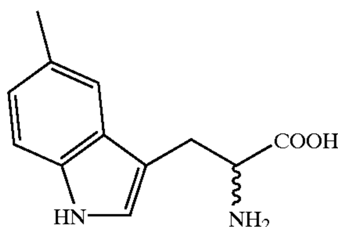
DL-5-Me-Trp
