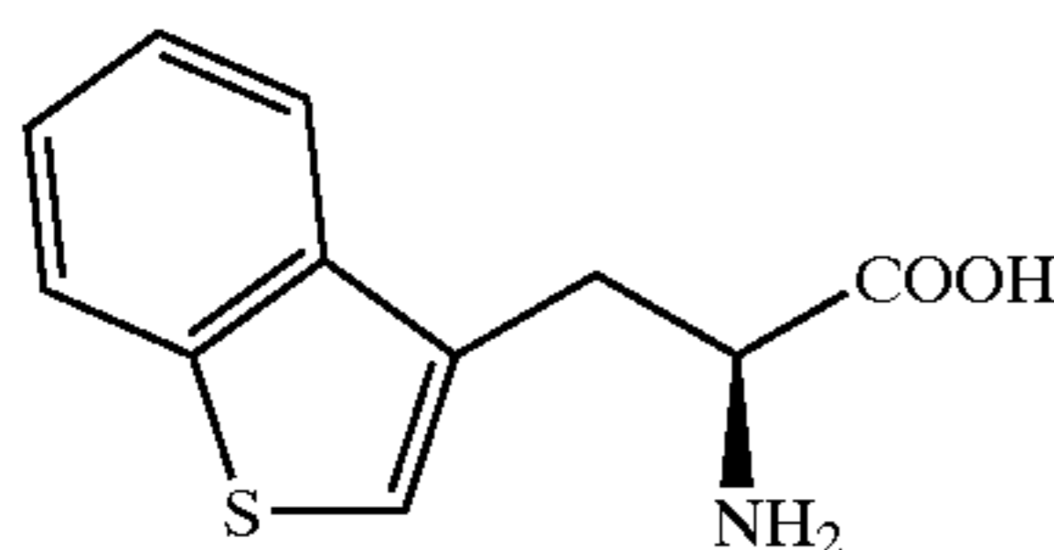
L-(Benzothieryl)-alanine
