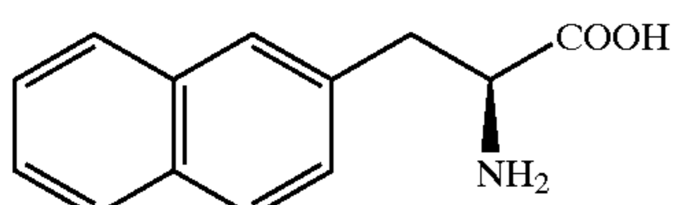
L-2-Nal
