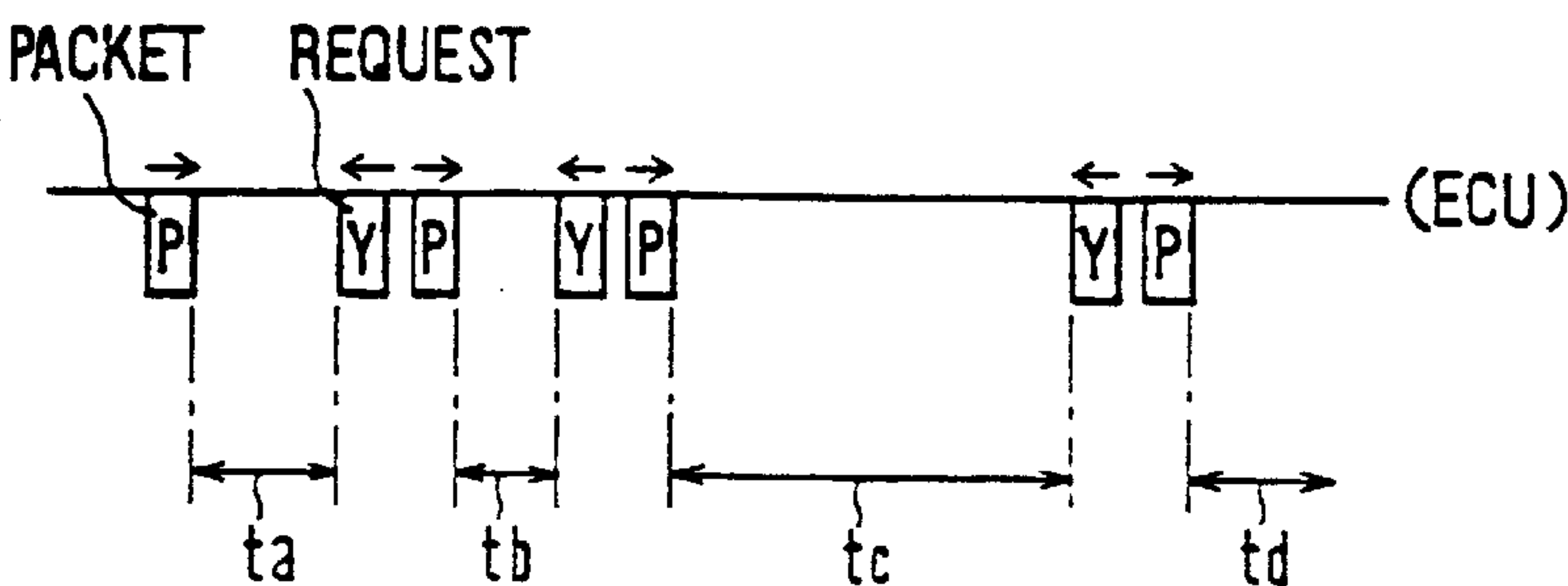
FIG. 15A
