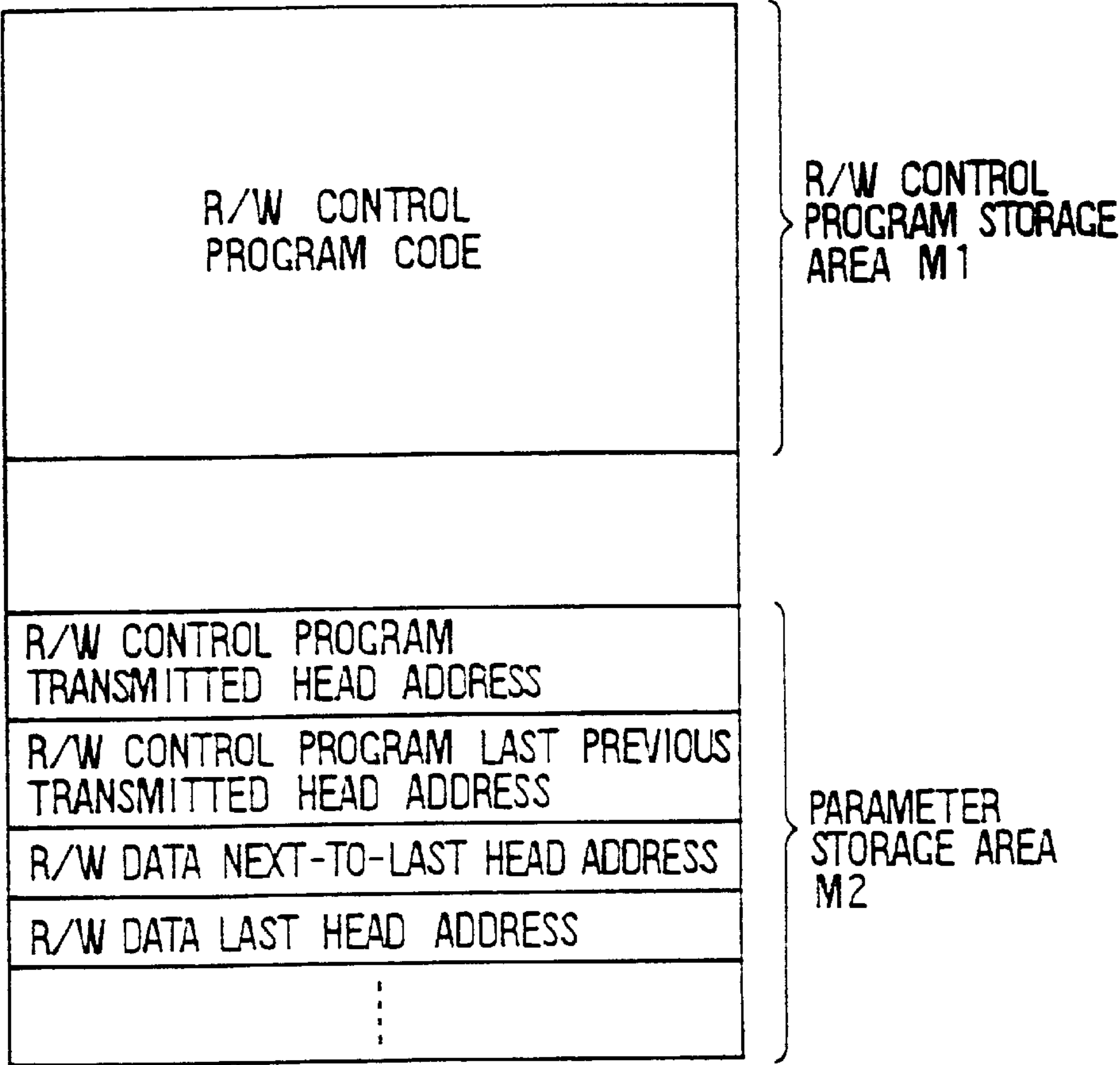
FIG. 2
