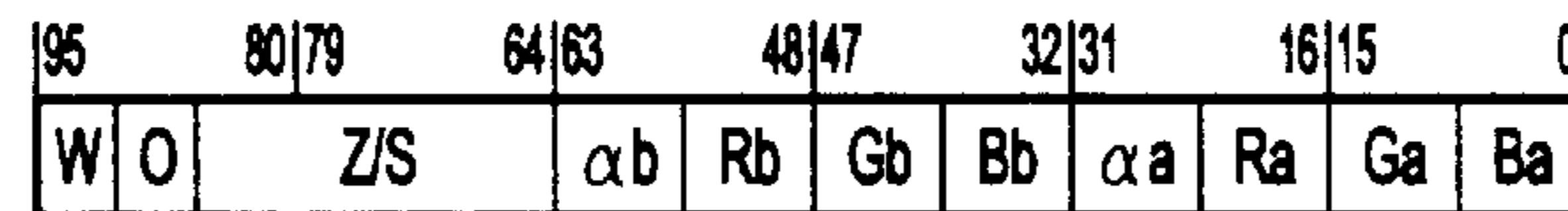
96 bpp Pixel Format 4:4:24:2*(8:8:8:8)
