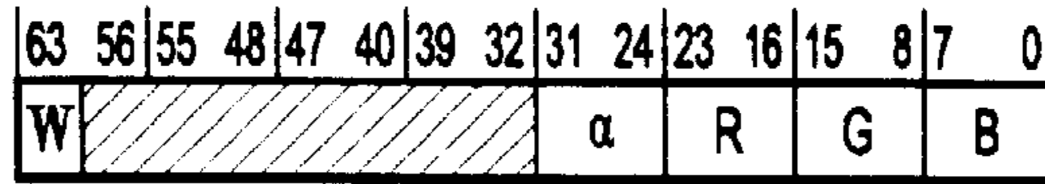
64 BPP PIXEL FORMAT 4:8:8:8
