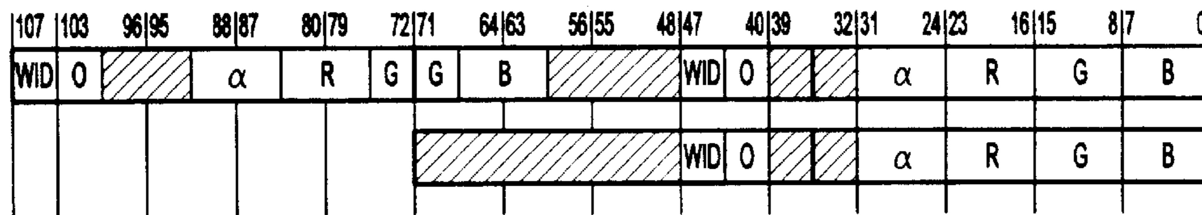
96 bpp Display Refresh 4:4:24:2*(8:8:8:8)
