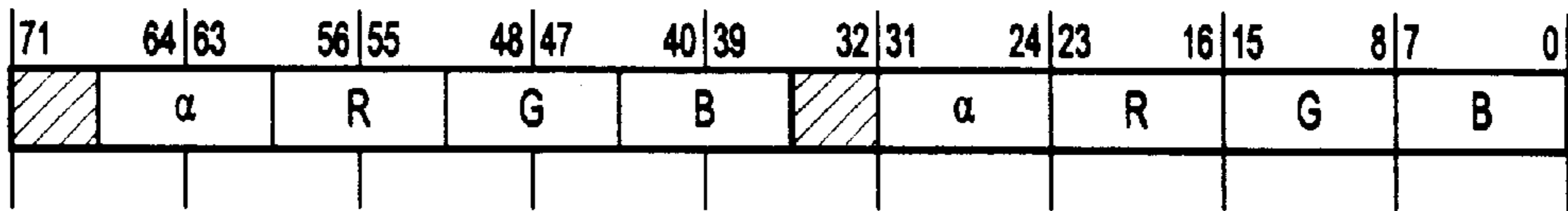
32 BPP DISPLAY REFRESH 8:8:8:8
