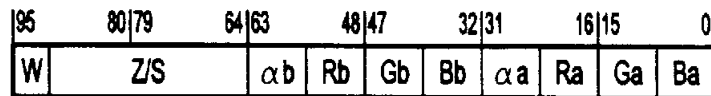
96 bpp Pixel Format 4:28:2*(8:8:8:8)
