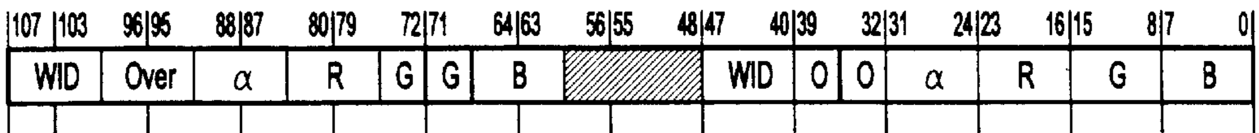
128 bpp Display Refresh 8:32:8:2*(8:8:8:8)
